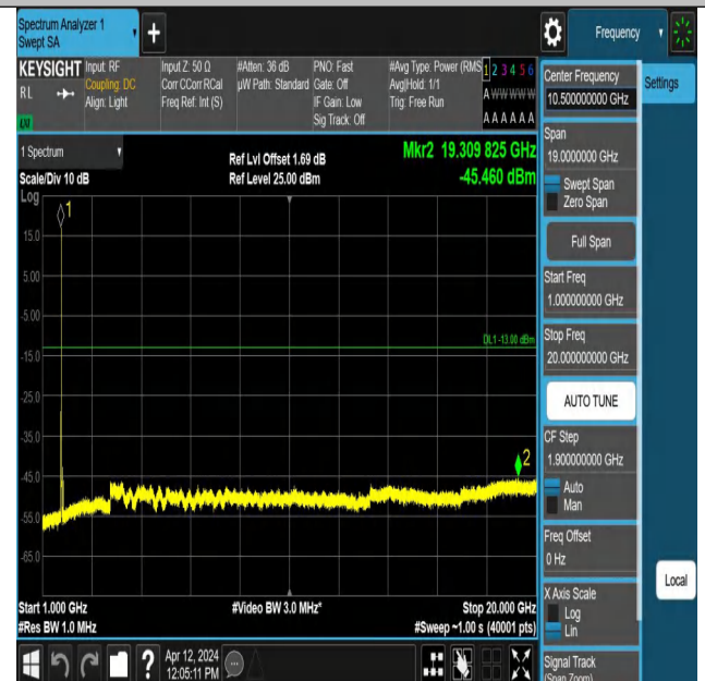
Band4-1312-1-1000~20000MHz-PASS
