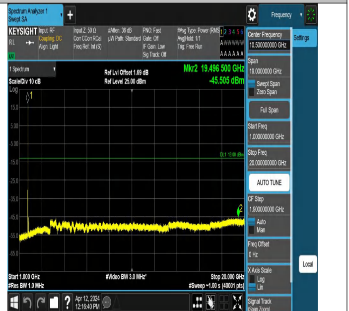
Band4-1312-5-1000~20000MHz-PASS
