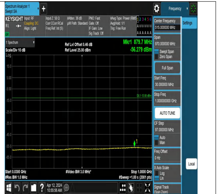
Band4-1513-2-30~1000MHz-PASS
