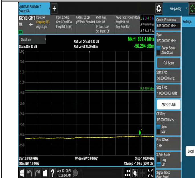
Band4-1513-3-30~1000MHz-PASS
