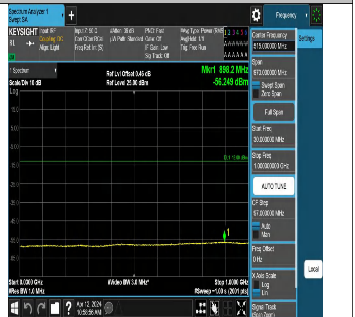
Band4-1312-4-30~1000MHz-PASS
