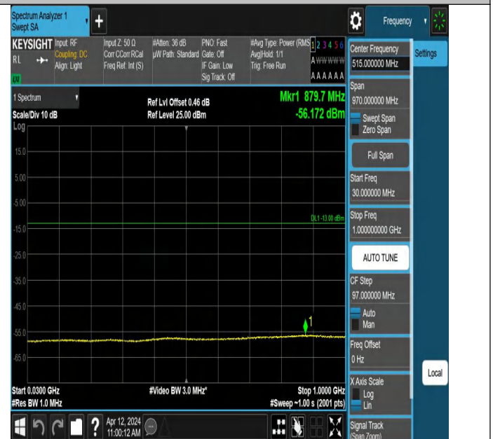
Band4-1513-4-30~1000MHz-PASS
