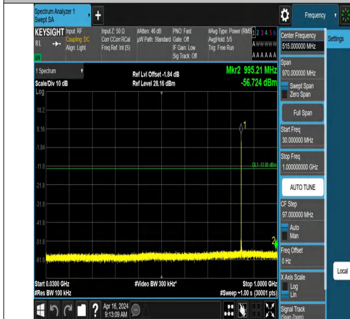
EGPRS850-251-8-30~1000MHz-PASS
