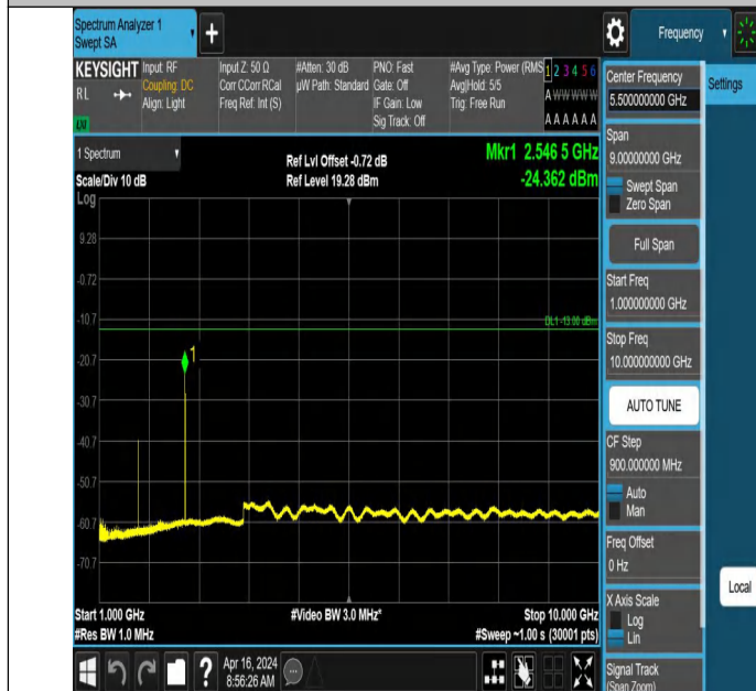
GSM850-251-5-1000~10000MHz-PASS
