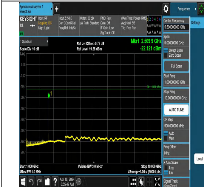
GSM850-190-5-1000~10000MHz-PASS
