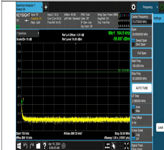
GSM850-251-5-0.15~30MHz-PASS
