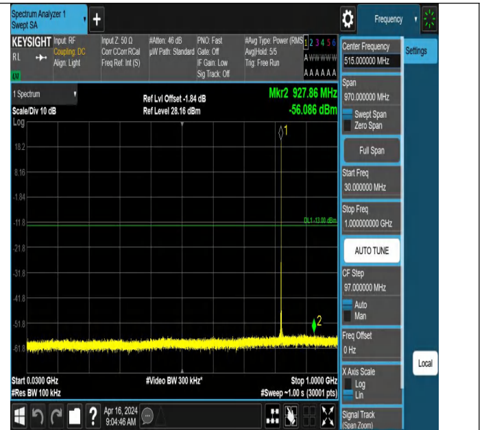
GPRS850-128-5-30~1000MHz-PASS
