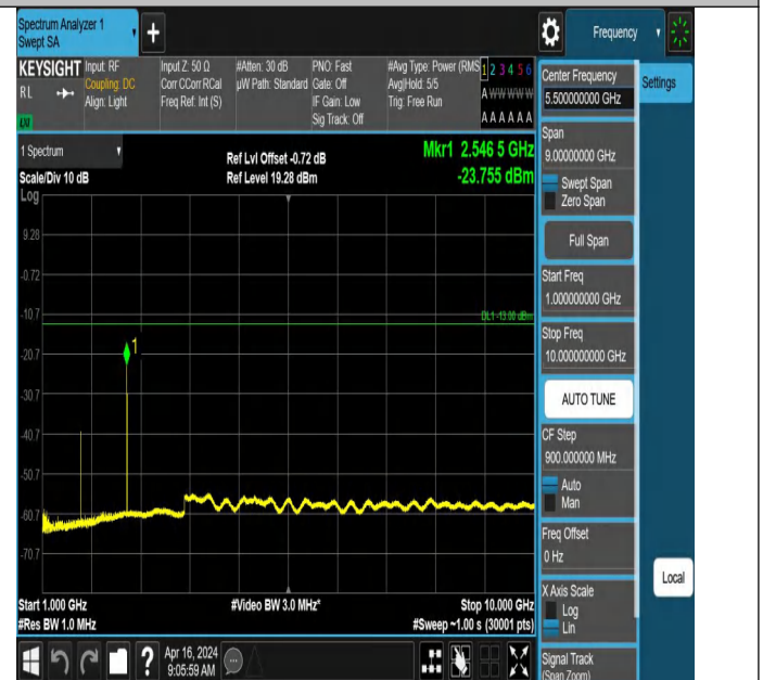
GPRS850-251-5-1000~10000MHz-PASS
