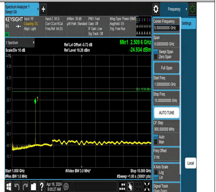
GPRS850-190-5-1000~10000MHz-PASS
