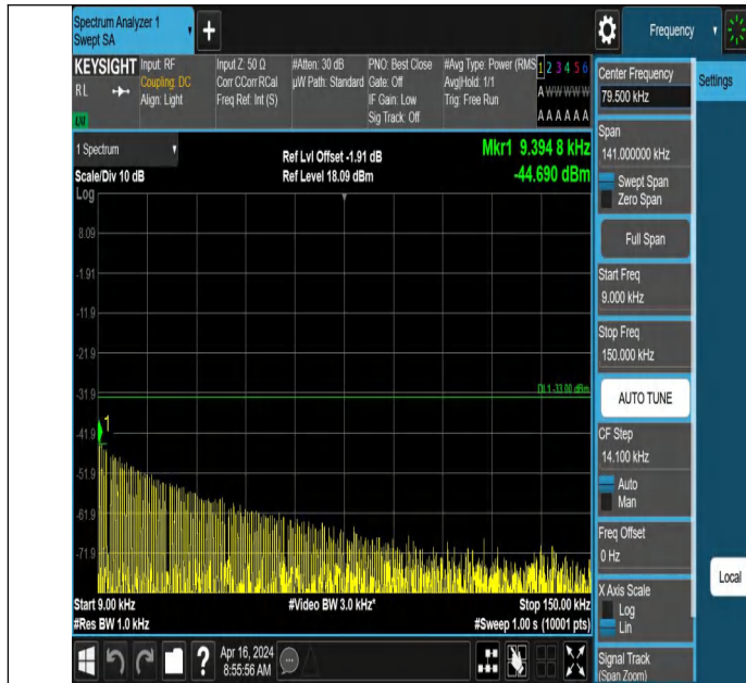
GSM850-251-5-0.009~0.15MHz-PASS
