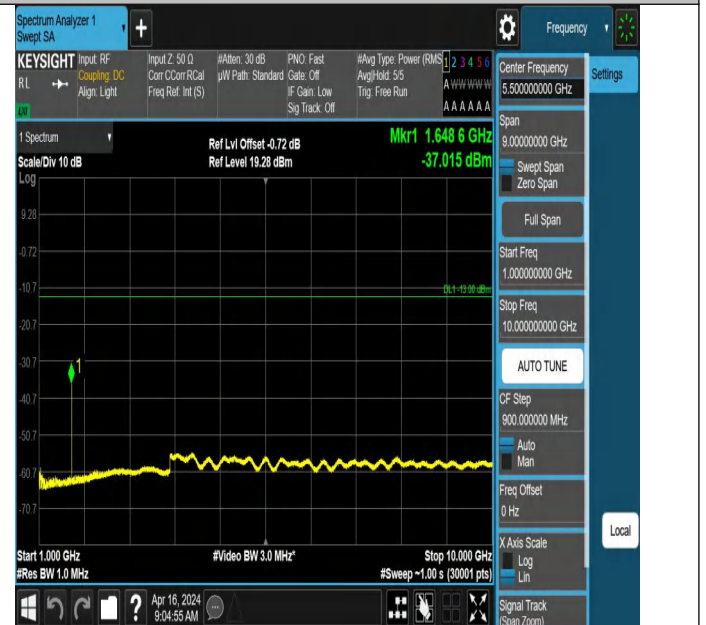
GPRS850-128-5-1000~10000MHz-PASS
