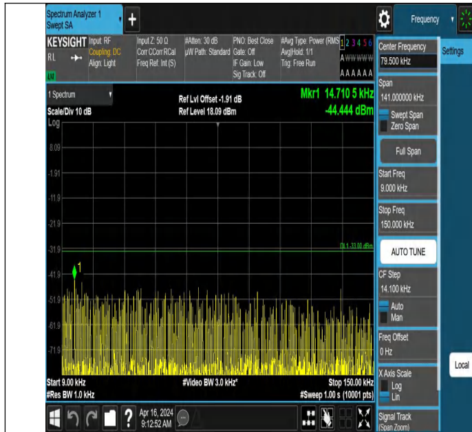
EGPRS850-251-8-0.009~0.15MHz-PASS
