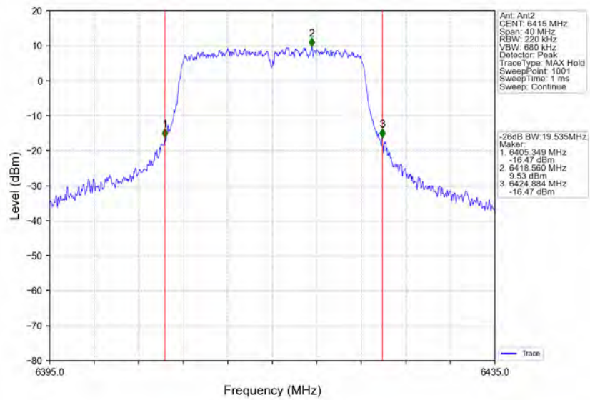
802.11a_HCH_6415MHz_Ant2_NTNV
