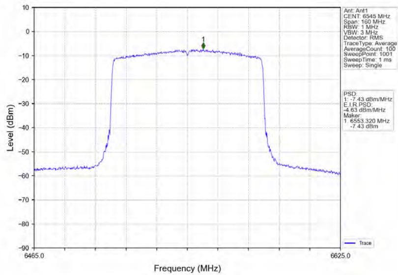
802.11ax(HEW80)_HCH_6545MHz_RU996_Left_Ant1_NTNV
