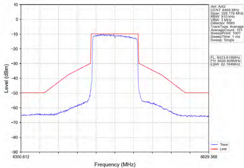
802.11ax(HEW80)_LCH_6465MHz_RU996_Left_Ant2_NTNV
