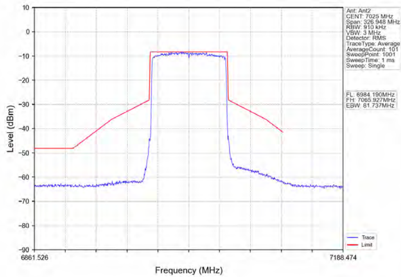
802.11ax(HEW80)_HCH_7025MHz_RU996_Left_Ant2_NTNV
