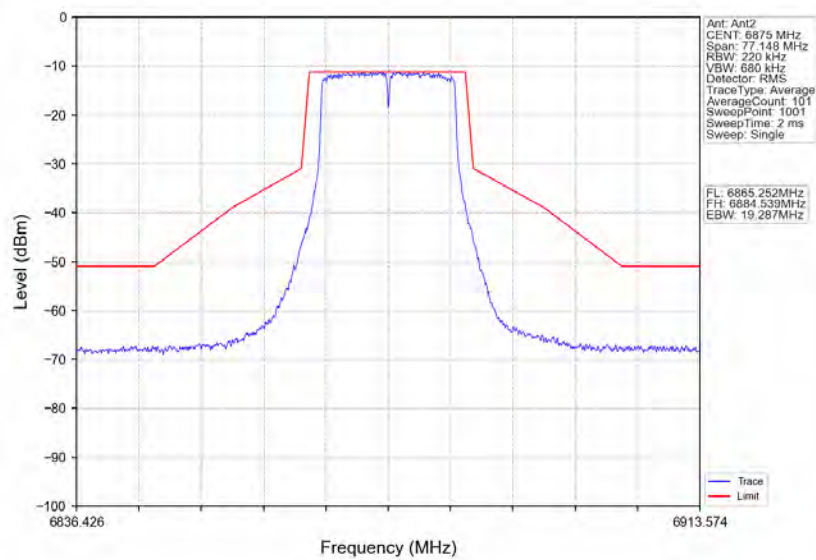
802.11a HCH 6875MHz Ant2 NTN
