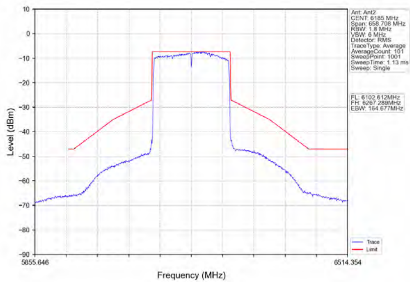
802.11ax(HEW160)_MCH_6185MHz_2xRU996_Left_Ant2_NTNV
