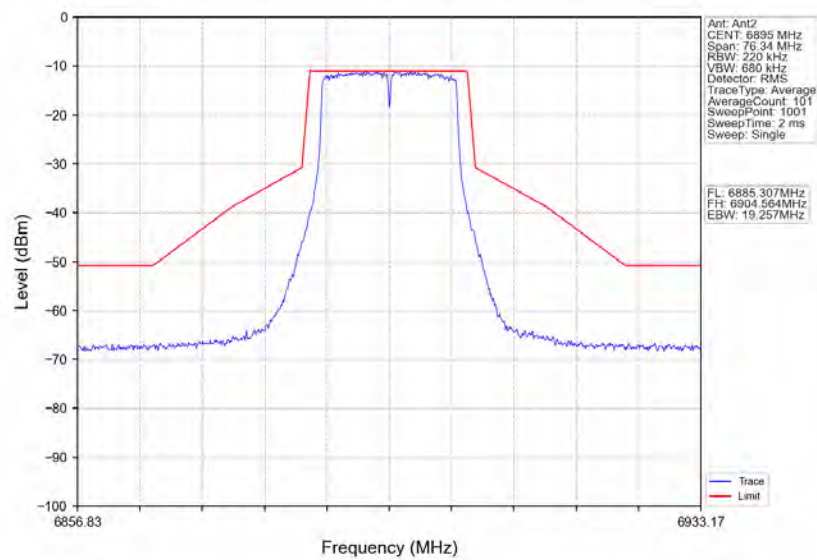
802.11a LCH 6895MHz Ant2 NTN
