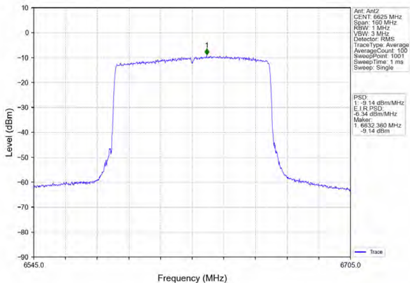
802.11ax(HEW80)_LCH_6625MHz_RU996_Left_Ant2_NTNV
