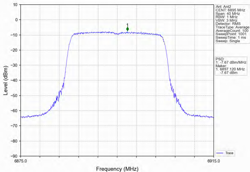
802.11ax(HEW20)_LCH_6895MHz_RU242_Left_Ant2_NTNV
