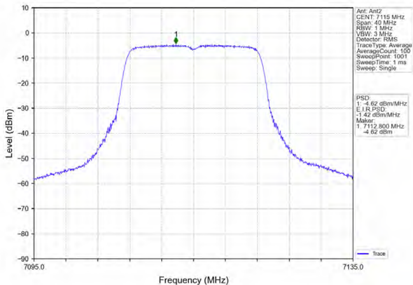
802.11a_HCH_7115MHz_Ant2_NTNV
