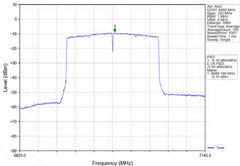
802.11ax(HEW160)_MCH_6985MHz_2xRU996_Left_Ant2_NTNV
