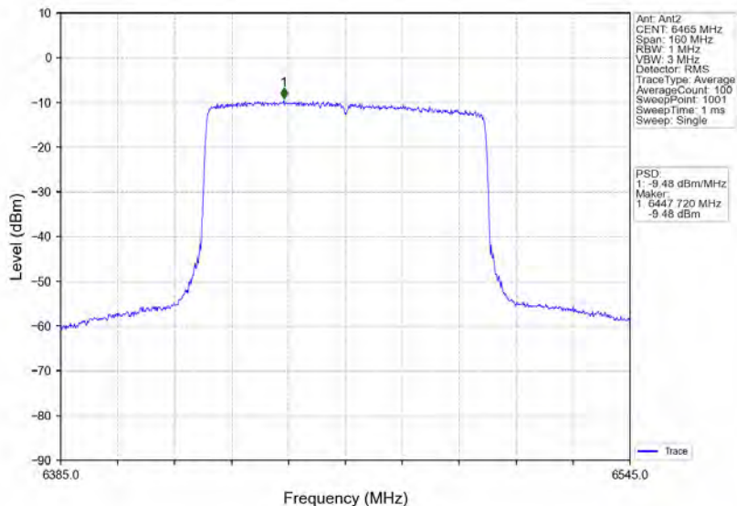
802.11ax(HEW80)_LCH_6465MHz_RU996_Left_MIMO_NTNV
