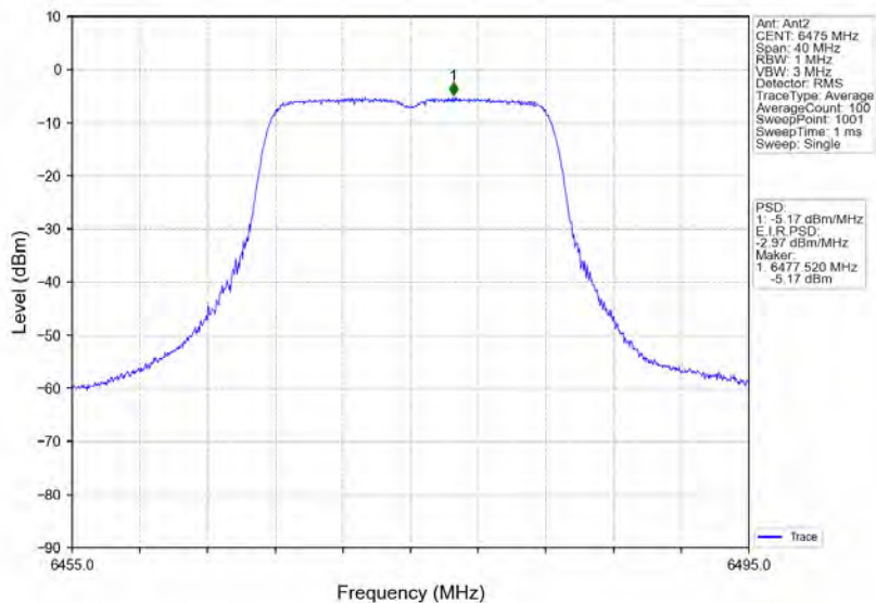
802.11a_MCH_6475MHz_Ant2_NTNV
