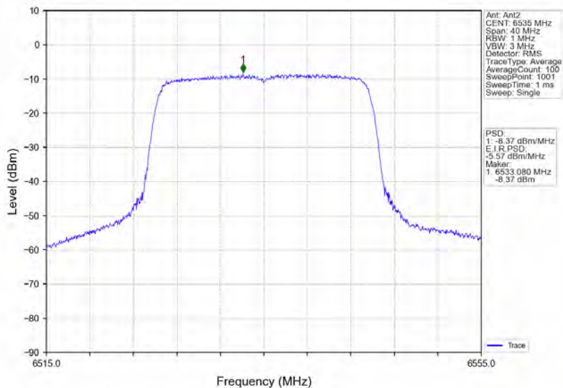
802.11ax(HEW20)_LCH_6535MHz_RU242_Left_Ant2_NTNV
