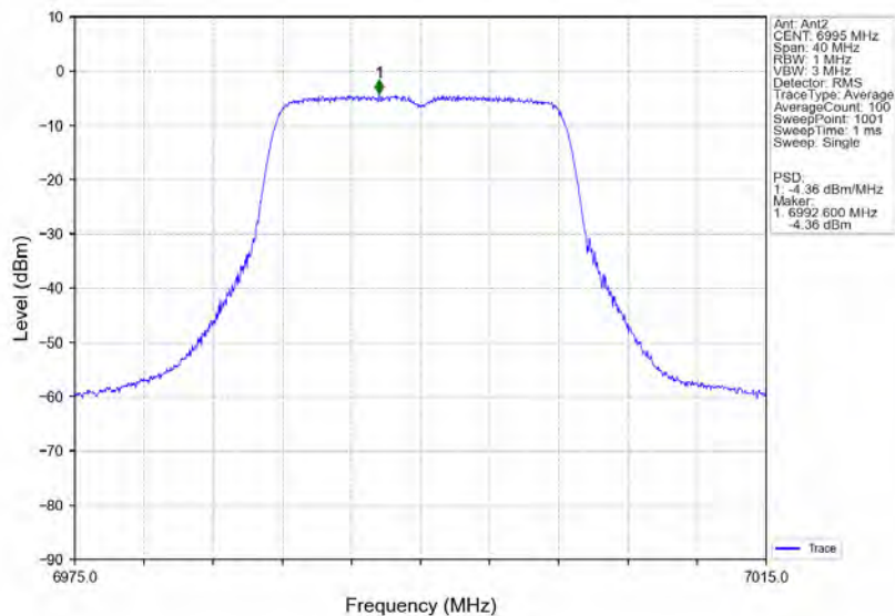
802.11a_MCH_6995MHz_Ant2_NTNV
