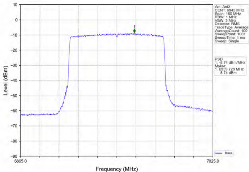
802.11ax(HEW80)_LCH_6945MHz_RU996_Left_Ant2_NTNV
