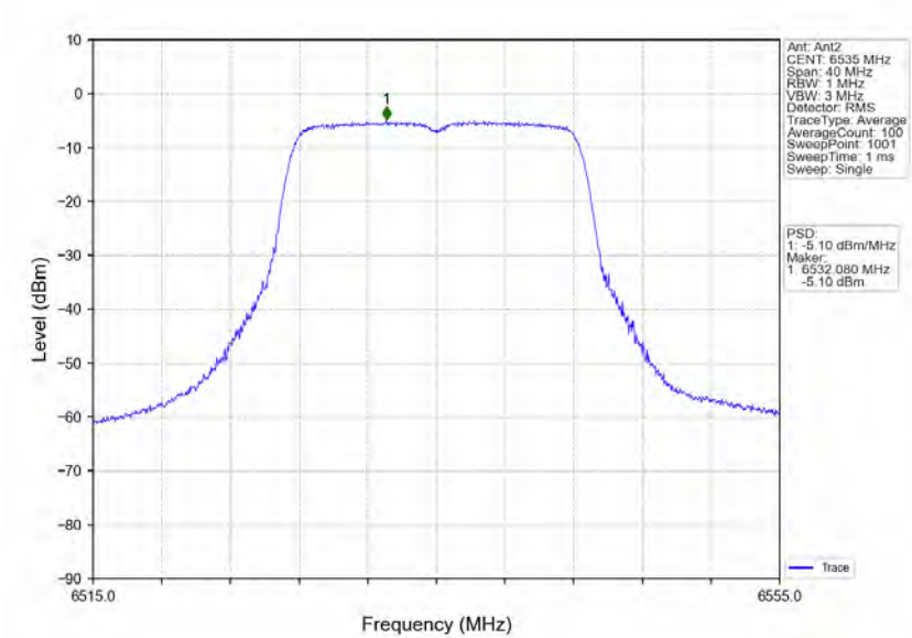
802.11a_LCH_6535MHz_Ant2_NTNV
