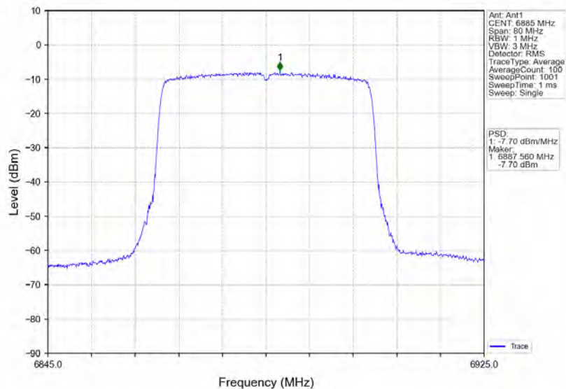
802.11ax(HEW40)_HCH_6885MHz_RU484_Left_Ant1_NTNV
