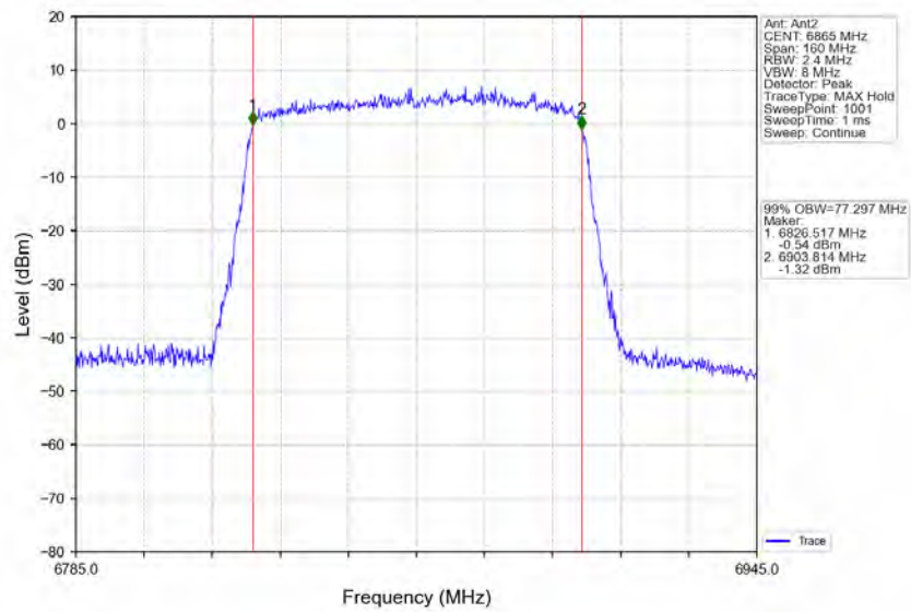
802.11ax(HEW80)_HCH_6865MHz_RU996_Left_Ant2_NTNV
