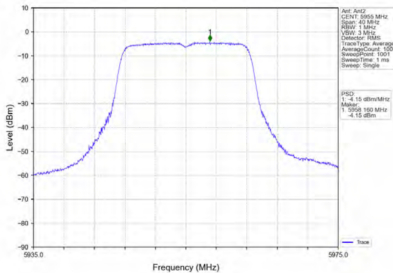
802.11a_LCH_5955MHz_Ant2_NTNV
