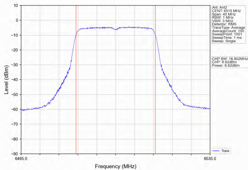
802.11a_HCH_6515MHz_Ant2_NTNV
