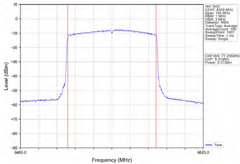
802.11ax(HEW80)_HCH_6545MHz_RU996_Left_Ant2_NTNV
