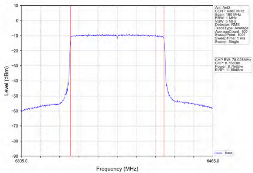
802.11ax(HEW80)_HCH_6385MHz_RU996_Left_Ant2_NTNV
