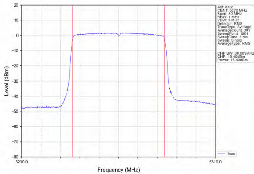
802.11ax(HEW40)_LCH_5270MHz_RU484_Left_Ant2_NTNV
