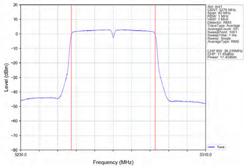
802.11n(HT40)_LCH_5270MHz_Ant2_NTNV
