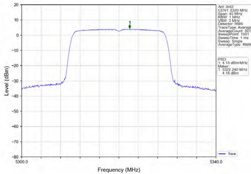
802.11ax(HEW20)_HCH_5320MHz_RU242_Left_Ant2_NTNV
