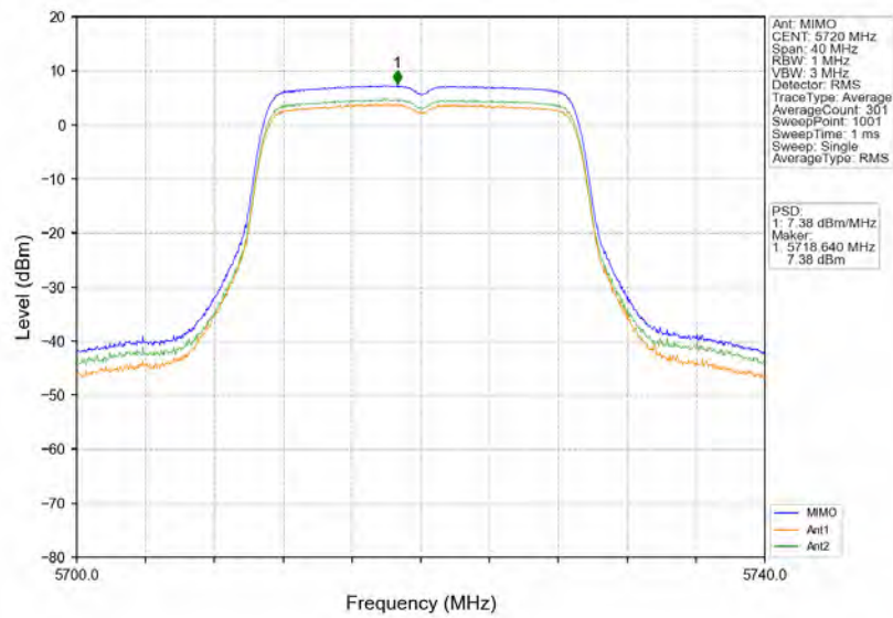
802.11n(HT20)_HCH_5720MHz_MIMO_NTNV
