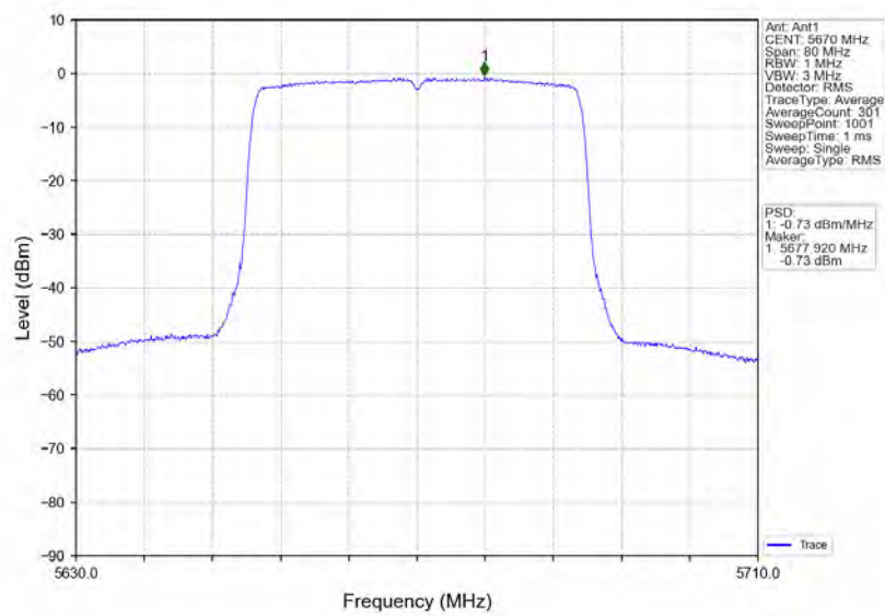
802.11ax(HEW40)_HCH_5670MHz_RU484_Left_Ant1_NTNV
