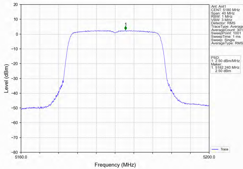
802.11ax(HEW20)_LCH_5180MHz_RU242_Left_Ant1_NTNV
