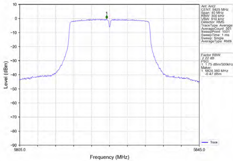
802.11n(HT20)_HCH_5825MHz_Ant2_NTNV
