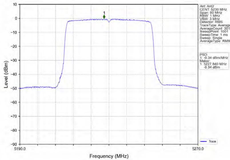
802.11ax(HEW40)_HCH_5230MHz_RU484_Left_Ant2_NTNV
