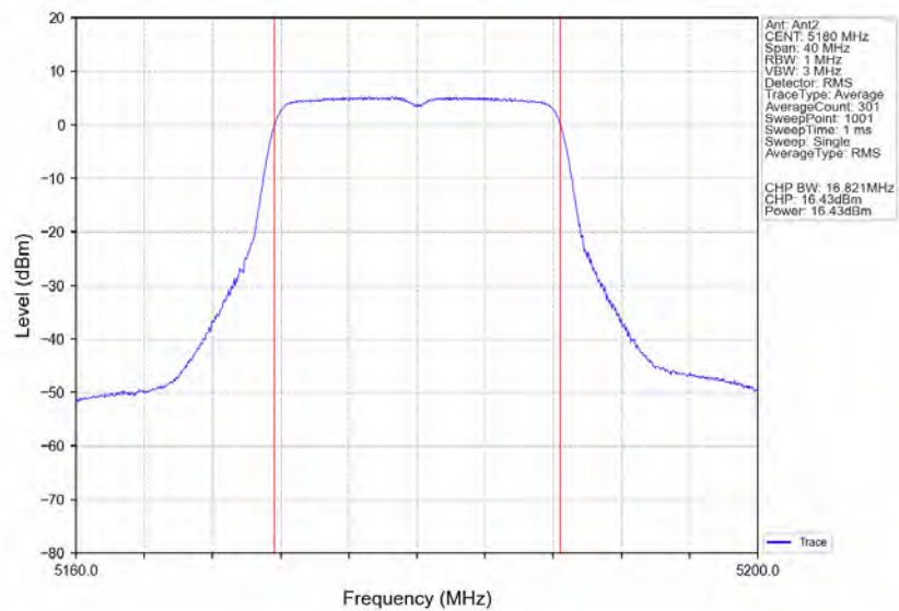
802.11a LCH 5180MHz Ant2 NTNV
