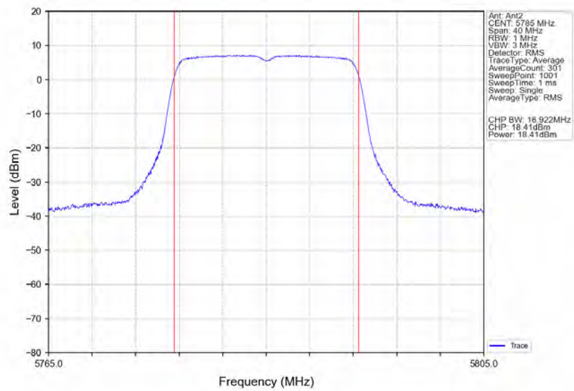
802.11a_MCH_5785MHz_Ant2_NTNV
