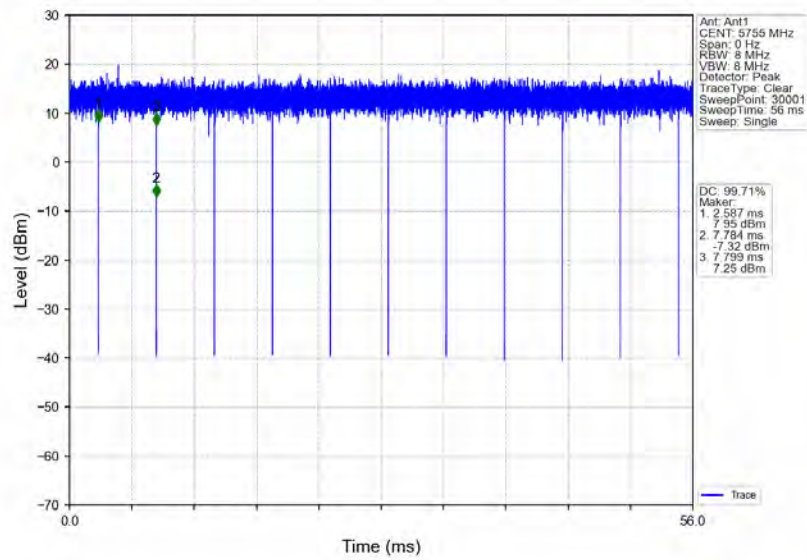
802.11n(HT40)_LCH_5755MHz_Ant1_NTNV
