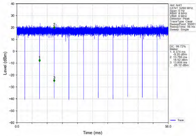
802.11ax(HEW20)_LCH_5260MHz_RU242_Left_Ant1_NTNV
