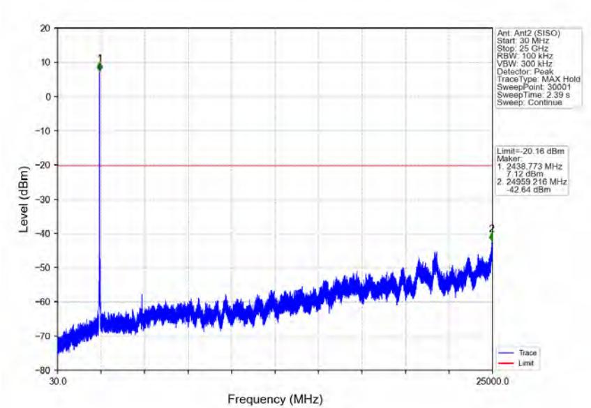
802.11b MCH 2437MHz Ant2 (SISO) NTNV
