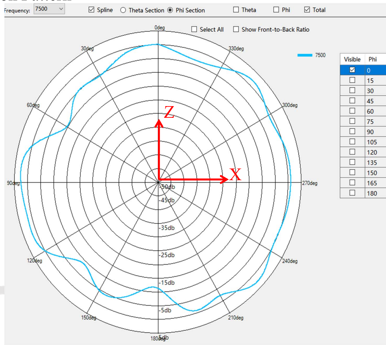
7500MHz XZ plot
