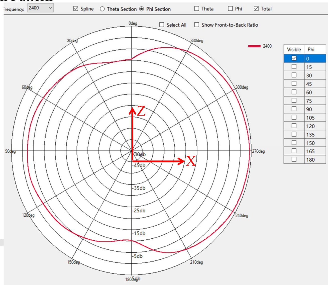
2400MHz XZ plot
