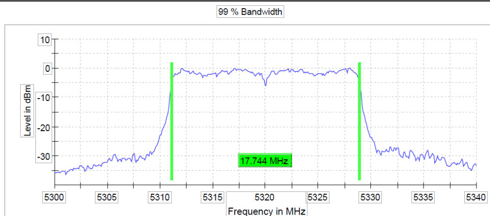
11N20_Ant1_5320
