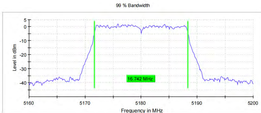
11A_Ant0_5180
