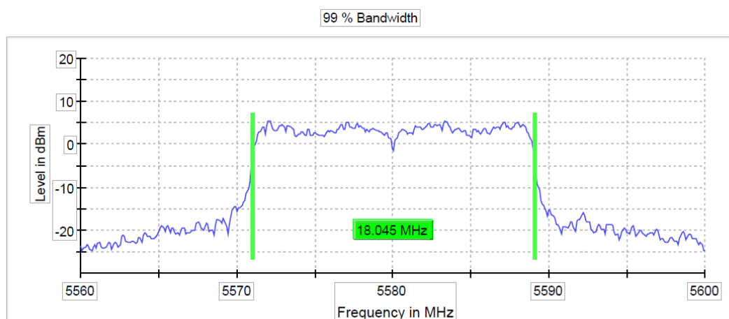
11N20_Ant0_5580
