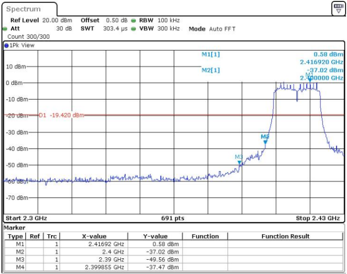
11N20_Ant1_Low_2412
