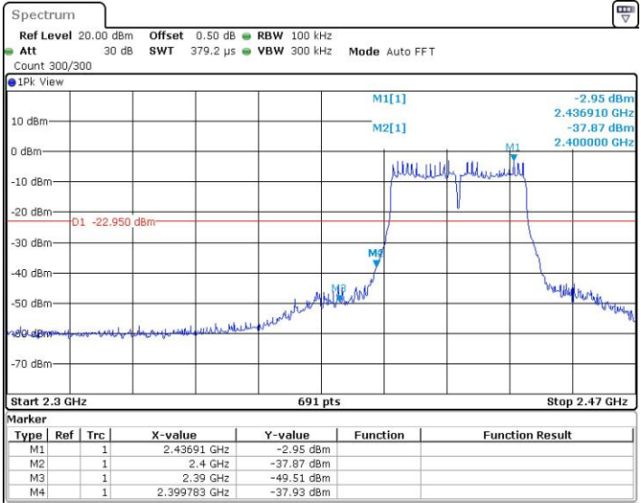
11N40_Ant2_Low_2422
