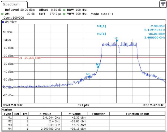
11N40_Ant1_Low_2422
