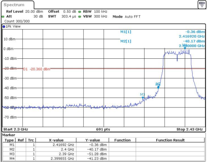
11N20_Ant2_Low_2412
