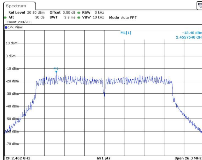
11N20_Ant2_2462
