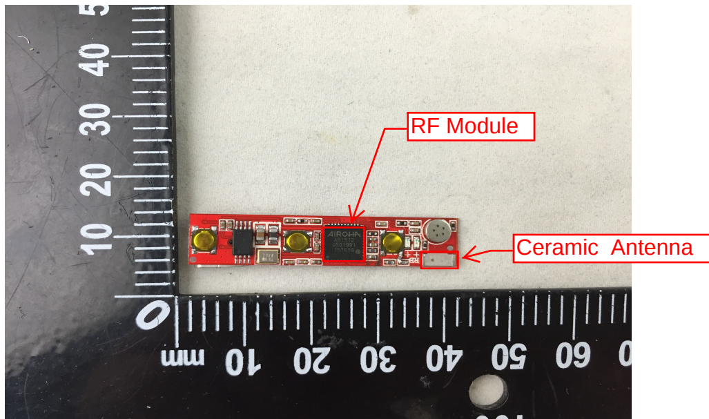
EUT Photo 4
