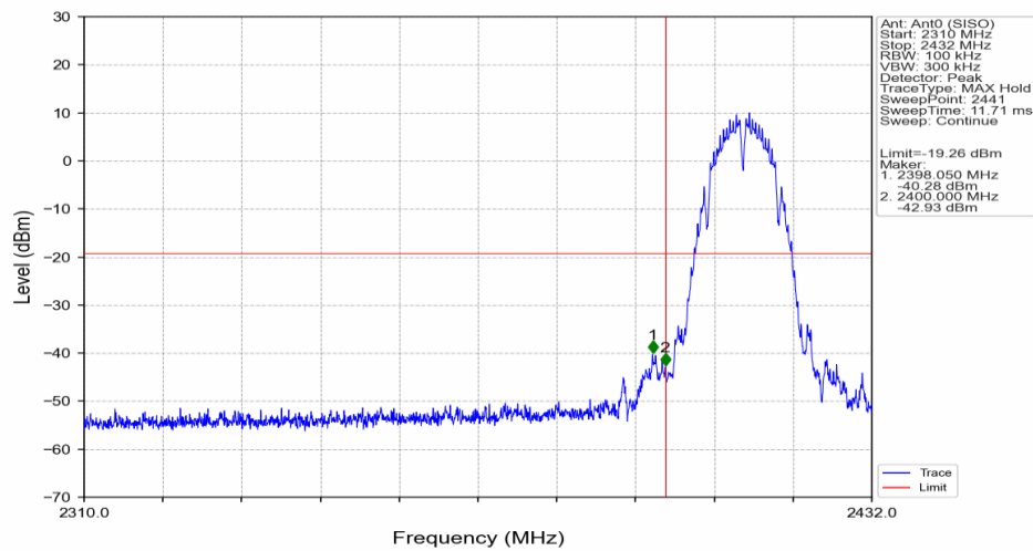
802.11b_LCH_2412MHz_Ant0 (SISO)_NTNV
