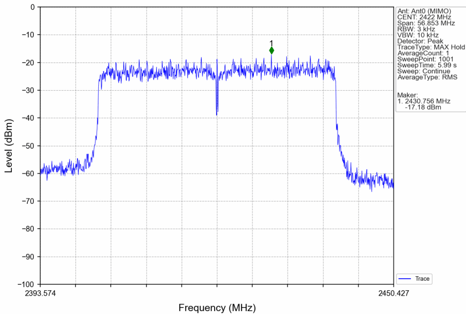
802.11ax(HEW40)_LCH_2422MHz_RU484_Left_Ant0 (MIMO)_NTNV
