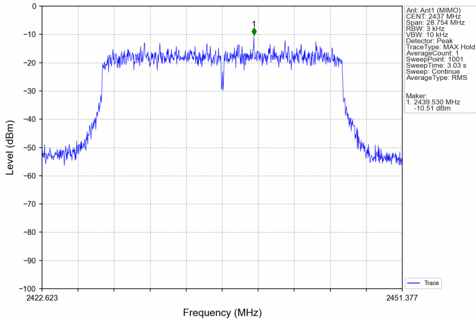
802.11ax(HEW20)_MCH_2437MHz_RU242_Left_MIMO_NTNV
