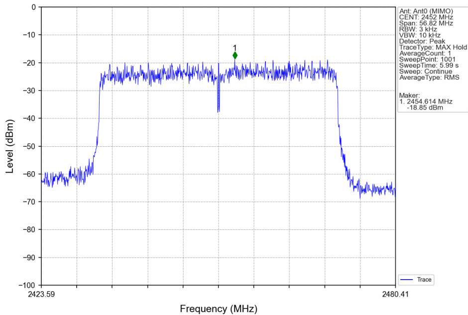
802.11ax(HEW40)_HCH_2452MHz_RU484_Left_Ant0 (MIMO)_NTNV
