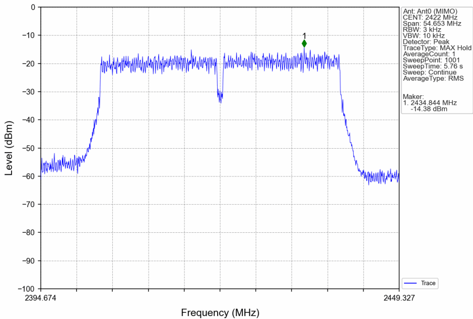
802.11n(HT40)_LCH_2422MHz_Ant0 (MIMO)_NTNV
