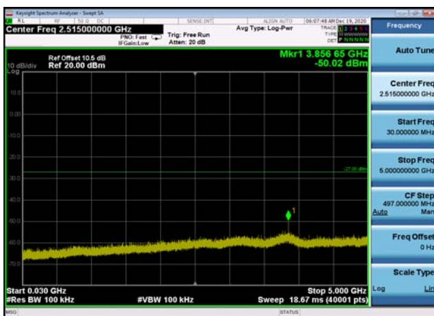
U-NII-3 ,Plot 2,30MHz~5000MHz-802.11n (20MHz),5785MHz
