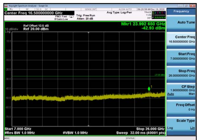
U-NII-3 ,Plot 4,7000MHz~26000MHz-802. 11n(20MHz),5825MHz
