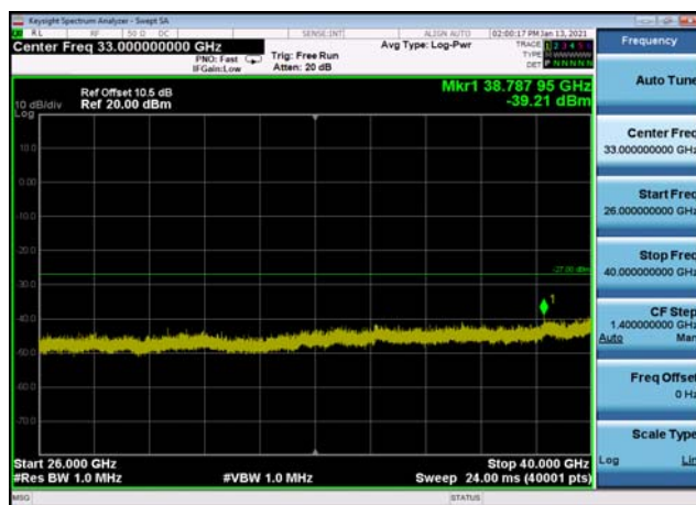
U-NII-1 ,Plot 2,26000MHz~40000MHz-802 .11a(20MHz),5240MHz
