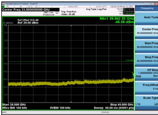
U-NII-3 ,Plot 2,26000MHz~40000MHz-802 .11ac(20MHz),5825MHz
