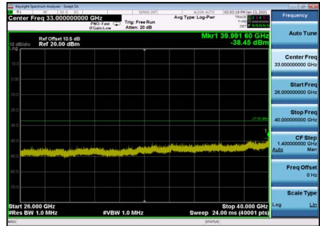
U-NII-1 ,Plot 2,26000MHz~40000MHz-802 .11n(20MHz),5240MHz
