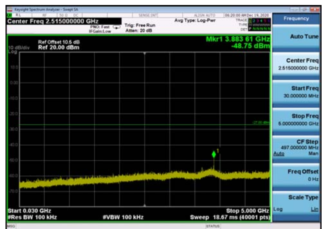
U-NII-3 ,Plot 2,30MHz~5000MHz-802.11n (20MHz),5825MHz
