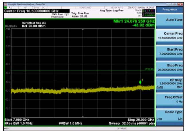
U-NII-3 ,Plot 4,7000MHz~26000MHz-802. 11ac(40MHz),5755MHz
