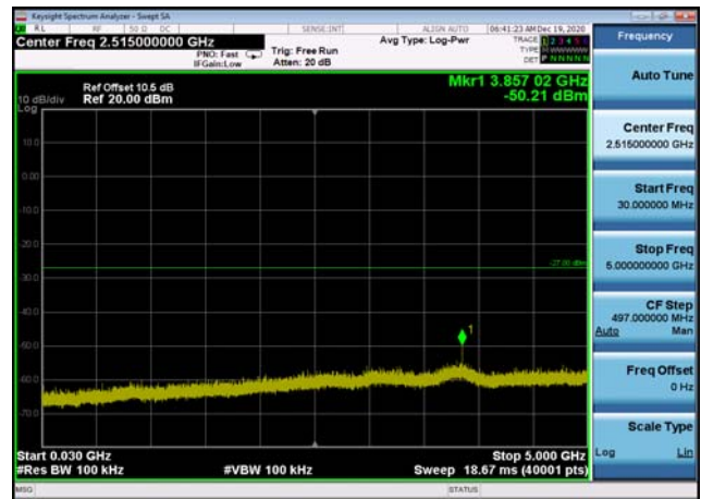
U-NII-3 ,Plot 2,30MHz~5000MHz-802.11a c(40MHz),5755MHz
