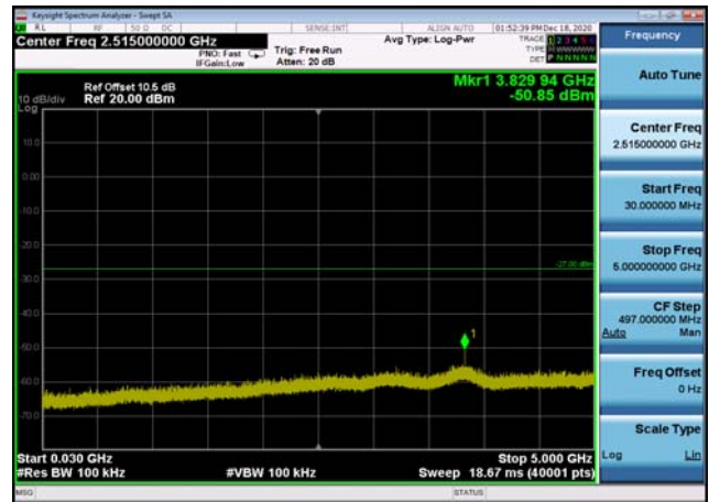
U-NII-3 ,Plot 2,30MHz~5000MHz-802.11a (20MHz),5825MHz
