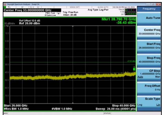
U-NII-1 ,Plot 2,26000MHz~40000MHz-802 .11ac(80MHz),5210MHz
