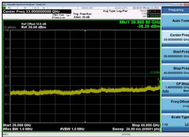
U-NII-1 ,Plot 2,26000MHz~40000MHz-802 .11ac(20MHz),5240MHz
