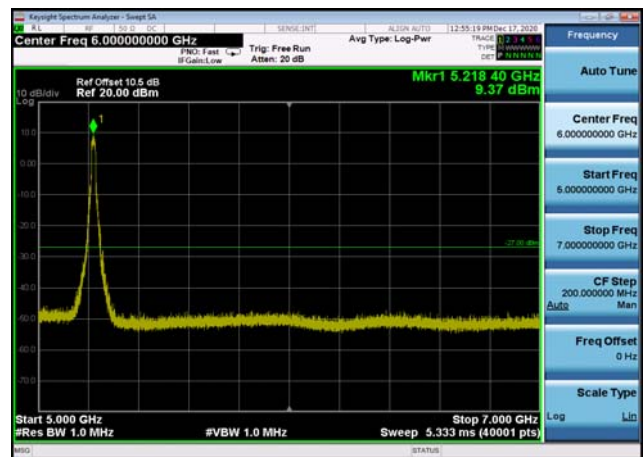
U-NII-1 ,Plot 3,5000MHz~7000MHz-802.1 1ac(20MHz),5180MHz
