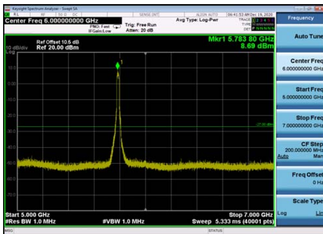
U-NII-3 ,Plot 3,5000MHz~7000MHz-802.1 1ac(40MHz),5755MHz
