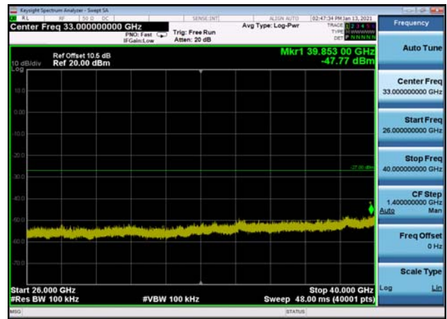
U-NII-3 ,Plot 2,26000MHz~40000MHz-802 .11a(20MHz),5825MHz
