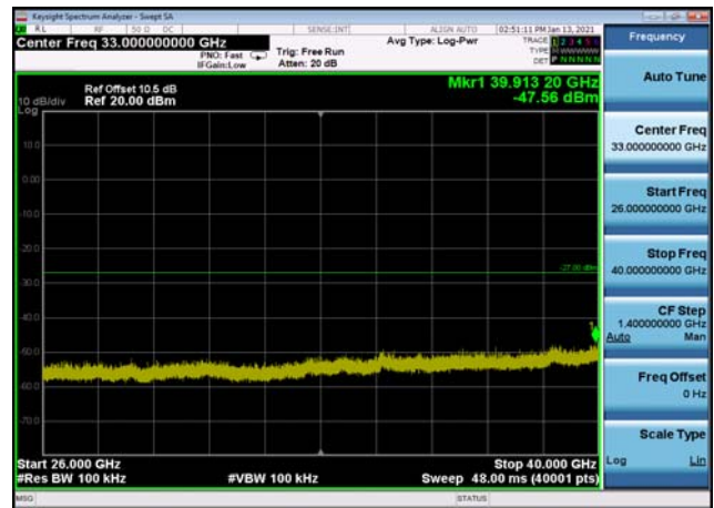
U-NII-3 ,Plot 2,26000MHz~40000MHz-802 .11n(20MHz),5825MHz
