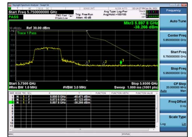
U-NII-3 ,Plot 1,Band Edge-802.11n(40M Hz),5795MHz
