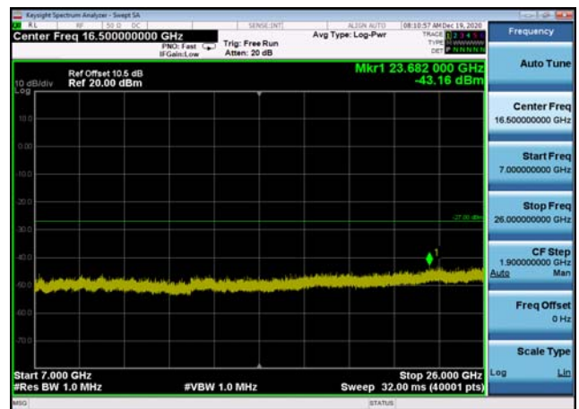
U-NII-3 ,Plot 4,7000MHz~26000MHz-802. 11ac(80MHz),5775MHz
