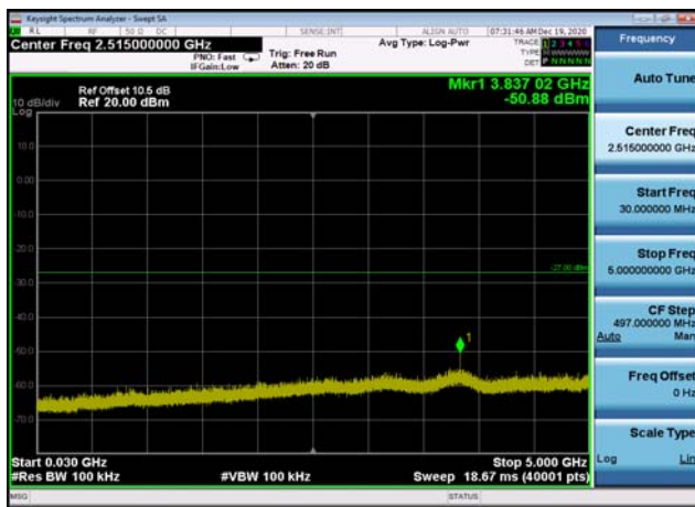
U-NII-3 ,Plot 2,30MHz~5000MHz-802.11n (40MHz),5755MHz
