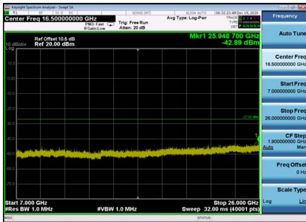
U-NII-3 ,Plot 4,7000MHz~26000MHz-802. 11ac(40MHz),5795MHz
