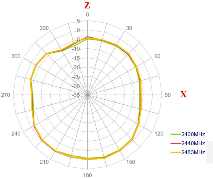
XZ-Plane
