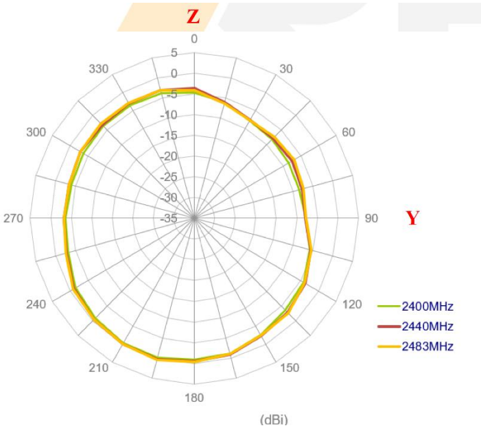
YZ-Plane
