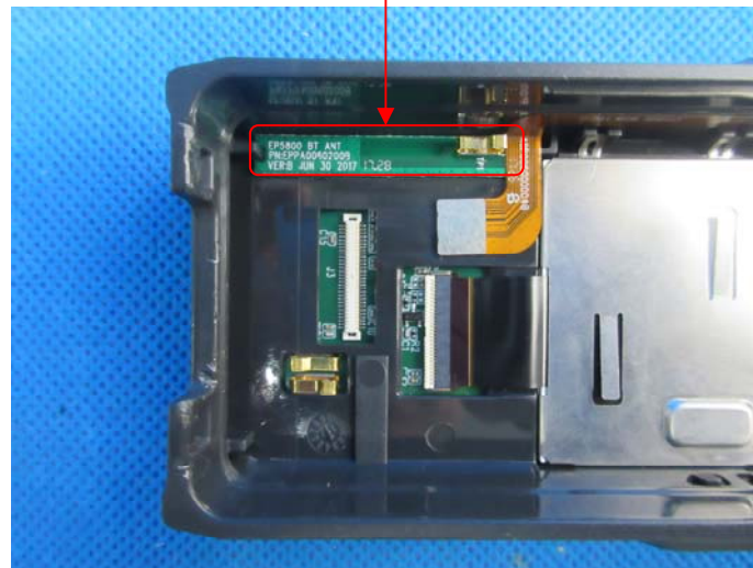
BT ANT
