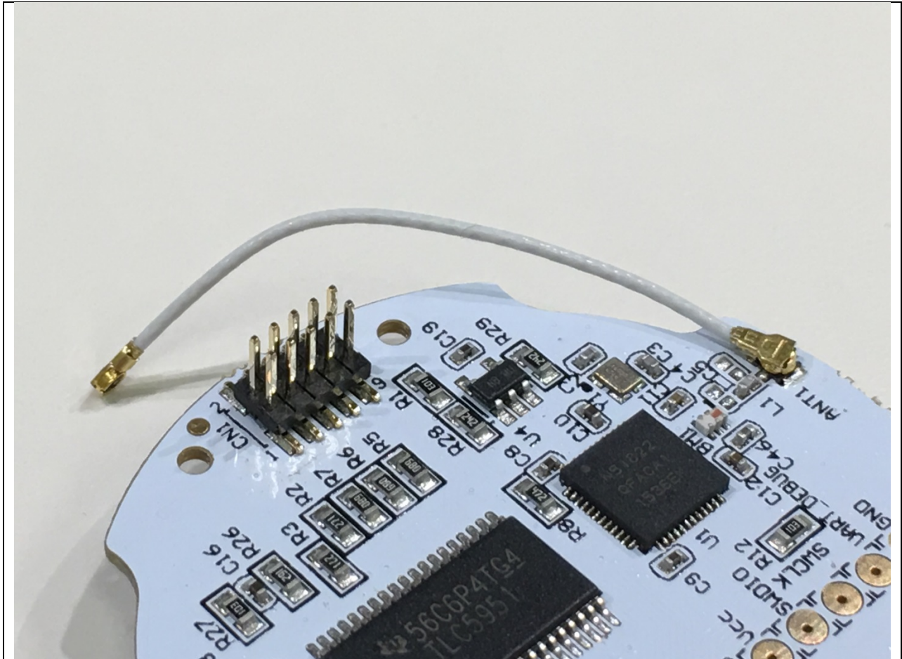
BLE Board RF cable
