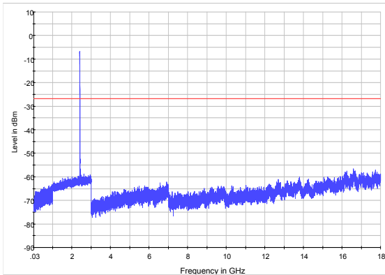
802.11b CH1 30MHz to 18GHz
