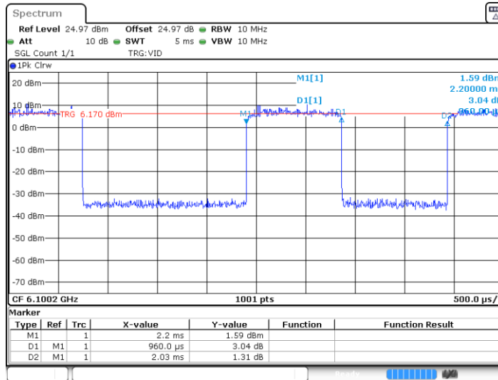
11BE320MIMO_Ant1_6105_242RU*16
