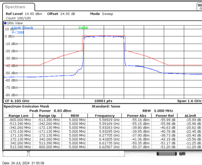
11BE320MIMO_Ant2_6105
