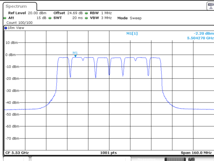
11BE80MIMO_Ant2_5530_106Tone_RU8
