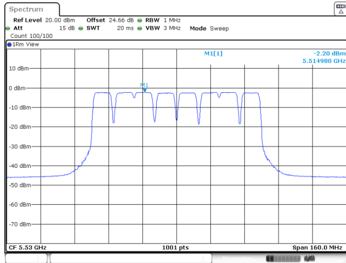
11BE80MIMO_Ant1_5530_106Tone_RU8
