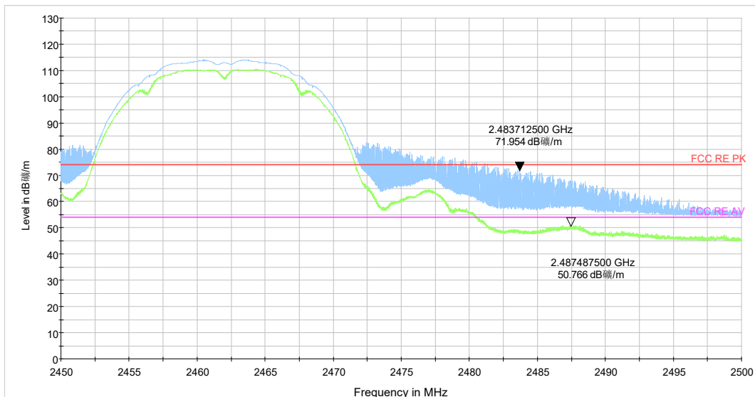
802.11n (HT20) CH11
