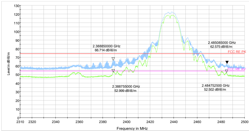
802.11b CH6
