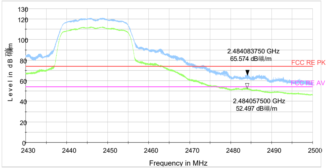
802.11g CH8
