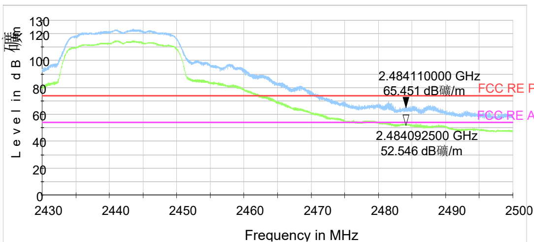
802.11g CH7
