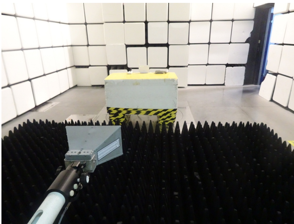
1GHz-18GHz
