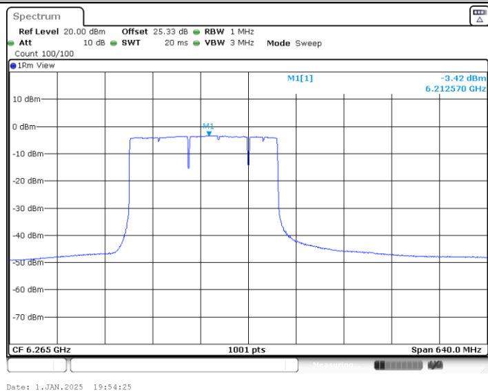
11BE320MIMO_Ant1_6265_Puncturing 80+40M_RU6
