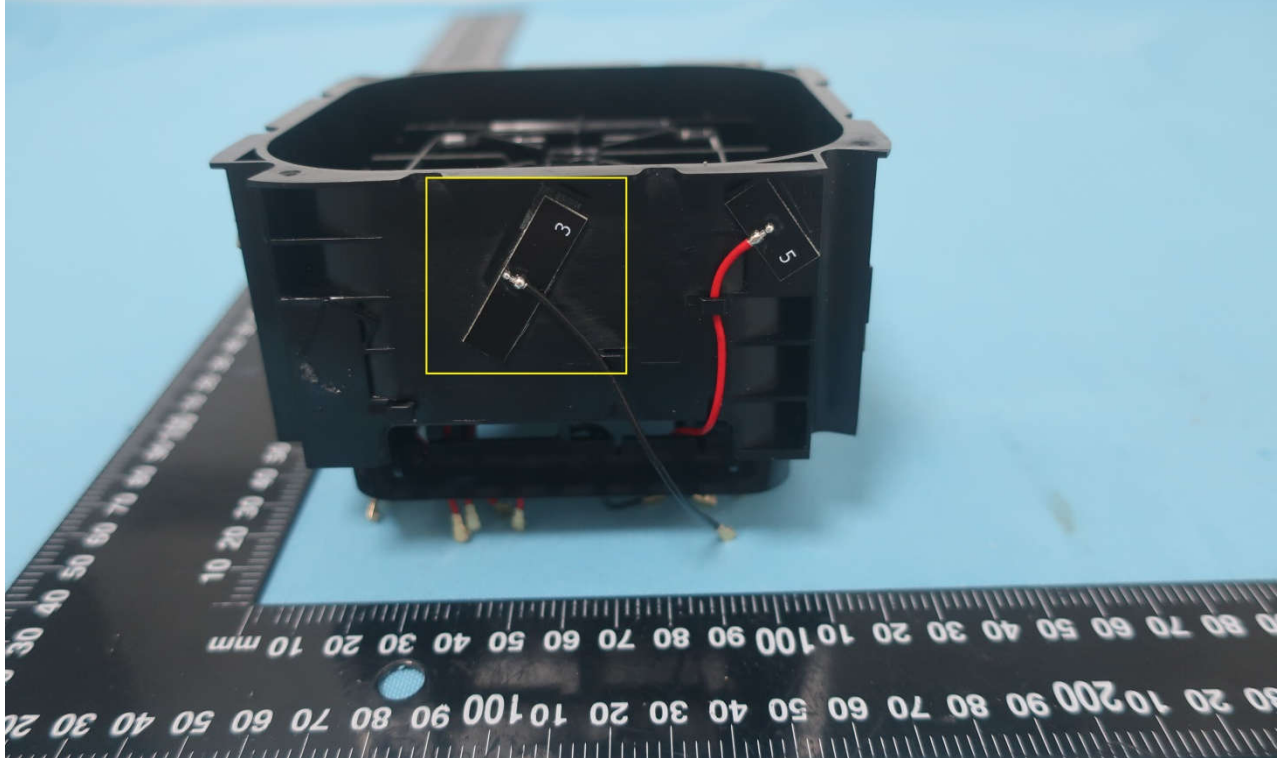
2.4G WLAN ANT3 (INPAQ Antenna)
