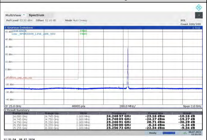
n258-b 50MHz-BPSK- High -V-1RB31
