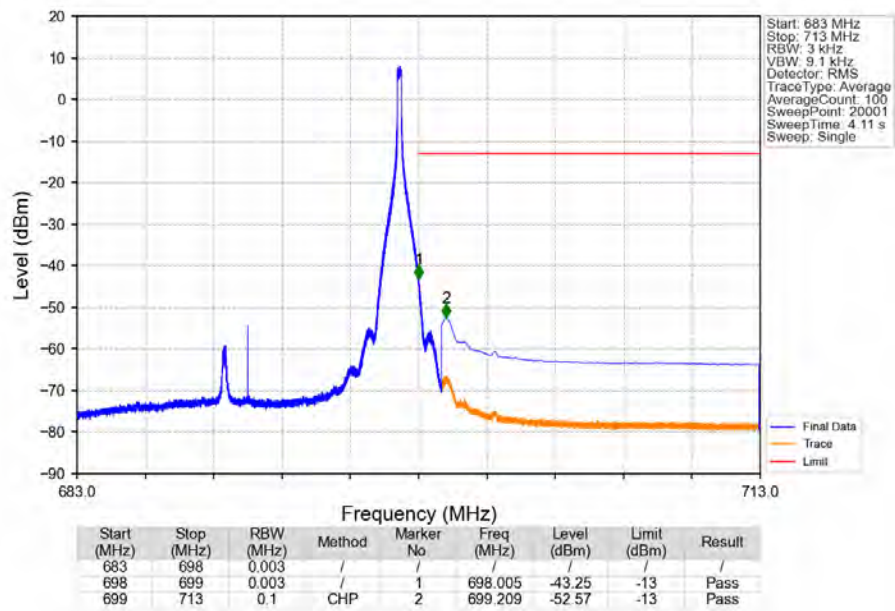
Band71 15MHz QPSK HCH 690.5MHz RB 1 74 NTV
