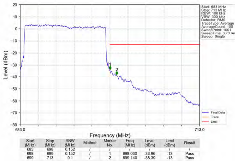
Band71 15MHz QPSK HCH 690.5MHz RB 75 0 NTV
