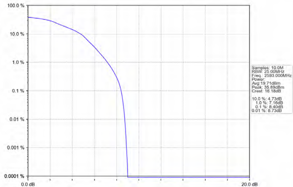
Band41_20MHz_16QAM_MCH_2593MHz_RB_100_0_NTNV
