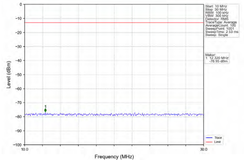
Band12 1.4MHz QPSK MCH 707.5MHz RB 1 0 NTNV
