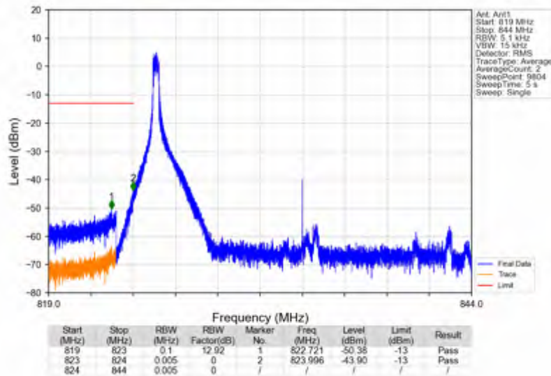
n5_30kHz_SISO_NTNV_20MHz_DFT-s-OFDM QPSK_834MHz_Inner_1RB_Left
