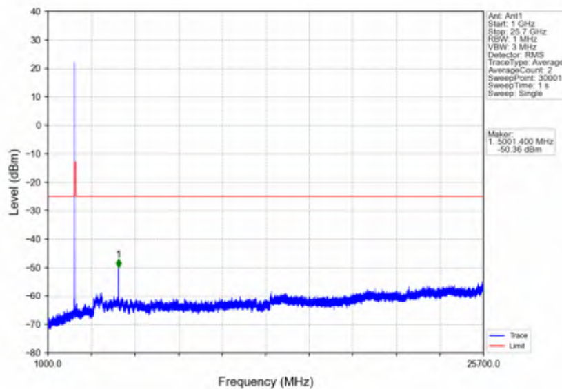
n7 15kHz SISO NTNv 5MHz DFT-s-OFDM PI/2 BPSK 2535MHz Edge 1RB Left
