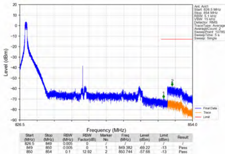
n5 30kHz SISO NTNv 20MHz DFT-s-OFDM QPSK 836.5MHz Edge 1RB Left
