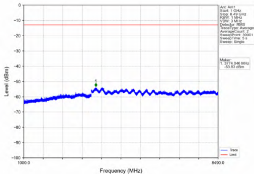
n5_30kHz_SISO_NTNV_20MHz_DFT-s-OFDM QPSK_834MHz_Inner_1RB_Left
