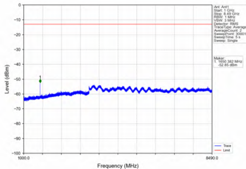
n5_30kHz_SISO_NTNV_15MHz_DFT-s-OFDM PI/2 BPSK 836.5MHz Edge 1RB_Left
