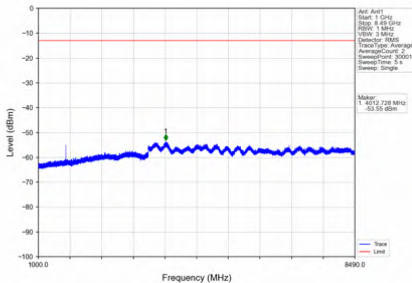
n5 30kHz SISO NTNv 10MHz DFT-s-OFDM QPSK 829MHz Edge 1RB Left
