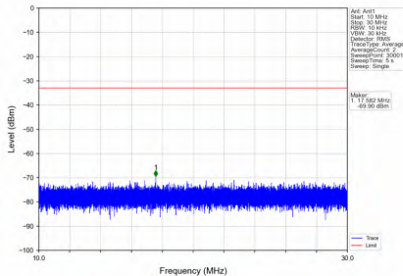
n5_30kHz_SISO_NTNV_20MHz_CP-OFDM_QPSK_834MHz_Inner_1RB_Left
