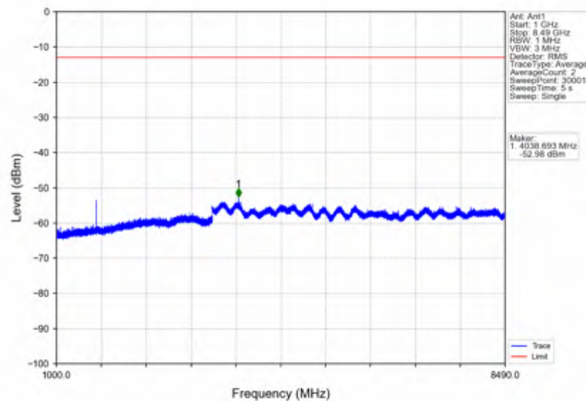
n5 30kHz SISO NTNv 10MHz DFT-s-OFDM QPSK 844MHz Edge 1RB Right
