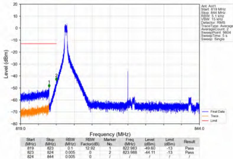
n5_30kHz_SISO_NTNV_20MHz_CP-OFDM_QPSK_834MHz_Inner_1RB_Left
