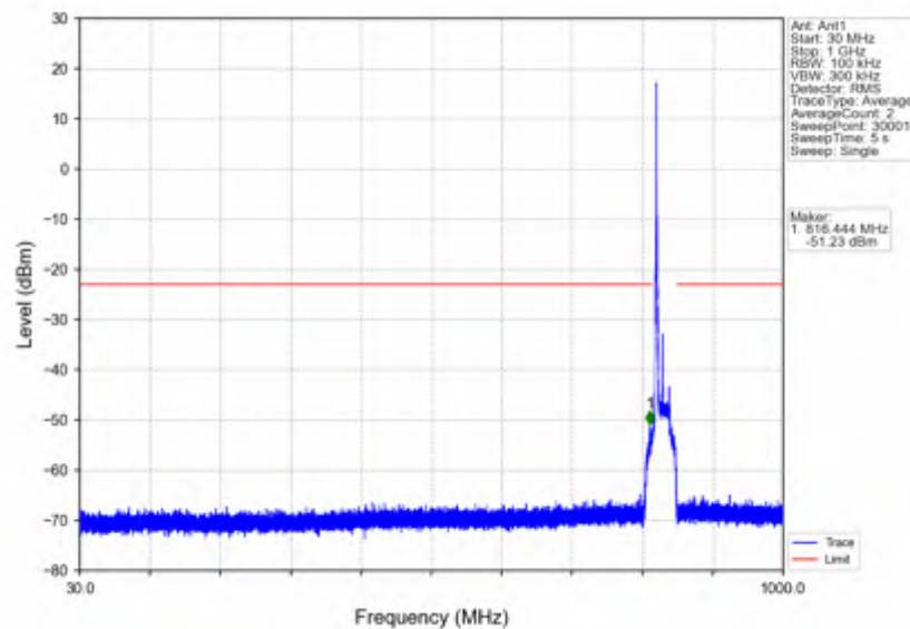
n5_30kHz_SISO_NTNV_20MHz_CP-OFDM_QPSK_834MHz_Inner_1RB_Left
