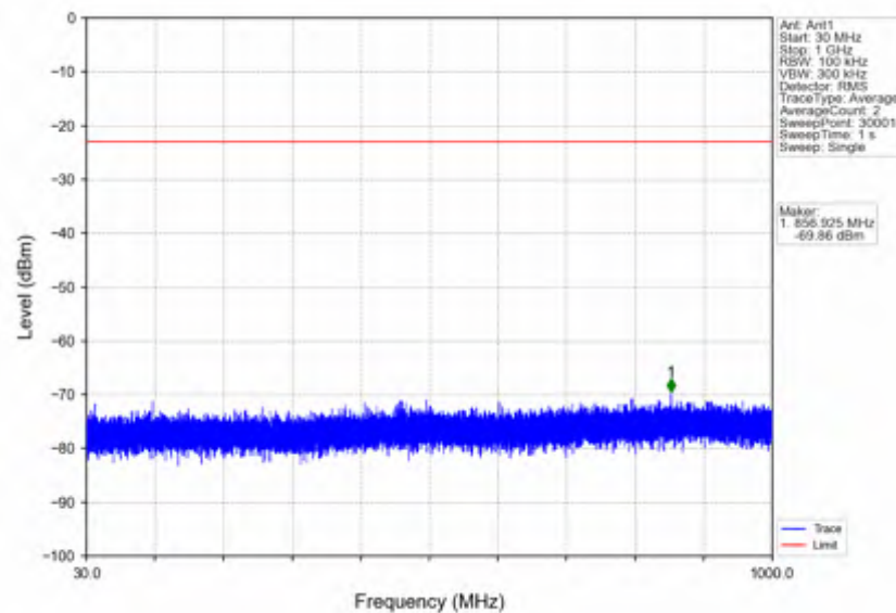
n7_15kHz_SISO_NTNV_5MHz_DFT-s-OFDM PI/2 BPSK_2502.5MHz_Inner_1RB_Left
