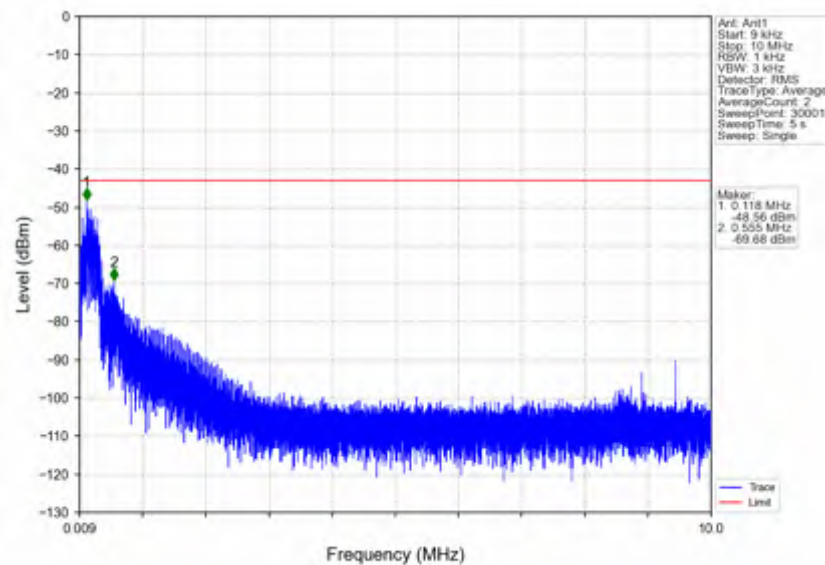
n5 30kHz SISO NTN 20MHz DFT-s-OFDM QPSK 839MHz Inner 1RB Right
