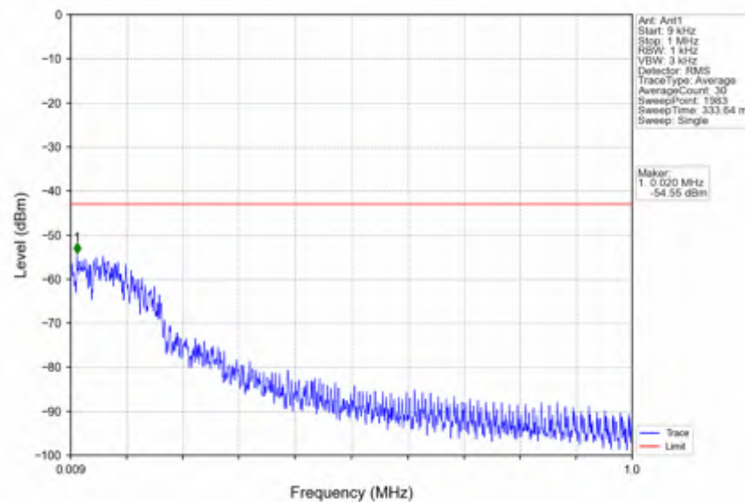
n5 15kHz SISO NTN 20MHz CP-OFDM QPSK 836.5MHz Edge 1RB Left
