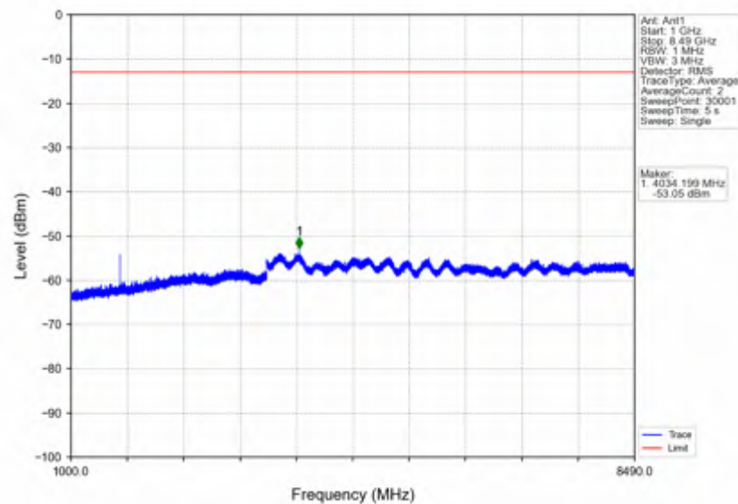
n5 30kHz SISO NTV 20MHz CP-OFDM QPSK 836.5MHz Edge 1RB Left
