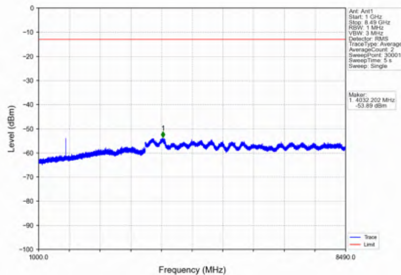
n5 30kHz SISO NTN 15MHz DFT-s-OFDM QPSK 841.5MHz Edge 1RB Right
