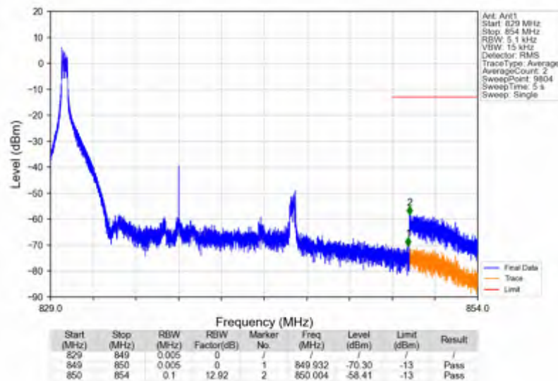
n5_30kHz_SISO_NTNV_15MHz_DFT-s-OFDM PI/2 BPSK 836.5MHz Edge 1RB_Left
