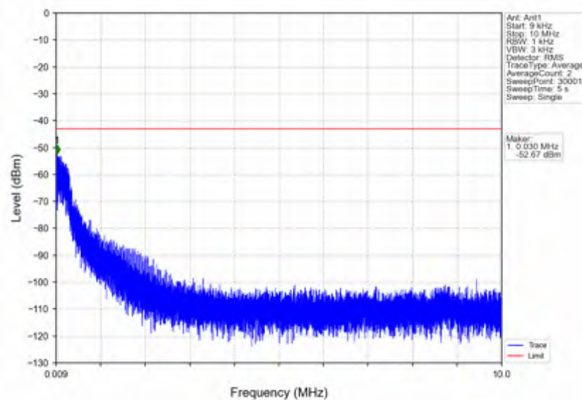
n5_30kHz_SISO_NTNV_20MHz_CP-OFDM_QPSK_834MHz_Inner_1RB_Left
