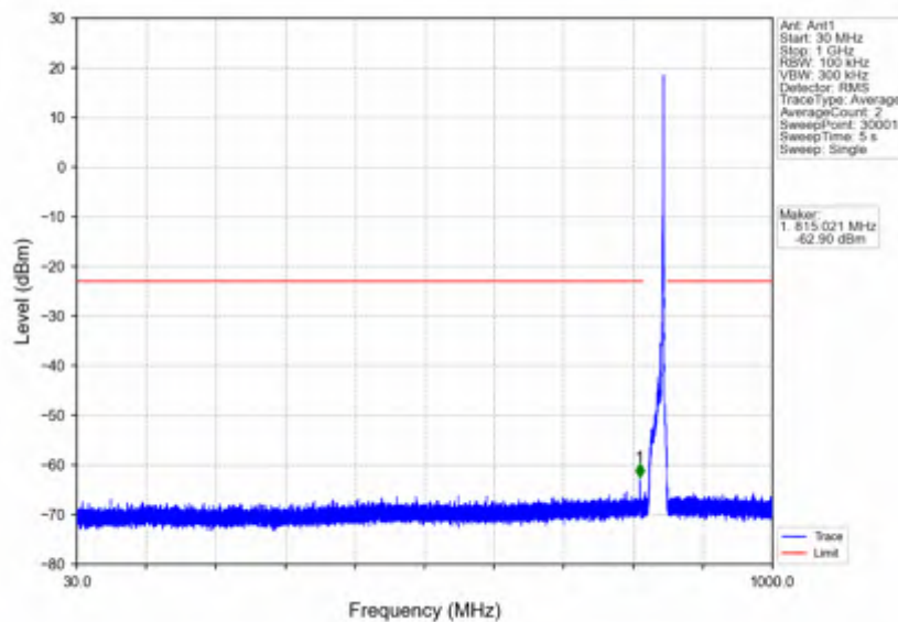
n5 30kHz SISO NTN 10MHz DFT-s-OFDM QPSK 844MHz Edge 1RB Right
