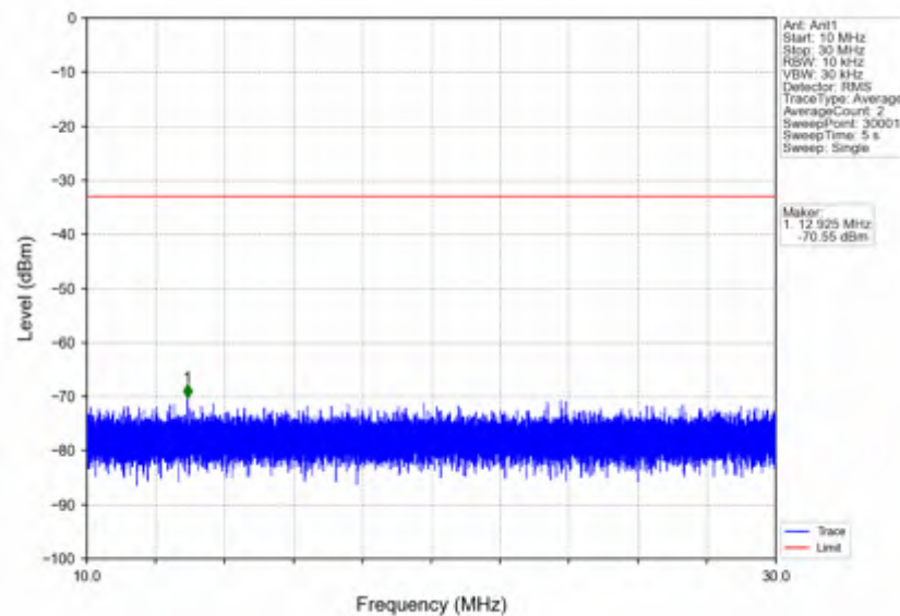
n5_30kHz_SISO_NTNV_20MHz_DFT-s-OFDM_QPSK_834MHz_Inner_1RB_Left
