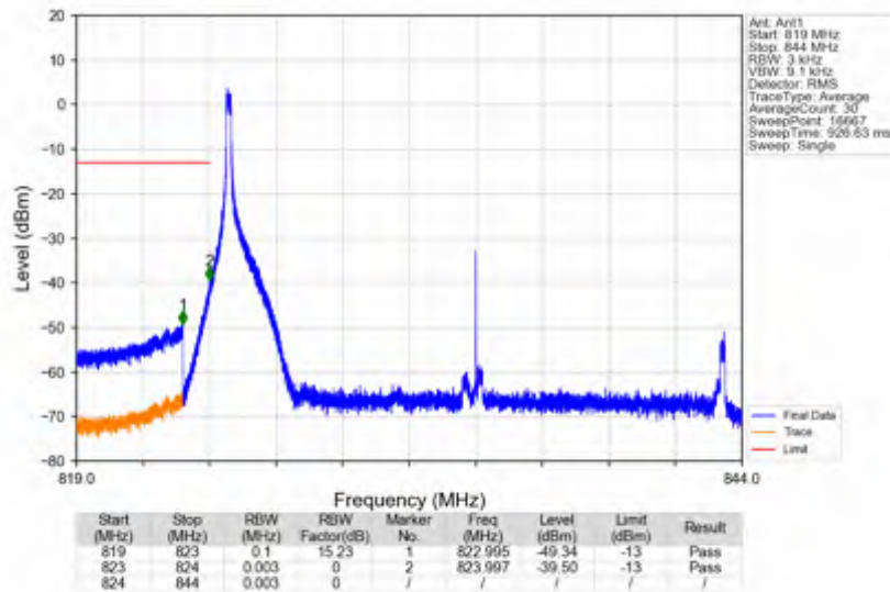
n5_15kHz_SISO_NTNV_20MHz_CP-OFDM_QPSK_834MHz_Inner_1RB_Left
