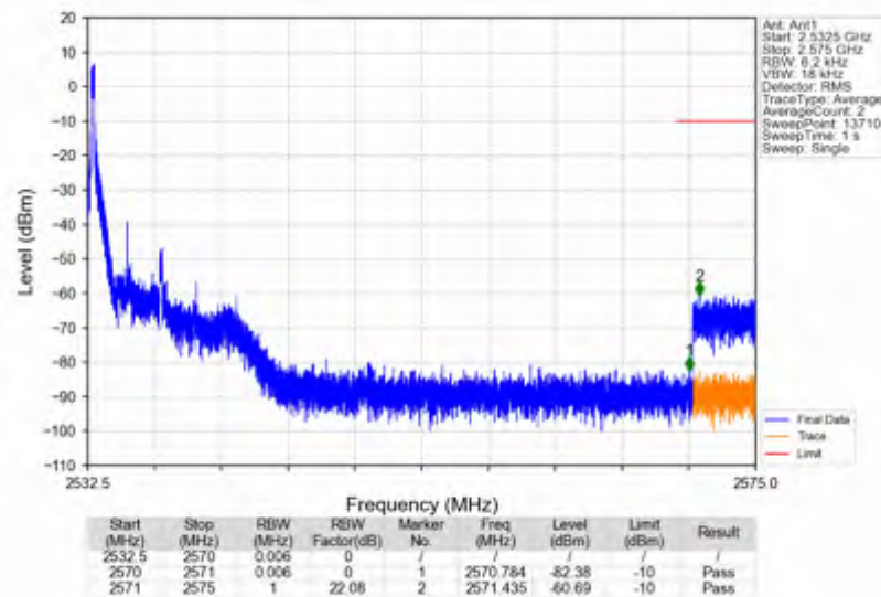
n7 15kHz SISO NTNv 5MHz DFT-s-OFDM PI/2 BPSK 2535MHz Edge 1RB Left
