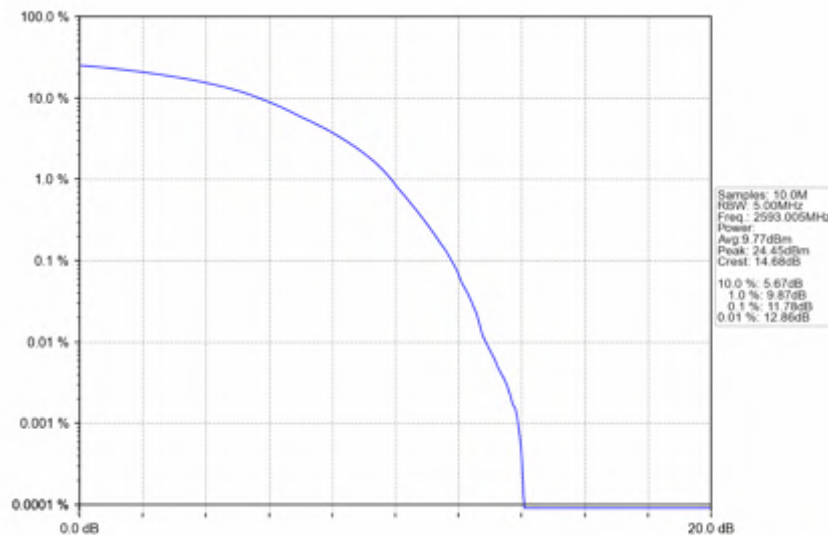
n41_15kHz_SISO_NTNV_30MHz_DFT-s-OFDM_256_QAM_2593.005MHz_Outer_Full
