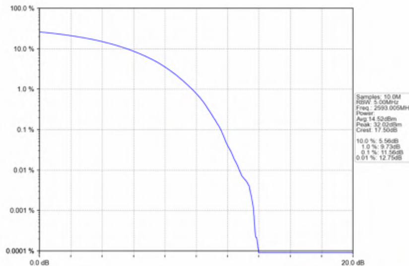
n41_15kHz_SISO_NTNV_15MHz_CP-OFDM_QPSK_2593.005MHz_Outer_Full
