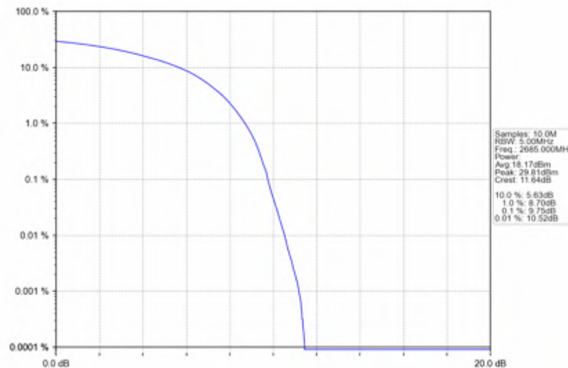
n41_15kHz_SISO_NTNV_10MHz_DFT-s-OFDM_16_QAM_2685MHz_Outer_Full
