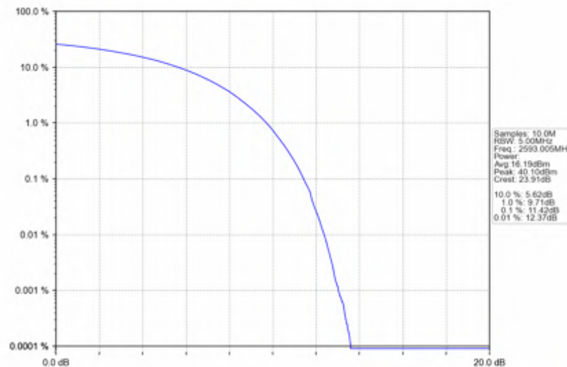
n41_15kHz_SISO_NTNV_10MHz_CP-OFDM_16_QAM_2593.005MHz_Outer_Full
