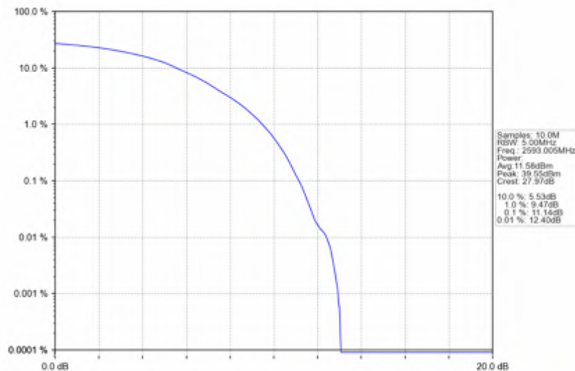
n41_15kHz_SISO_NTNV_50MHz_DFT-s-OFDM_PI/2_BPSK_2593.005MHz_Outer_Full
