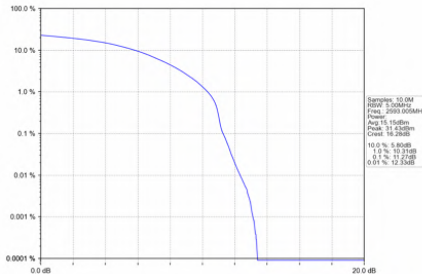
n41_15kHz_SISO_NTNV_15MHz_DFT-s-OFDM_16_QAM_2593.005MHz_Outer_Full
