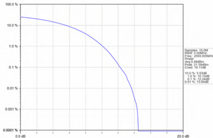
n41_15kHz_SISO_NTNV_50MHz_CP-OFDM_256_QAM_2593.005MHz_Outer_Full
