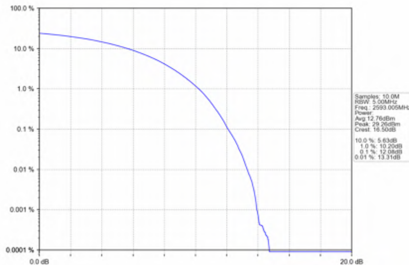
n41_15kHz_SISO_NTNV_20MHz_CP-OFDM_16 QAM_2593.005MHz_Outer_Full
