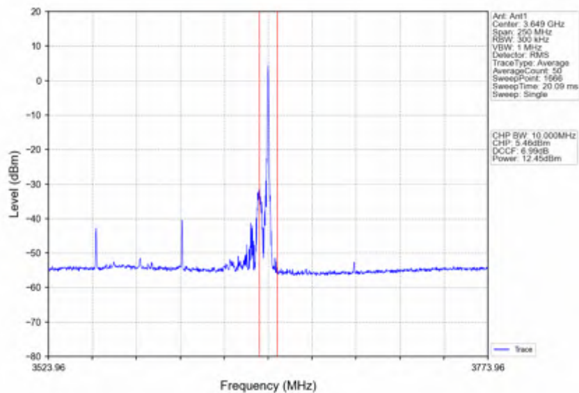
n78d 30kHz SISO NTN 100MHz CP-OFDM QPSK 3600MHz Edge 1RB Right
