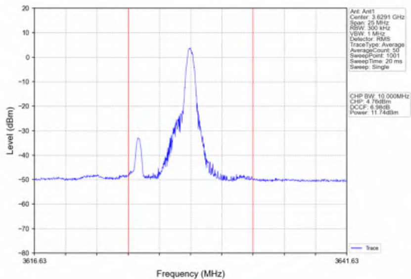
n78d 30kHz SISO NTV 10MHz CP-OFDM QPSK 3624.99MHz Edge 1RB Right
