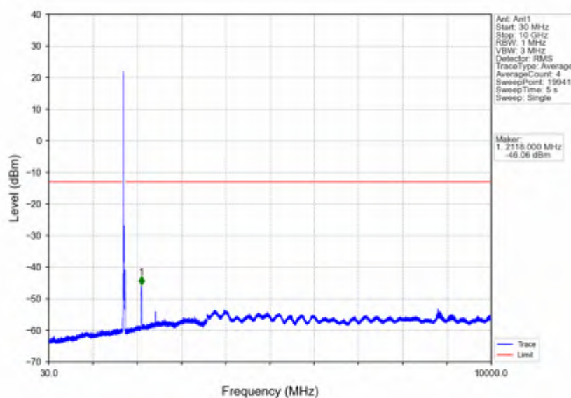
Band66_20MHz_QPSK_LCH_1720MHz_RB_1_0_NTNV
