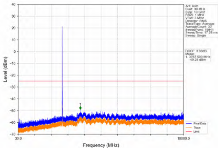
Band41_10MHz_256QAM_HCH_2685MHz_RB_1_0_NTNV
