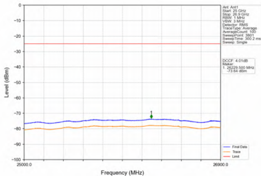
Band41_20MHz_QPSK_LCH_2506MHz_RB_1_0_NTNV
