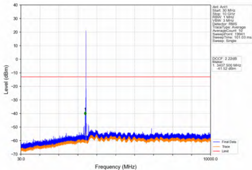
Band42a_10MHz_16QAM_LCH_3455MHz_RB_1_0_NTNV
