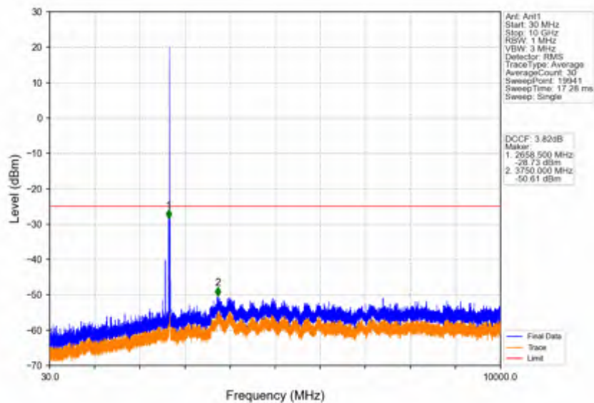
Band41_10MHz_QPSK_HCH_2685MHz_RB_1_0_NTNV
