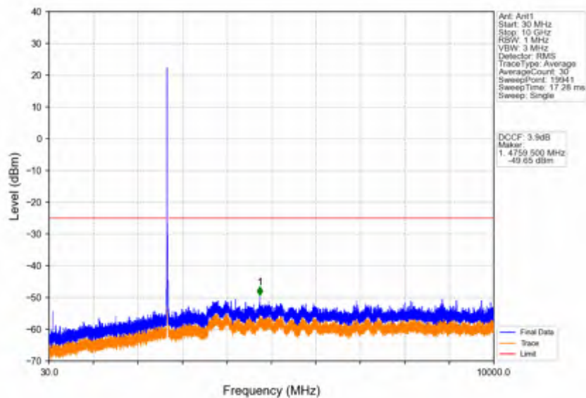
Band41_15MHz_QPSK_HCH_2682.5MHz_RB_1_0_NTNV
