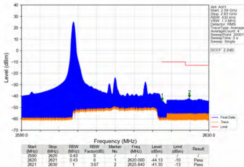
Band38_20MHz_QPSK_HCH_2610MHz_RB_1_99_NTNV
