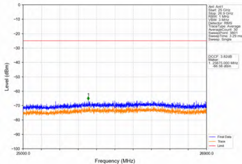
Band41_10MHz_16QAM_HCH_2685MHz_RB_1_0_NTNV
