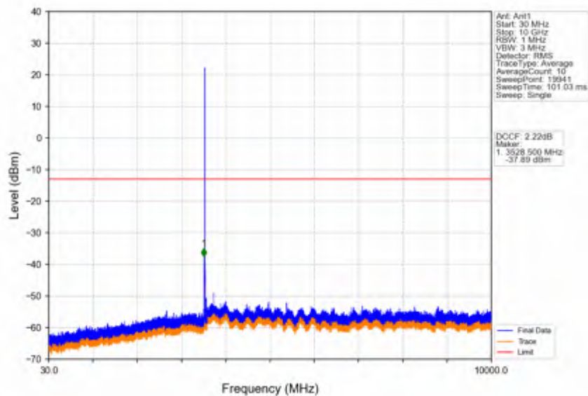
Band42a 5MHz_QPSK_HCH_3547.5MHz_RB_1_0_NTNV
