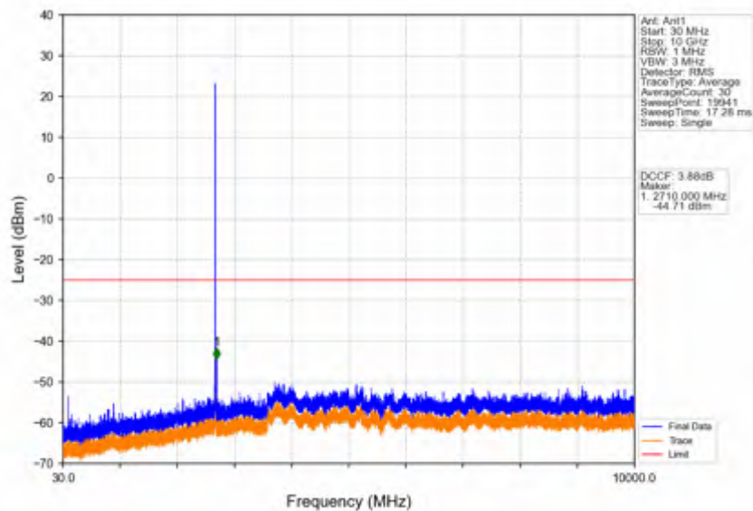
Band41_5MHz_QPSK_HCH_2687.5MHz_RB_1_0_NTNV
