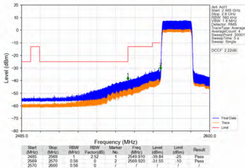
Band38_20MHz_256QAM_LCH_2580MHz_RB_100_0_NTNV
