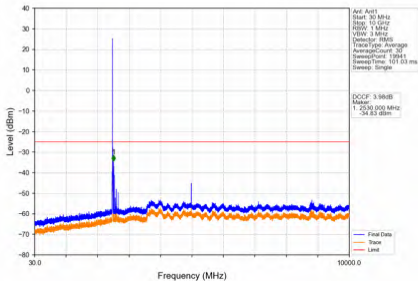
Band41_10MHz_16QAM_LCH_2501MHz_RB_1_0_NTNV
