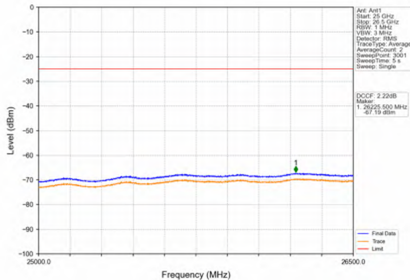
Band38_20MHz_QPSK_HCH_2610MHz_RB_1_99_NTNV
