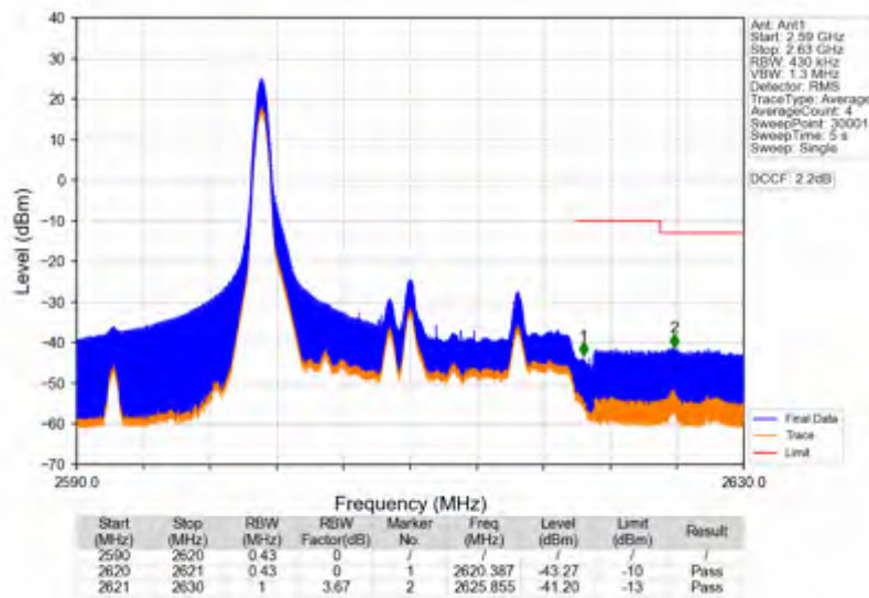
Band38_20MHz_64QAM_HCH_2610MHz_RB_1_99_NTNV
