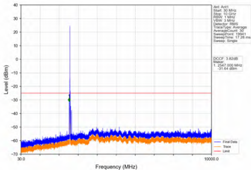
Band41_10MHz_16QAM_MCH_2593MHz_RB_1_0_NTNV
