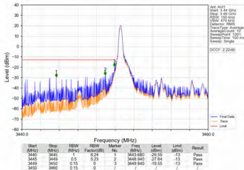
Band42a_10MHz_16QAM_LCH_3455MHz_RB_1_0_NTNV
