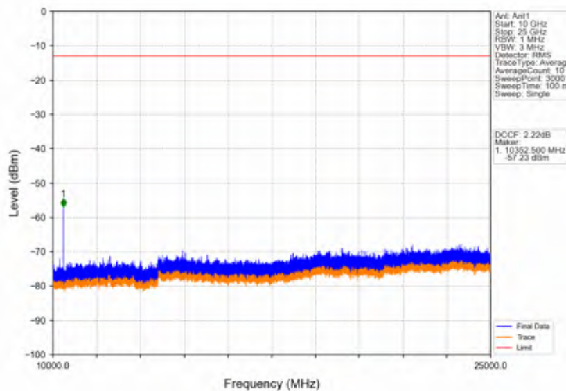
Band42a_10MHz_16QAM_LCH_3455MHz_RB_1_0_NTNV
