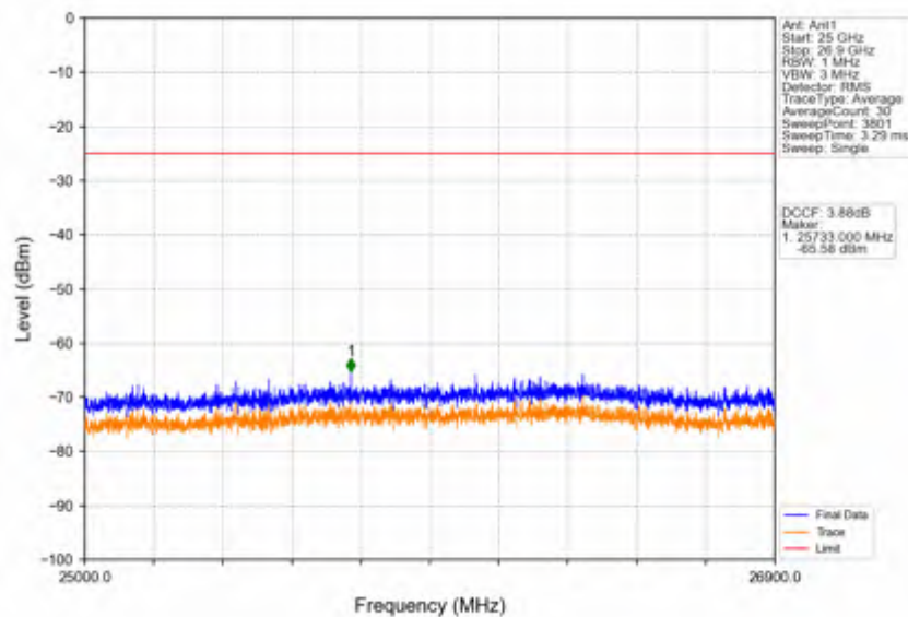
Band41_5MHz_QPSK_HCH_2687.5MHz_RB_1_24_NTNV
