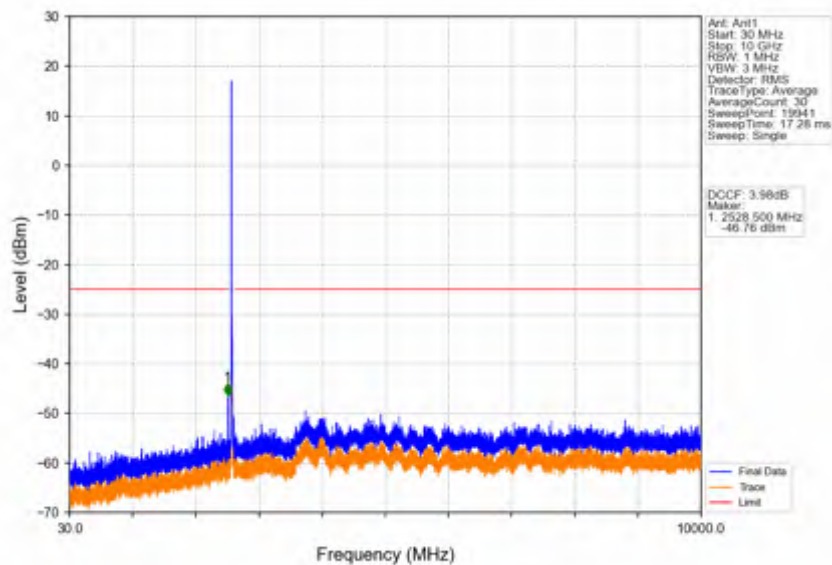
Band41_20MHz_256QAM_MCH_2593MHz_RB_1_0_NTNV
