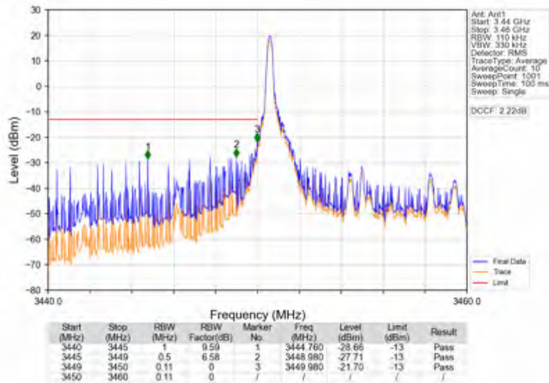
Band42a_10MHz_16QAM_LCH_3455MHz_RB_50_0_NTNV
