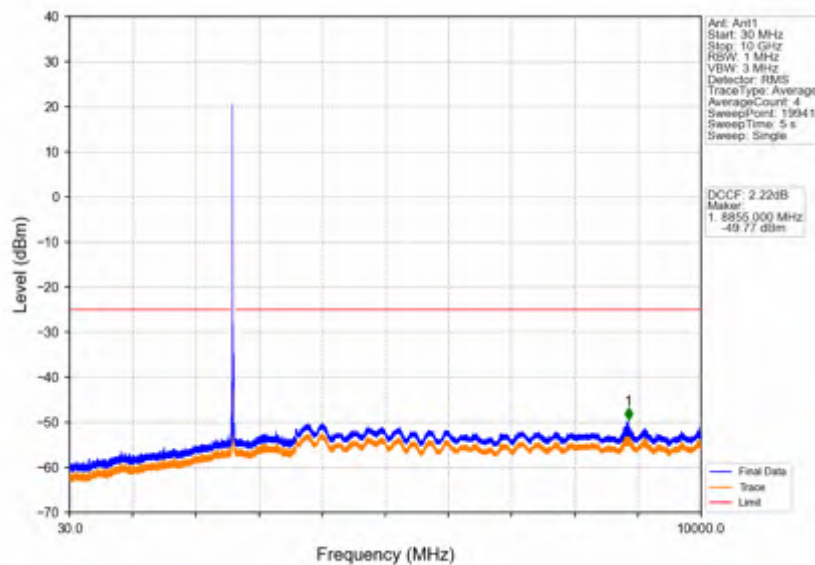
Band38_20MHz_256QAM_HCH_2610MHz_RB_1_0_NTNV
