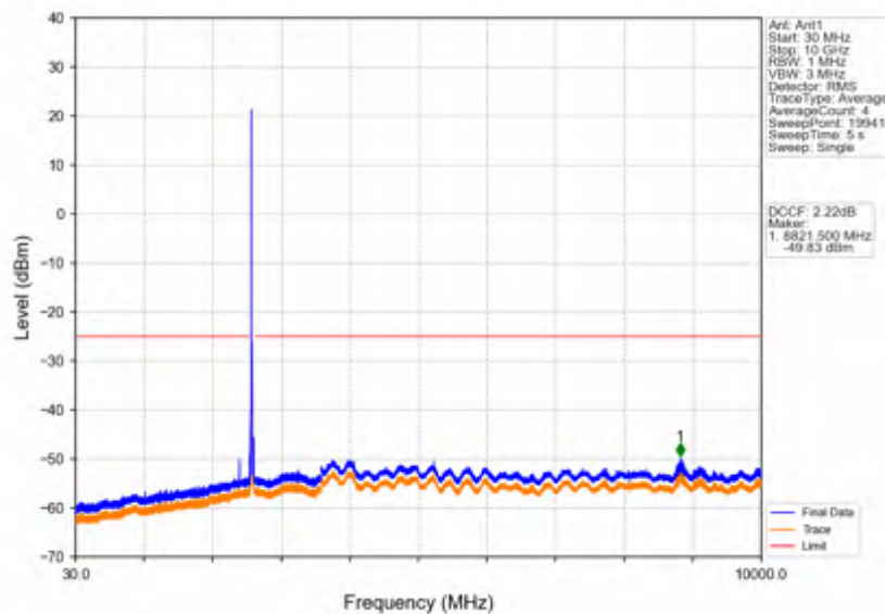
Band38_20MHz_QPSK_MCH_2595MHz_RB_1_0_NTNV
