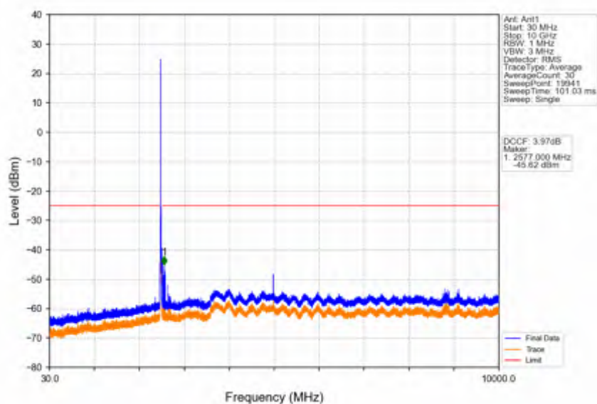
Band41_15MHz_QPSK_LCH_2503.5MHz_RB_1_0_NTNV
