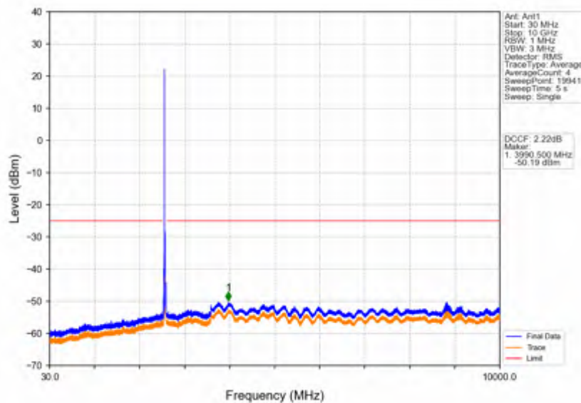
Band38_20MHz_16QAM_LCH_2580MHz_RB_1_0_NTNV
