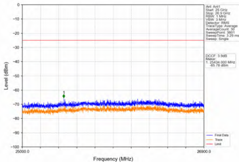
Band41_15MHz_QPSK_HCH_2682.5MHz_RB_1_74_NTNV
