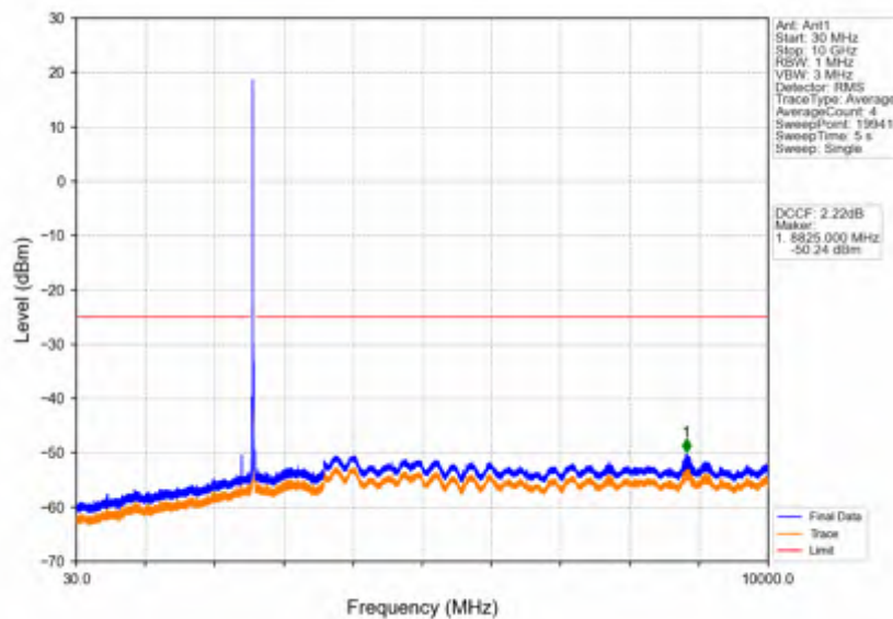
Band38_20MHz_256QAM_LCH_2580MHz_RB_1_0_NTNV
