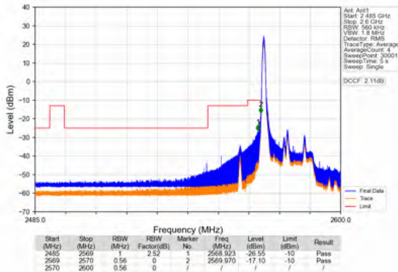
Band38_20MHz_QPSK_LCH_2580MHz_RB_100_0_NTNV
