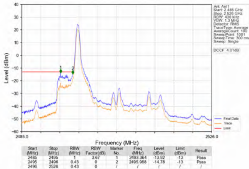
Band41 20MHz QPSK LCH 2506MHz RB 100 0 NTNV
