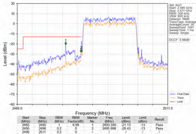
Band41_10MHz_256QAM_LCH_2501MHz_RB_50_0_NTNV
