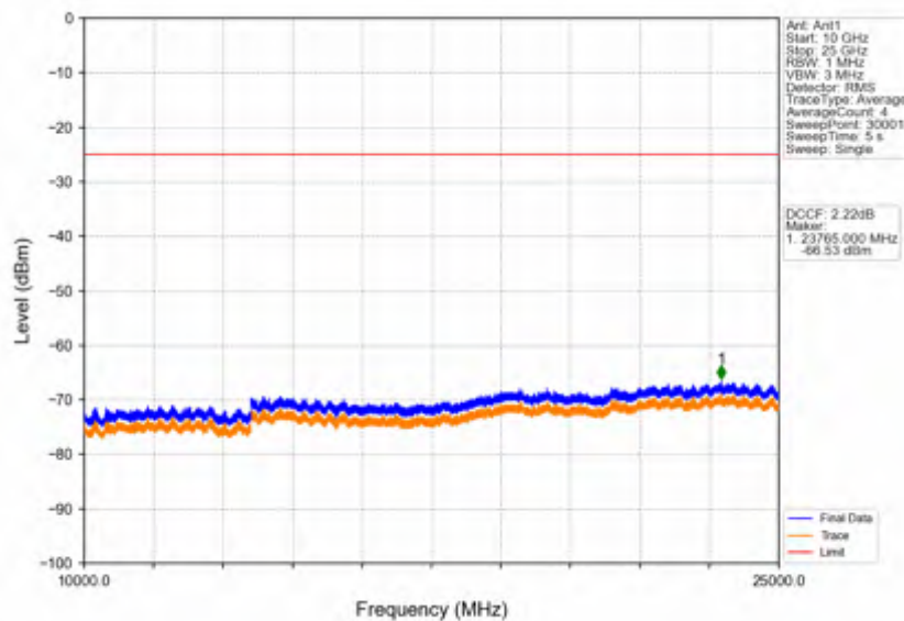
Band38_20MHz_256QAM_LCH_2580MHz_RB_1_0_NTNV
