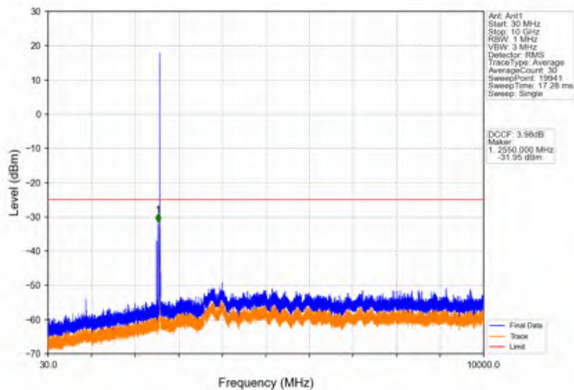
Band41_10MHz_256QAM_MCH_2593MHz_RB_1_0_NTNV
