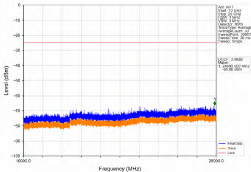
Band41_10MHz_256QAM_LCH_2501MHz_RB_1_0_NTNV
