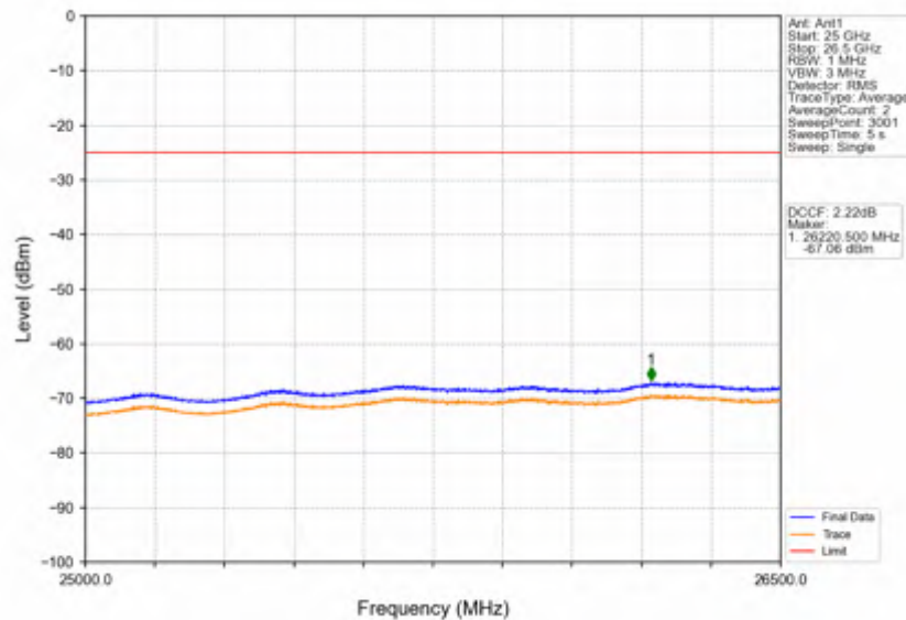
Band38_20MHz_256QAM_HCH_2610MHz_RB_1_0_NTNV
