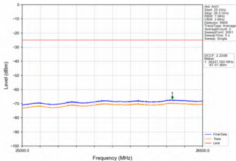
Band38_20MHz_256QAM_LCH_2580MHz_RB_100_0_NTNV
