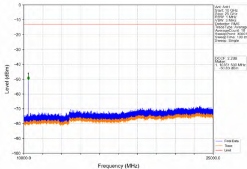
Band42a_10MHz_QPSK_LCH_3455MHz_RB_1_0_NTNV
