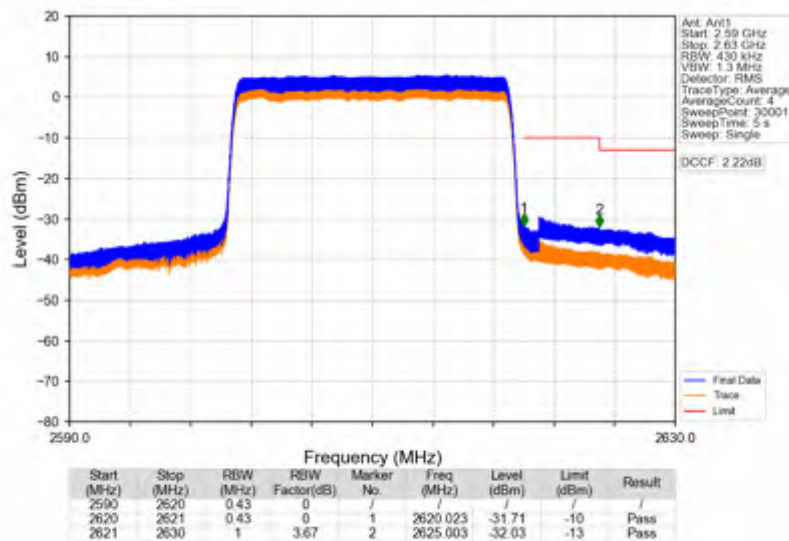
Band38_20MHz_256QAM_HCH_2610MHz_RB_100_0_NTNV
