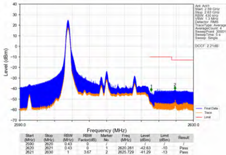
Band38_20MHz_16QAM_HCH_2610MHz_RB_1_99_NTNV
