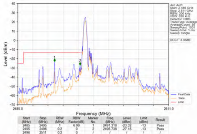
Band41_10MHz_16QAM_LCH_2501MHz_RB_50_0_NTNV
