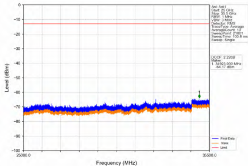
Band42a_10MHz_QPSK_MCH_3500MHz_RB_1_0_NTNV
