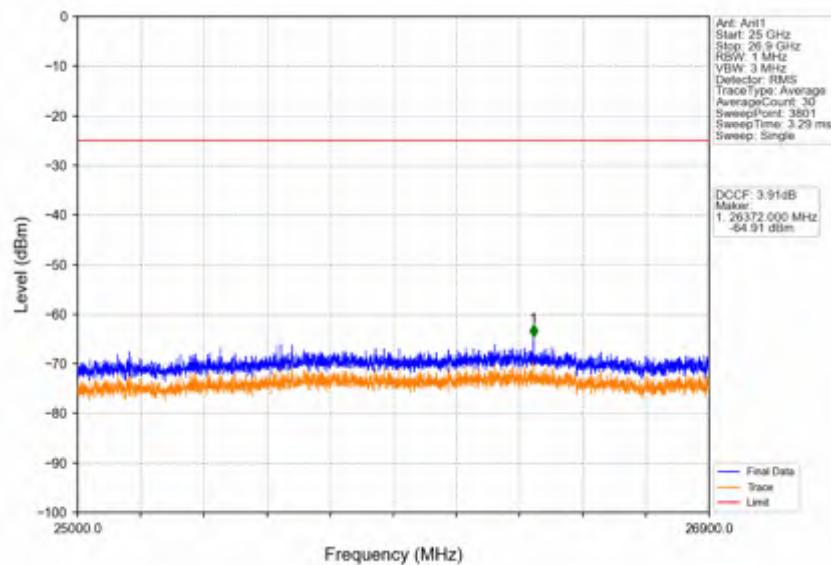
Band41_20MHz_QPSK_HCH_2680MHz_RB_1_99_NTNV
