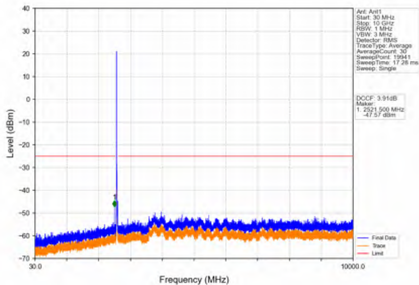
Band41_20MHz_16QAM_MCH_2593MHz_RB_1_0_NTNV
