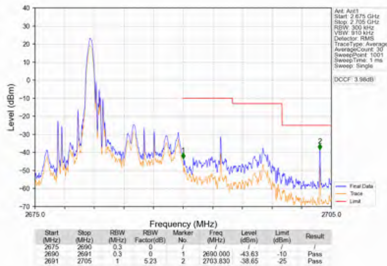
Band41_10MHz_64QAM_HCH_2685MHz_RB_1_49_NTNV
