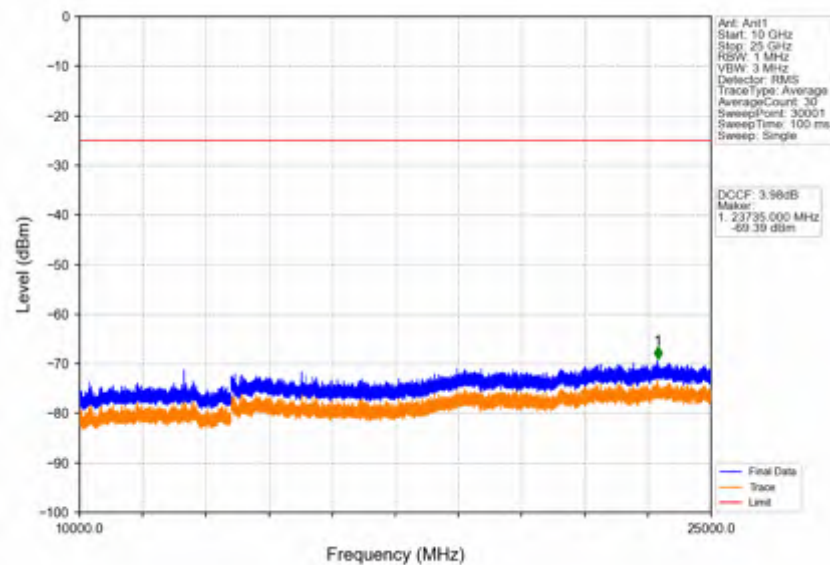
Band41_5MHz_QPSK_LCH_2498.5MHz_RB_1_0_NTNV
