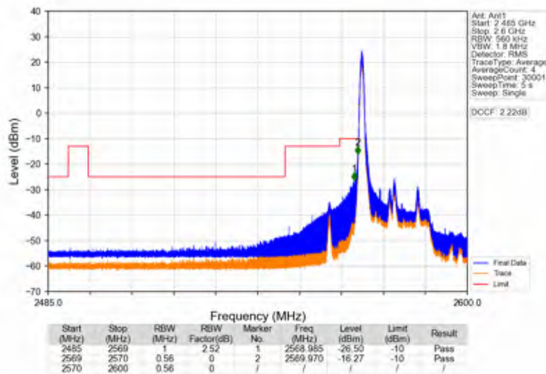
Band38_20MHz_16QAM_LCH_2580MHz_RB_100_0_NTNV
