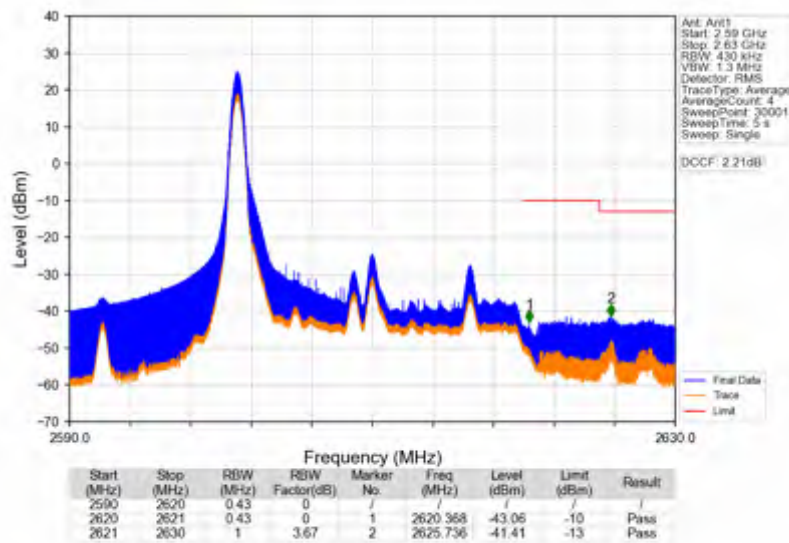
Band38_20MHz_16QAM_HCH_2610MHz_RB_100_0_NTNV
