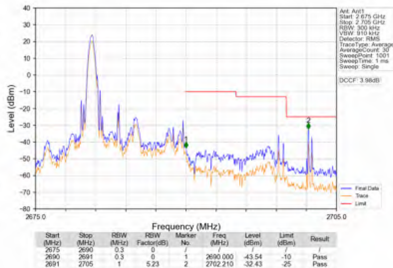
Band41_10MHz_QPSK_HCH_2685MHz_RB_1_49_NTNV
