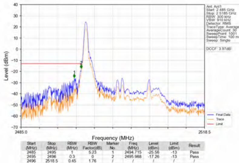
Band41_15MHz_QPSK_LCH_2503.5MHz_RB_1_0_NTNV
