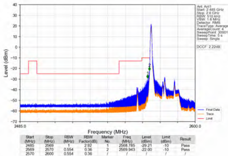
Band38_20MHz_256QAM_LCH_2580MHz_RB_1_0_NTNV
