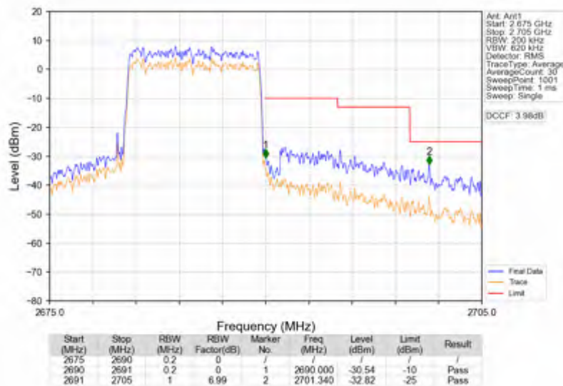
Band41_10MHz_256QAM_HCH_2685MHz_RB_50_0_NTNV
