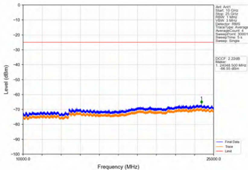
Band38_20MHz_256QAM_MCH_2595MHz_RB_1_0_NTNV
