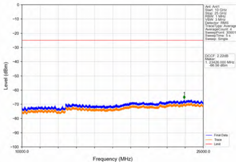
Band38_20MHz_16QAM_LCH_2580MHz_RB_1_0_NTNV
