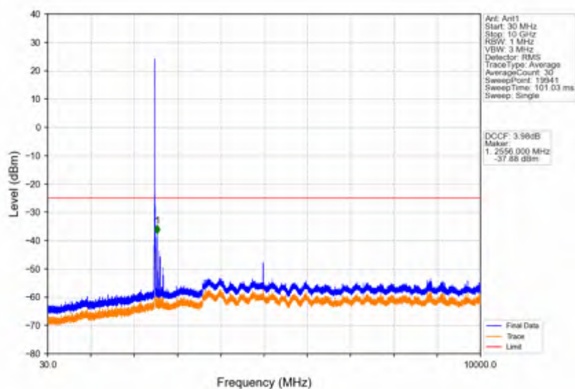
Band41_10MHz_QPSK_LCH_2501MHz_RB_1_0_NTNV
