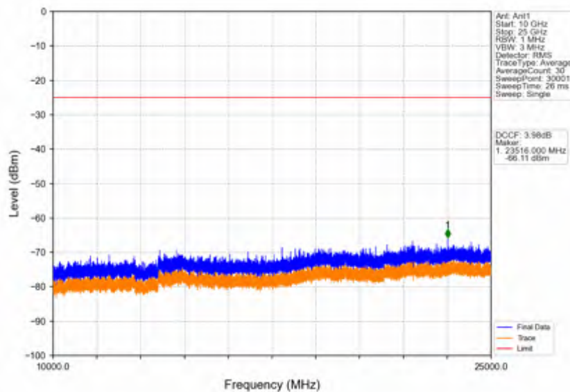
Band41_5MHz_256QAM_MCH_2593MHz_RB_1_0_NTNV
