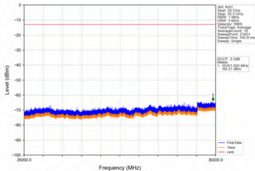
Band42a_10MHz_QPSK_LCH_3455MHz_RB_1_0_NTNV
