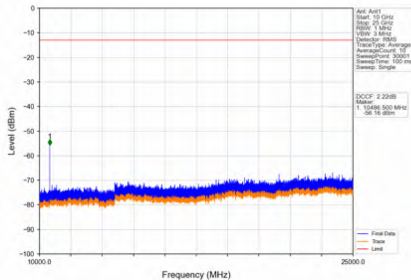
Band42a_10MHz_QPSK_MCH_3500MHz_RB_1_0_NTNV
