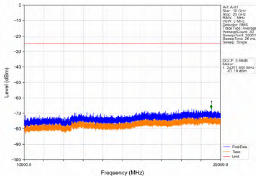
Band41_20MHz_256QAM_MCH_2593MHz_RB_1_0_NTNV
