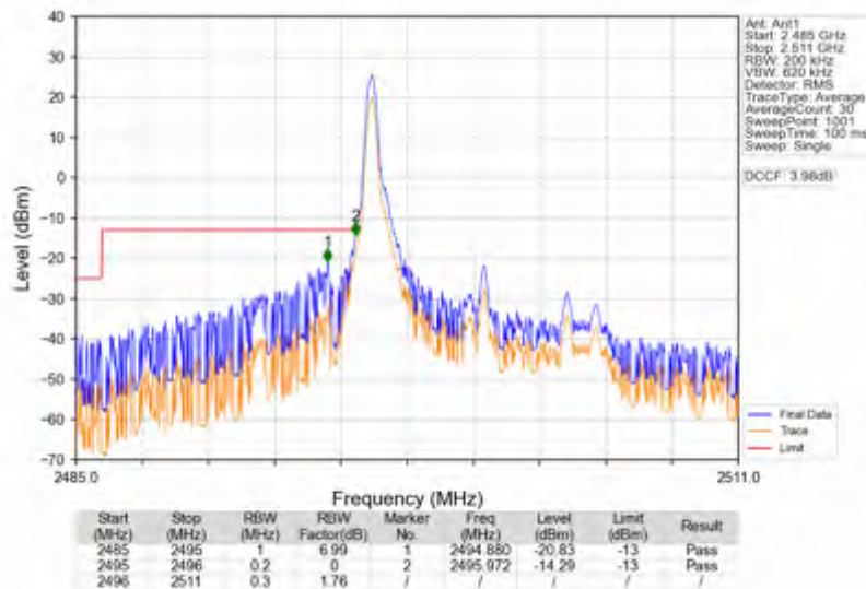
Band41_10MHz_QPSK_LCH_2501MHz_RB_1_0_NTNV
