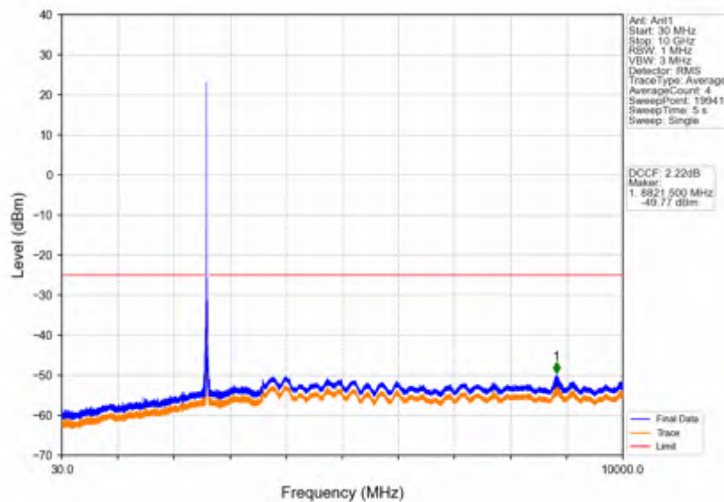
Band38_20MHz_QPSK_HCH_2610MHz_RB_1_0_NTNV
