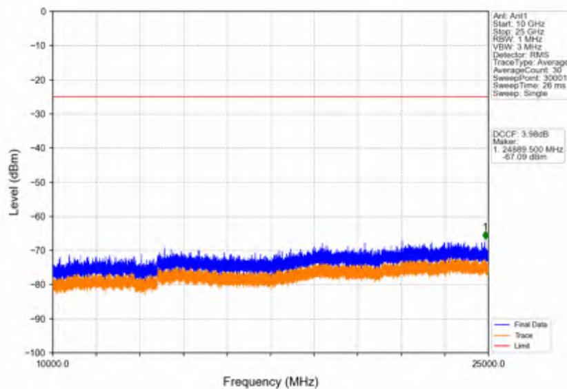
Band41_10MHz_256QAM_MCH_2593MHz_RB_1_0_NTNV
