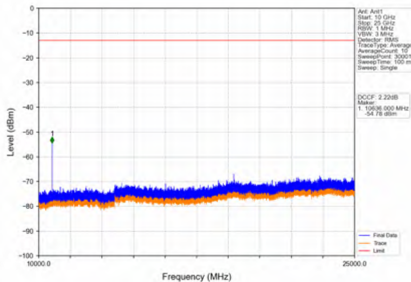
Band42a 5MHz_QPSK_HCH_3547.5MHz_RB_1_0_NTNV
