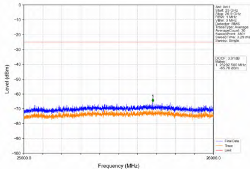
Band41_10MHz_64QAM_HCH_2685MHz_RB_1_49_NTNV
