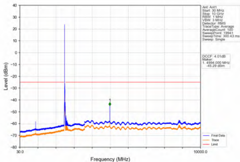
Band41_20MHz_QPSK_LCH_2506MHz_RB_1_0_NTNV
