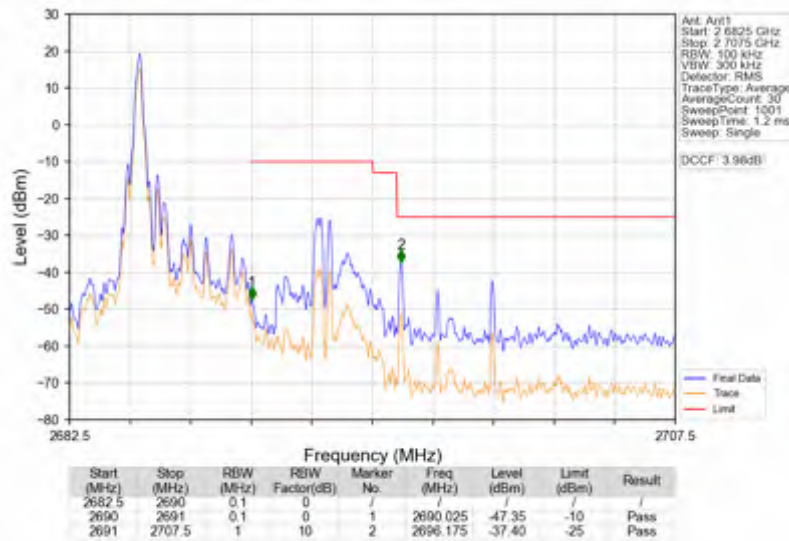
Band41_5MHz_QPSK_HCH_2687.5MHz_RB_25_0_NTNV
