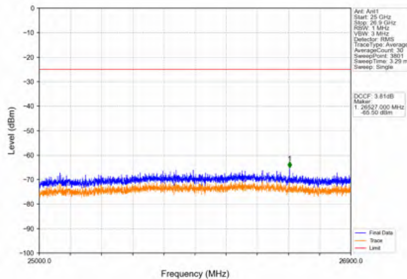
Band41_10MHz_16QAM_HCH_2685MHz_RB_1_0_NTV
