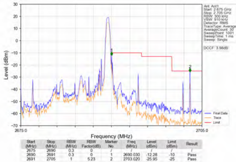
Band41_10MHz_256QAM_HCH_2685MHz_RB_1_49_NTNV
