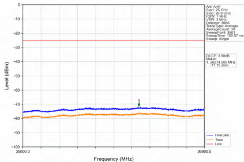
Band41_10MHz_16QAM_LCH_2501MHz_RB_50_0_NTNV
