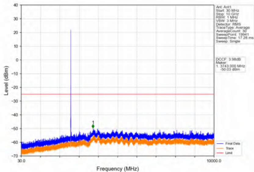
Band41_5MHz_256QAM_MCH_2593MHz_RB_1_0_NTNV
