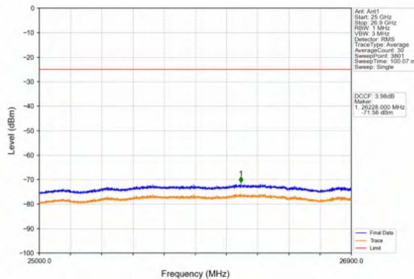
Band41_5MHz_QPSK_LCH_2498.5MHz_RB_1_0_NTNV
