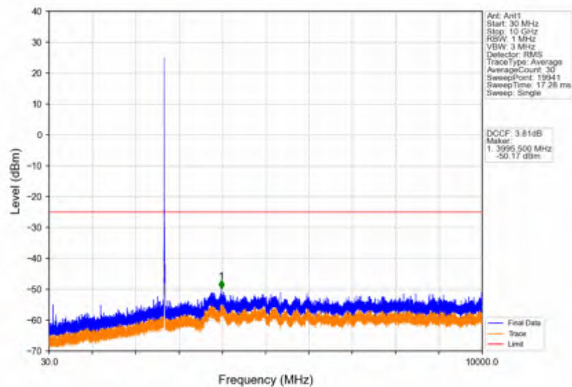
Band41_10MHz_16QAM_HCH_2685MHz_RB_1_0_NTNV
