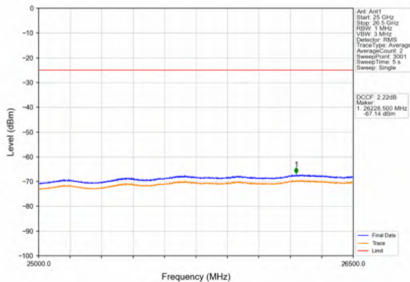
Band38_20MHz_16QAM_LCH_2580MHz_RB_100_0_NTNV
