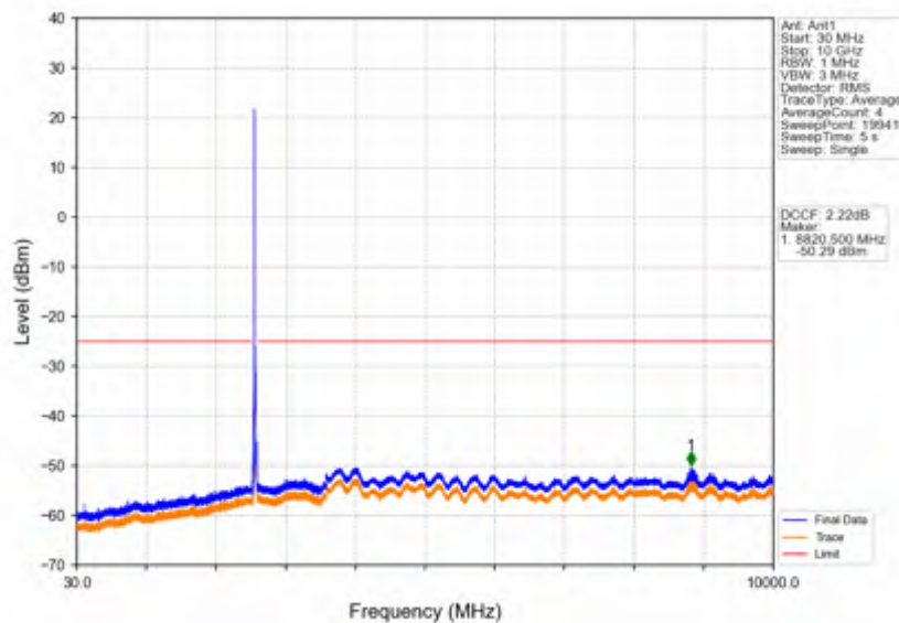
Band38 20MHz 64QAM LCH 2580MHz RB 1 0 NTNV
