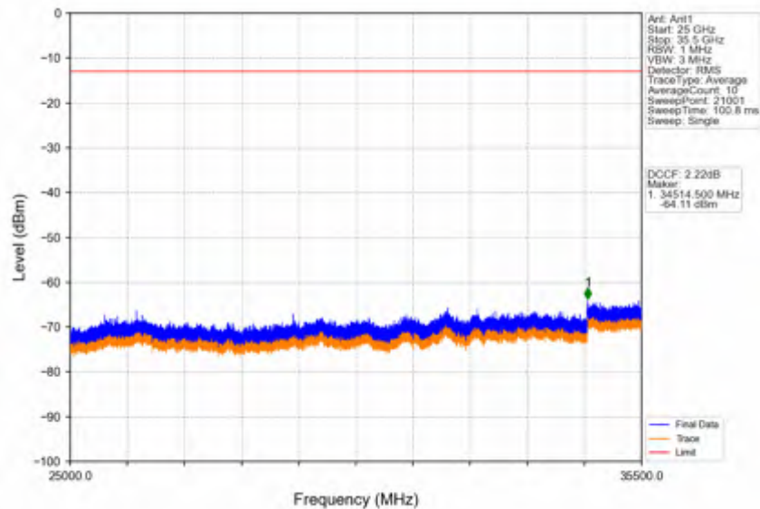
Band42a_10MHz_16QAM_LCH_3455MHz_RB_50_0_NTNV
