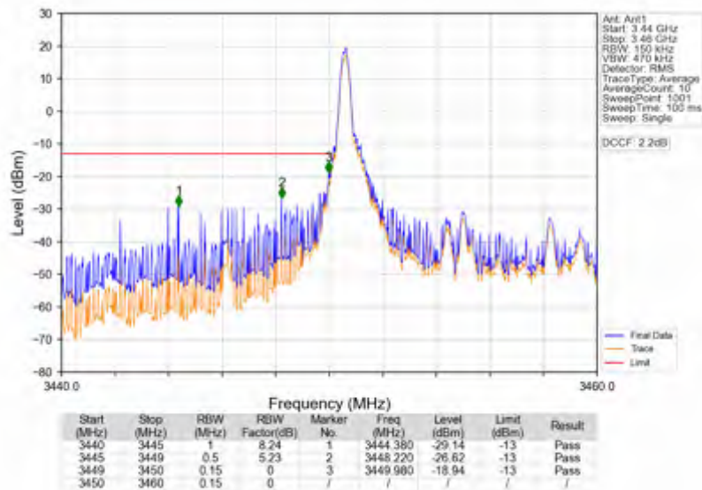
Band42a_10MHz_QPSK_LCH_3455MHz_RB_1_0_NTNV
