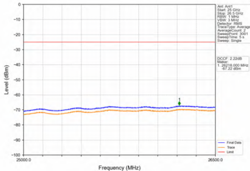
Band38_20MHz_64QAM_HCH_2610MHz_RB_1_99_NTNV
