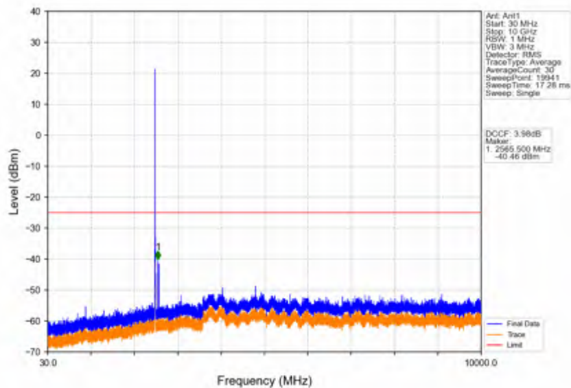
Band41_10MHz_256QAM_LCH_2501MHz_RB_1_0_NTNV
