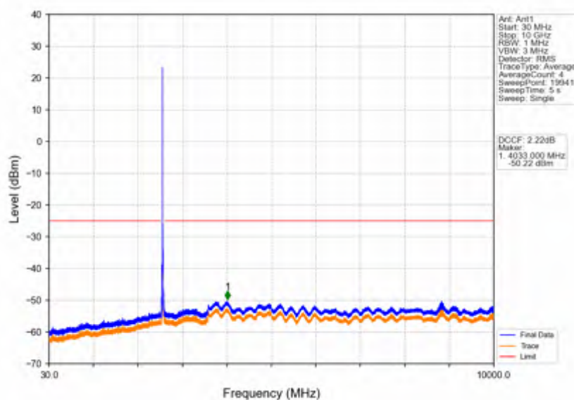
Band38_20MHz_QPSK_LCH_2580MHz_RB_1_0_NTNV
