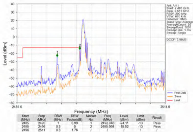
Band41_10MHz_256QAM_LCH_2501MHz_RB_1_0_NTNV
