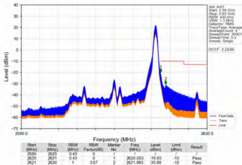
Band38_20MHz_256QAM_HCH_2610MHz_RB_1_99_NTNV
