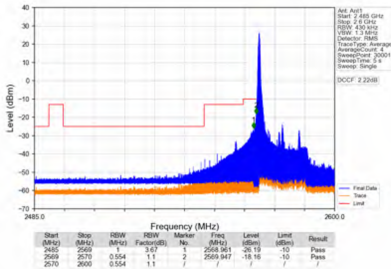
Band38_20MHz_QPSK_LCH_2580MHz_RB_1_0_NTNV
