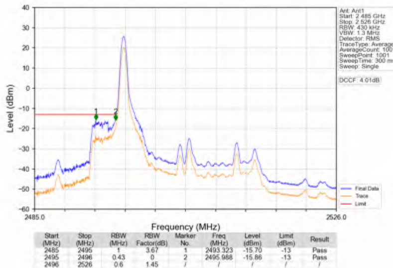
Band41_20MHz_QPSK_LCH_2506MHz_RB_1_0_NTNV
