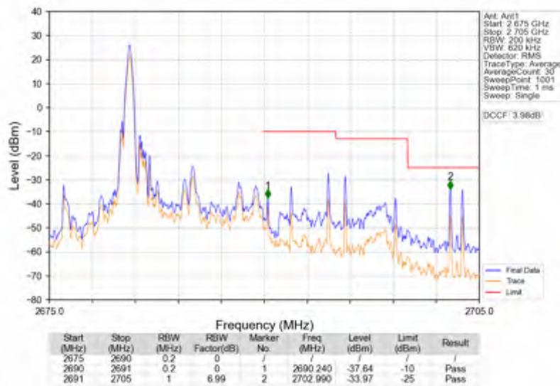
Band41_10MHz_16QAM_HCH_2685MHz_RB_50_0_NTNV
