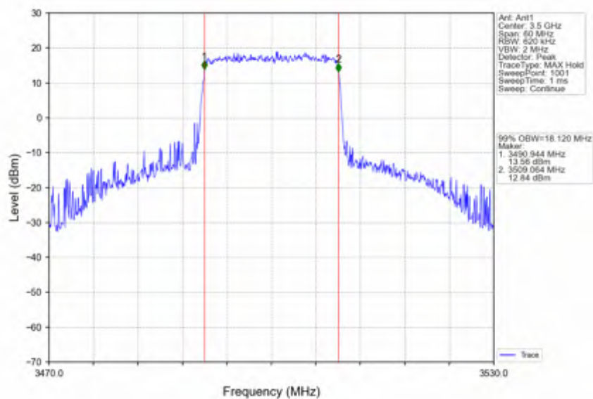
Band42a 20MHz 64QAM MCH 3500MHz RB 100 0 NTNV
