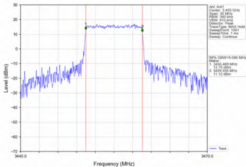
Band42a_10MHz_256QAM_LCH_3455MHz_RB_50_0_NTNV
