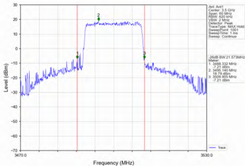
Band42a_20MHz_QPSK_MCH_3500MHz_RB_100_0_NTNV
