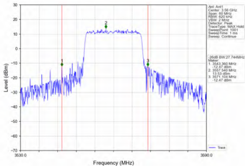
Band42c 20MHz 16QAM LCH 3560MHz RB 100 0 NTNV
