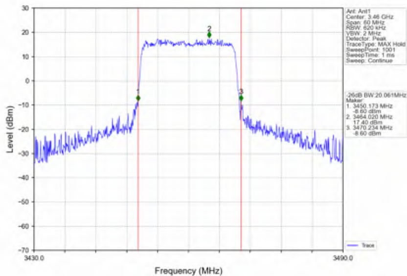
Band42a_20MHz_256QAM_LCH_3460MHz_RB_100_0_NTNV
