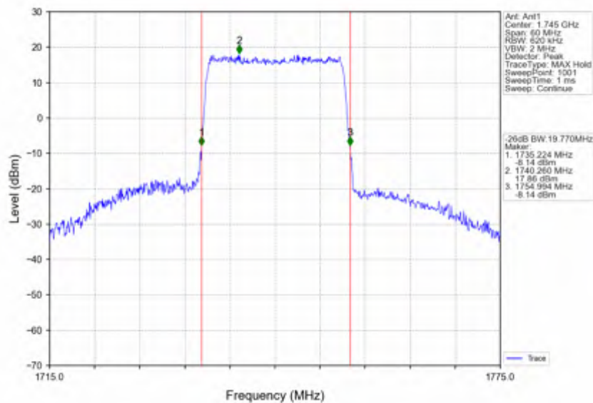
Band66_20MHz_QPSK_MCH_1745MHz_RB_100_0_NTNV
