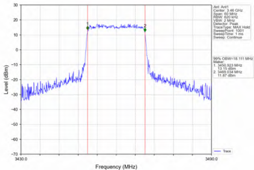
Band42a 20MHz 256QAM LCH 3460MHz RB 100 0 NTNV
