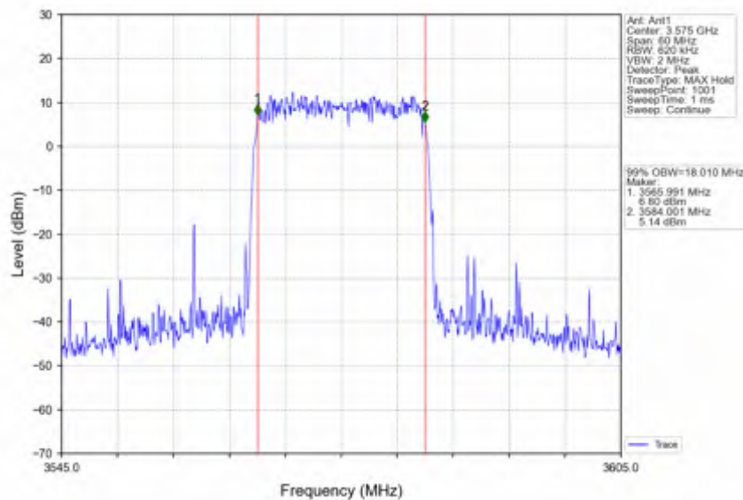
Band42c_20MHz_QPSK_MCH_3575MHz_RB_100_0_NTNV
