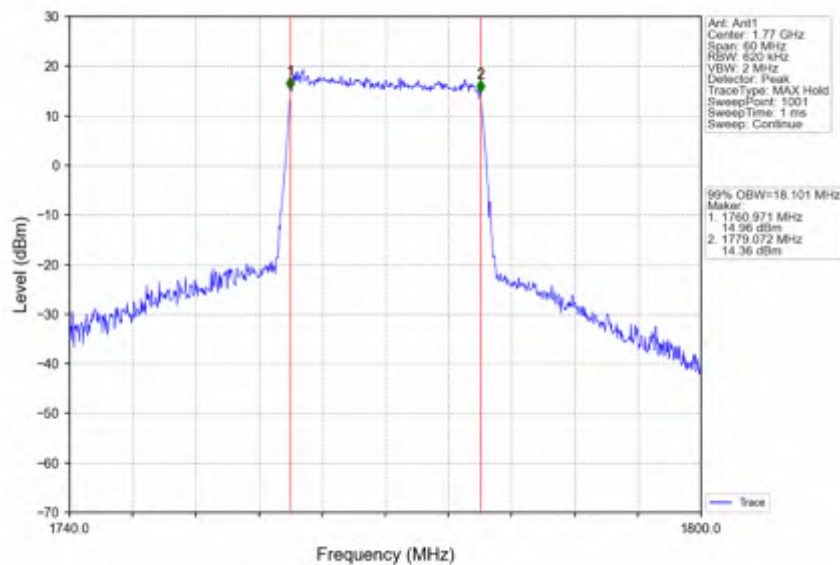
Band66 20MHz 16QAM HCH 1770MHz RB 100 0 NTNv
