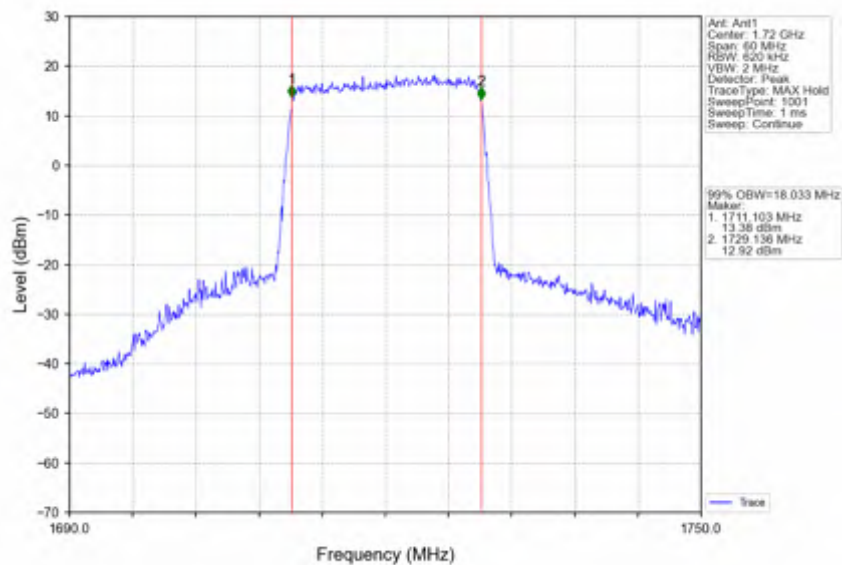
Band66 20MHz 16QAM LCH 1720MHz RB 100 0 NTN
