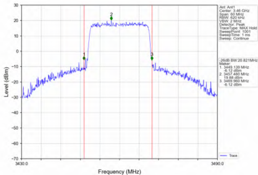
Band42a_20MHz_16QAM_LCH_3460MHz_RB_100_0_NTNV
