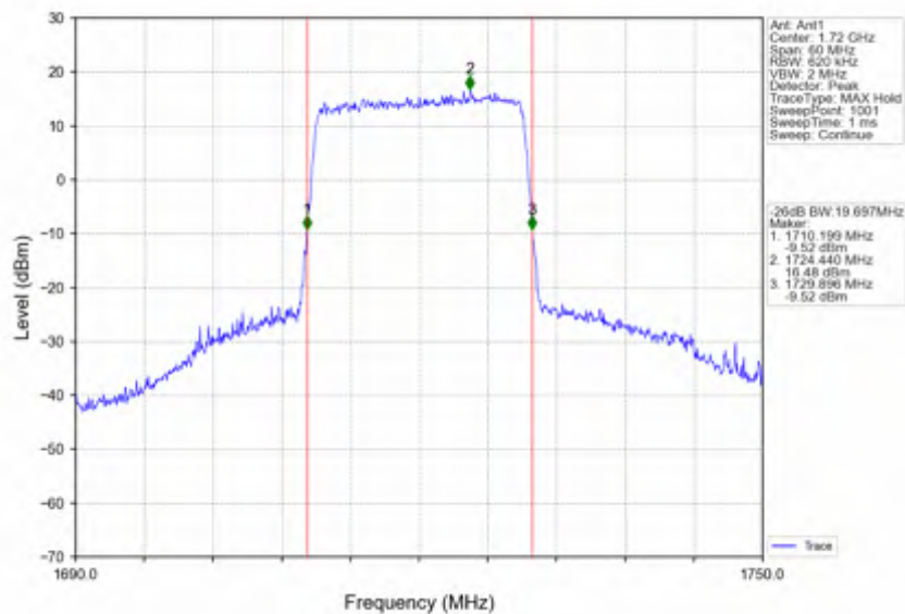
Band66_20MHz_256QAM_LCH_1720MHz_RB_100_0_NTNV
