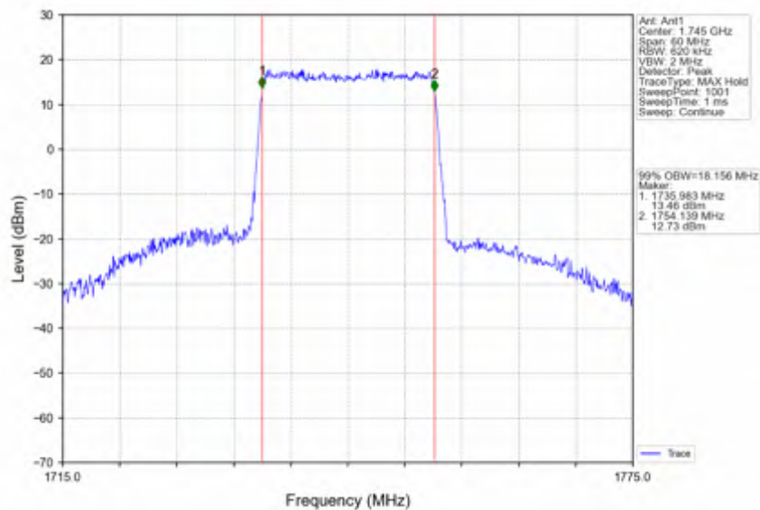
Band66_20MHz_QPSK_MCH_1745MHz_RB_100_0_NTNV
