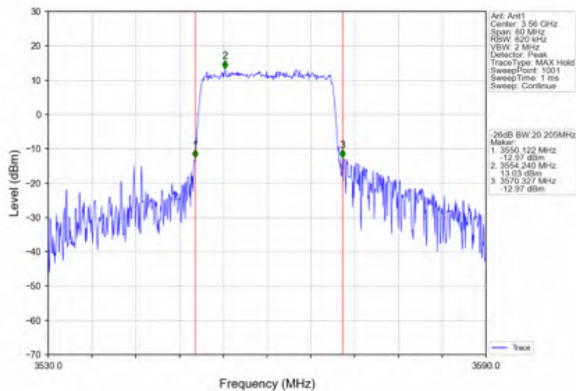
Band42c_20MHz_256QAM_LCH_3560MHz_RB_100_0_NTNV
