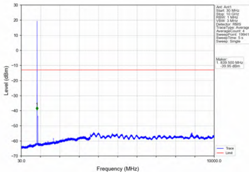
Band5_3MHz_QPSK_HCH_847.5MHz_RB_1_14_NTNV
