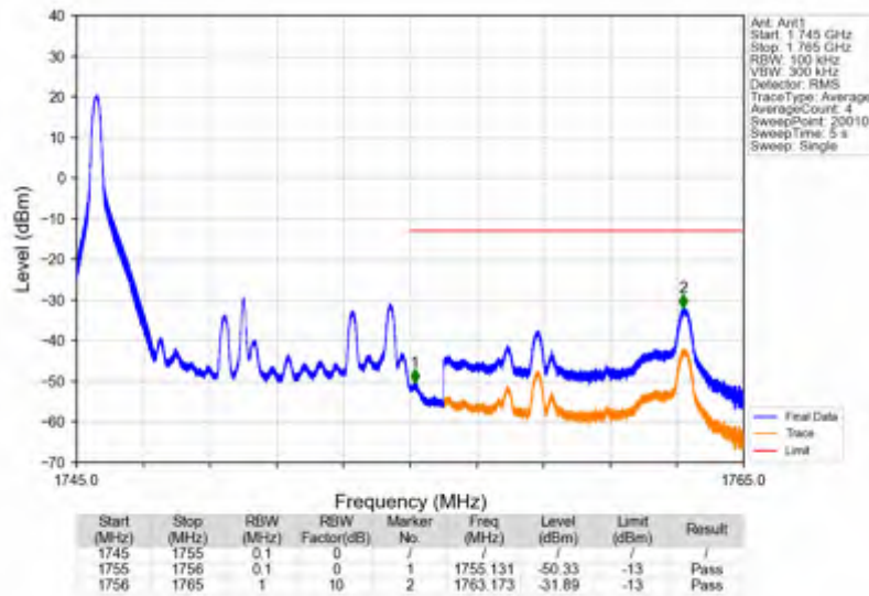
Band4_10MHz_QPSK_HCH_1750MHz_RB_1_49_NTNV
