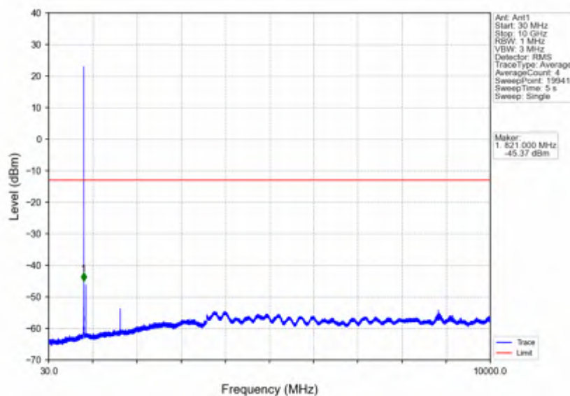
Band5 1.4MHz QPSK LCH 824.7MHz RB 1 0 NTNV
