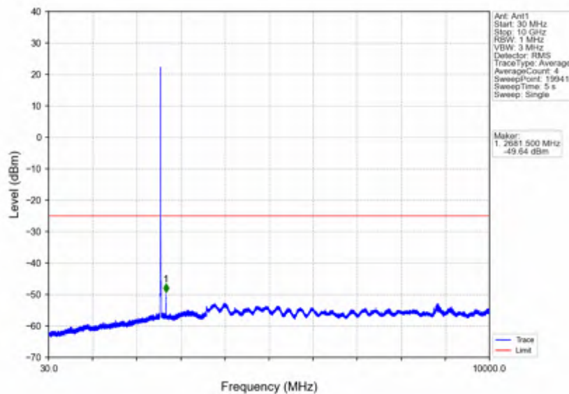
Band7_10MHz_QPSK_HCH_2565MHz_RB_1_0_NTNV
