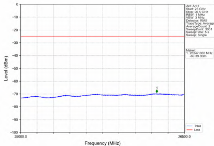
Band7_15MHz_QPSK_HCH_2562.5MHz_RB_1_74_NTNV
