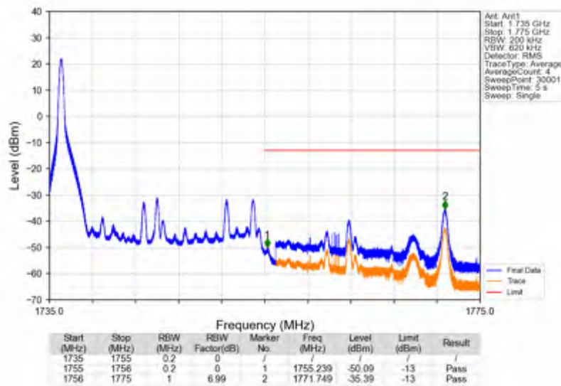
Band4_20MHz_QPSK_HCH_1745MHz_RB_100_0_NTNV
