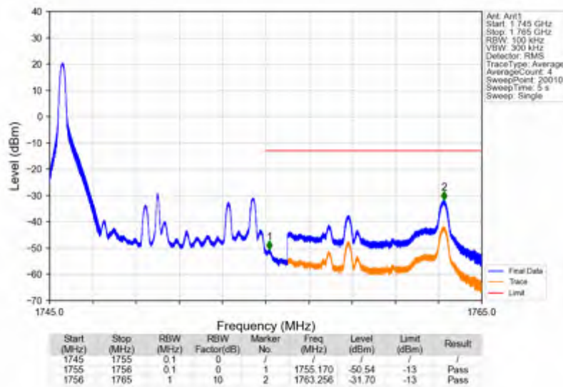
Band4_10MHz_QPSK_HCH_1750MHz_RB_50_0_NTNV
