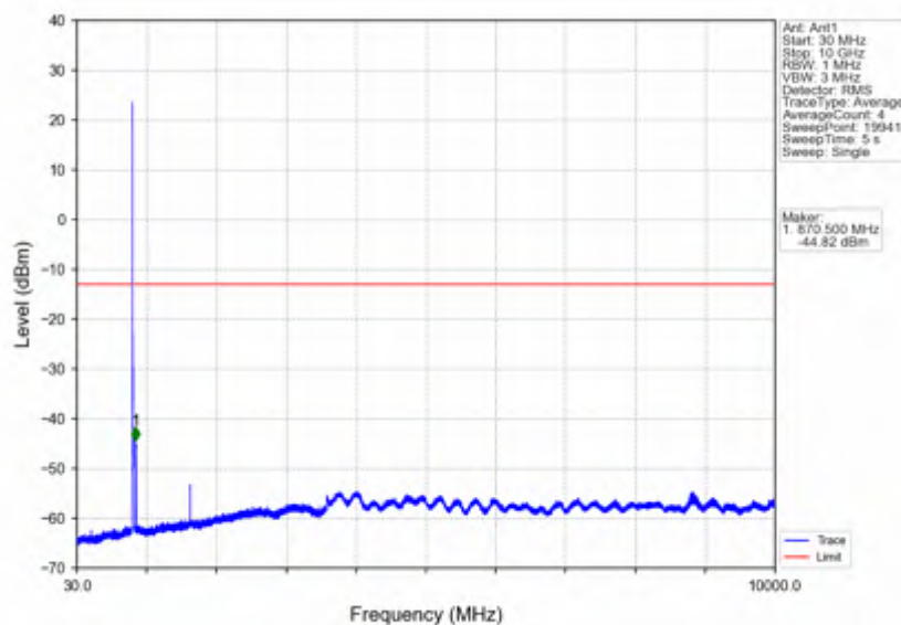
Band5 10MHz_QPSK_LCH_829MHz_RB_1_0_NTNV
