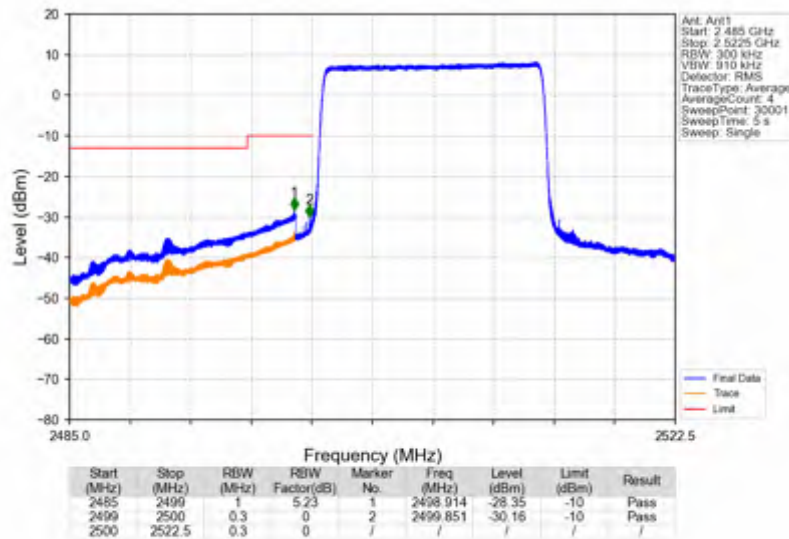
Band7 15MHz QPSK LCH 2507.5MHz RB 75 0 NTNV
