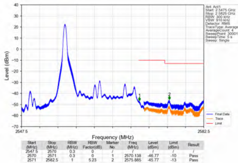
Band7_15MHz_QPSK_HCH_2562.5MHz_RB_1_74_NTNV
