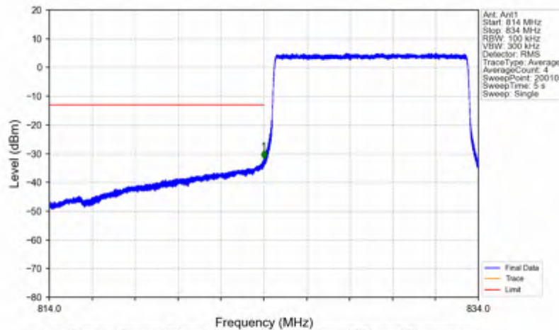
Band5_10MHz_QPSK_LCH_829MHz_RB_50_0_NTNV
