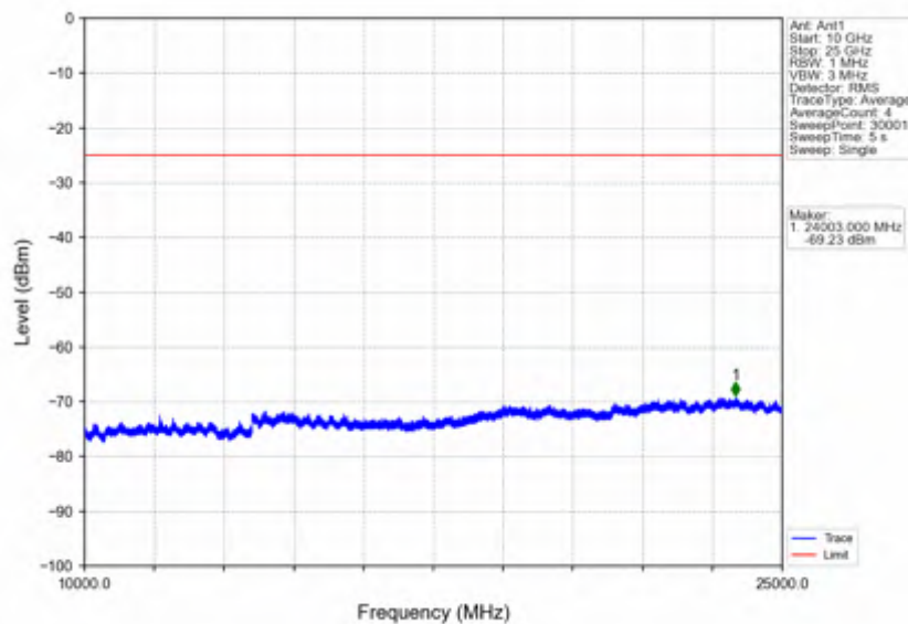
Band7_5MHz_QPSK_HCH_2567.5MHz_RB_1_0_NTNV
