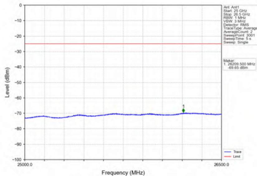
Band7_10MHz_QPSK_HCH_2565MHz_RB_1_49_NTNV
