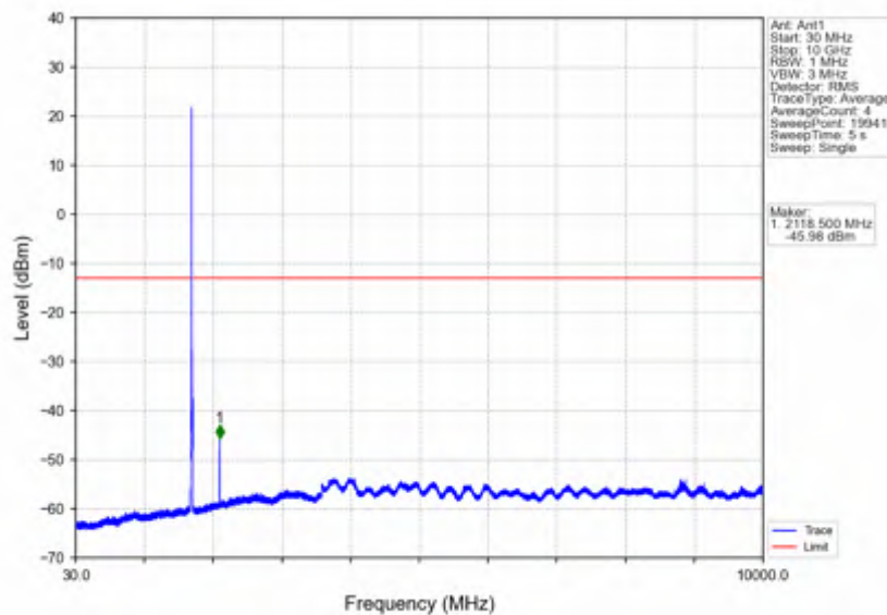
Band4 10MHz 64QAM LCH 1715MHz RB 1 0 NTNV
