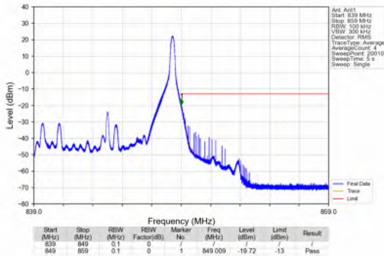
Band5_10MHz_QPSK_HCH_844MHz_RB_1_49_NTNV
