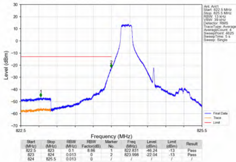
Band5 1.4MHz QPSK LCH 824.7MHz RB 1 0 NTNV
