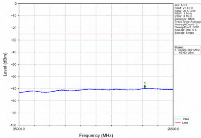
Band7_5MHz_QPSK_MCH_2535MHz_RB_1_0_NTNV
