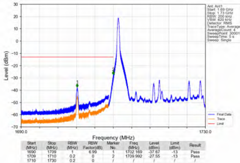
Band4 20MHz 256QAM LCH 1720MHz RB 1 0 NTNV
