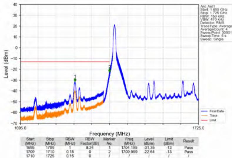
Band4_15MHz_QPSK_LCH_1717.5MHz_RB_1_0_NTNV
