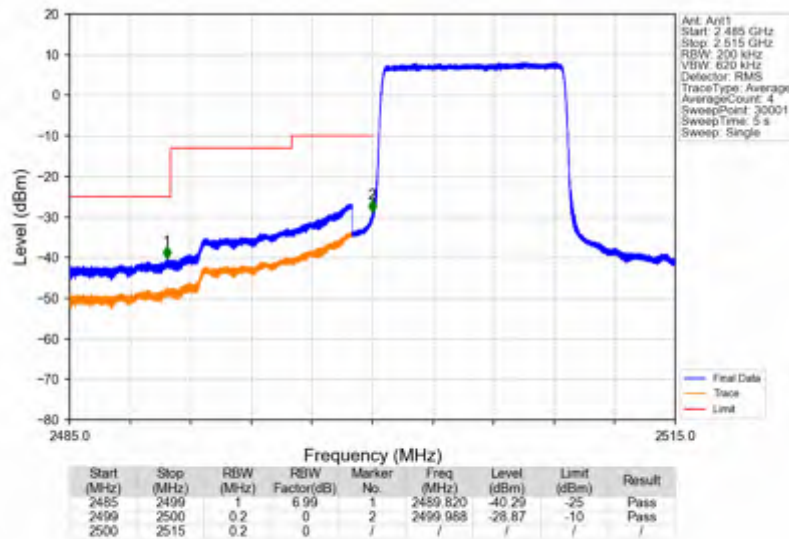
Band7 10MHz QPSK LCH 2505MHz RB 50 0 NTNV
