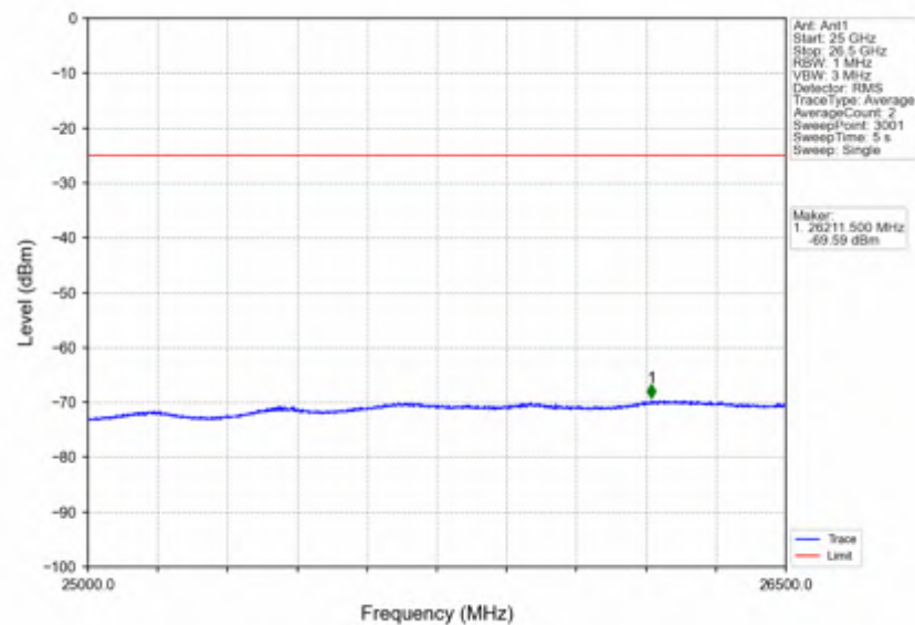
Band7 5MHz QPSK HCH 2567.5MHz RB 1 24 NTNV
