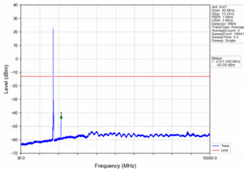
Band4_20MHz_QPSK_HCH_1745MHz_RB_1_0_NTNV
