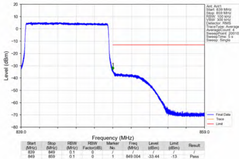
Band5_10MHz_QPSK_HCH_844MHz_RB_50_0_NTNV
