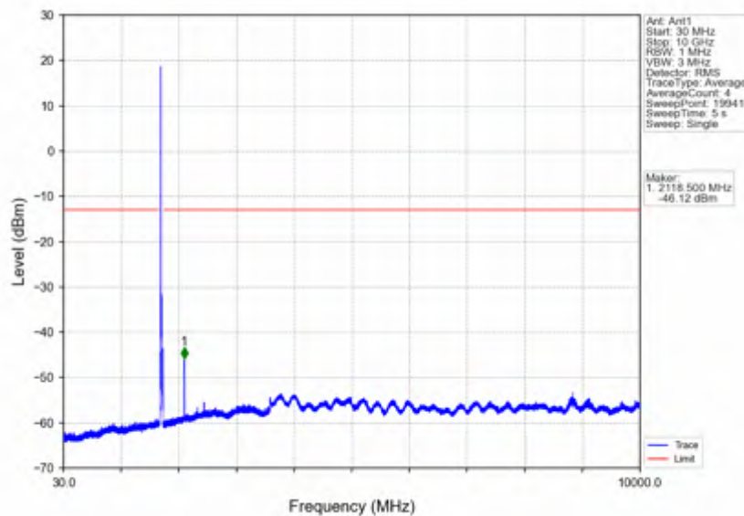
Band4 20MHz 256QAM LCH 1720MHz RB 1 0 NTNV
