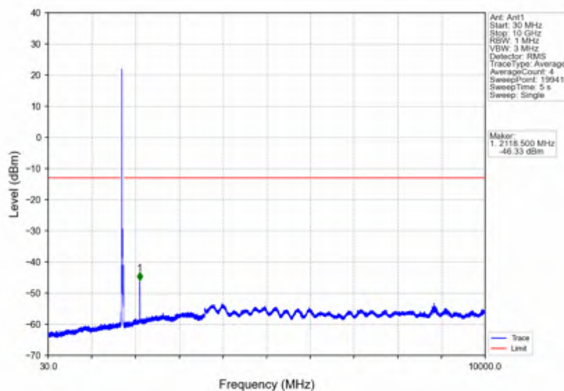
Band4_20MHz_QPSK_LCH_1720MHz_RB_1_0_NTNV
