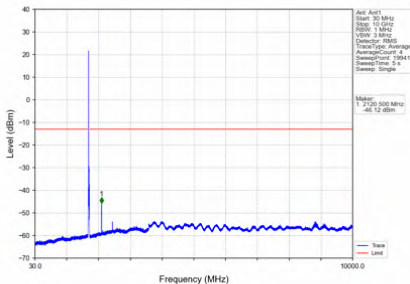
Band4_15MHz_QPSK_LCH_1717.5MHz_RB_1_0_NTNV
