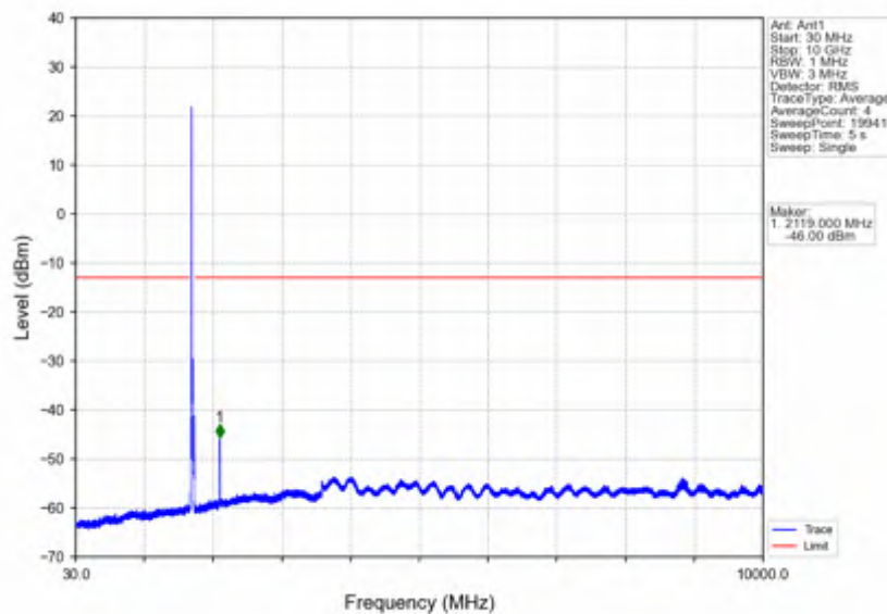
Band4_20MHz_16QAM_LCH_1720MHz_RB_1_0_NTNV
