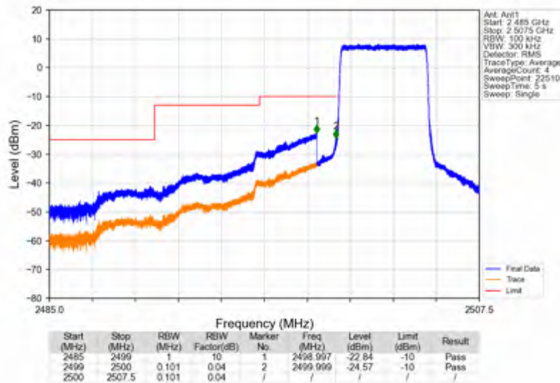
Band7_5MHz_QPSK_LCH_2502.5MHz_RB_25_0_NTNV
