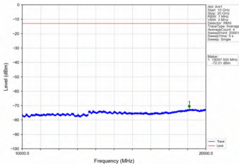
Band4_20MHz_QPSK_HCH_1745MHz_RB_1_0_NTNV
