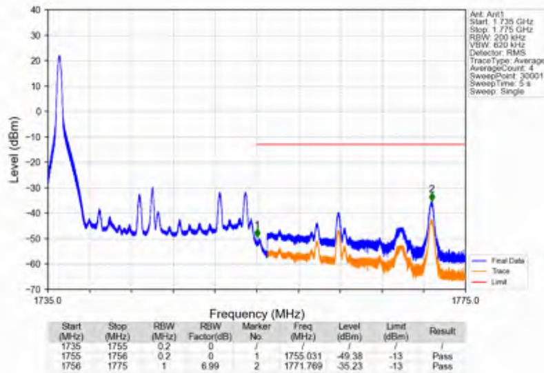
Band4_20MHz_QPSK_HCH_1745MHz_RB_1_99_NTNV
