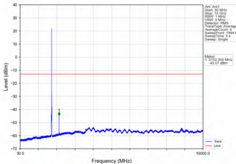
Band4_10MHz_QPSK_HCH_1750MHz_RB_1_0_NTNV
