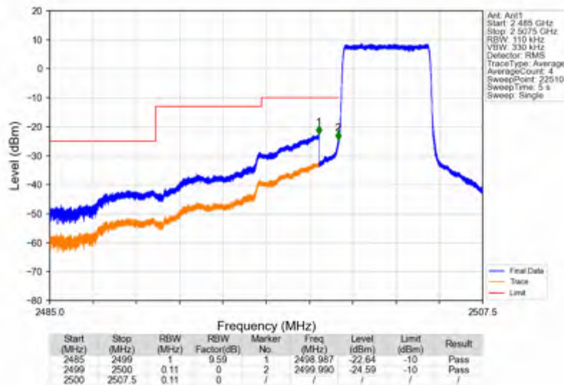
Band7_5MHz_QPSK_LCH_2502.5MHz_RB_1_0_NTNV
