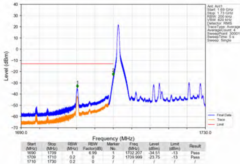
Band4_20MHz_16QAM_LCH_1720MHz_RB_1_0_NTNV
