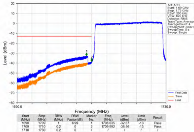
Band4_20MHz_256QAM_LCH_1720MHz_RB_100_0_NTNV
