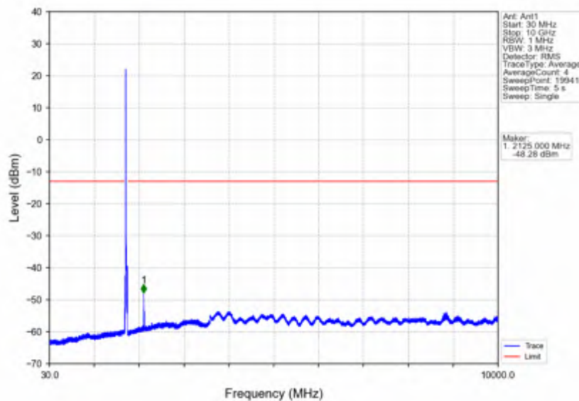
Band4 20MHz QPSK MCH 1732.5MHz RB 1 0 NTNV
