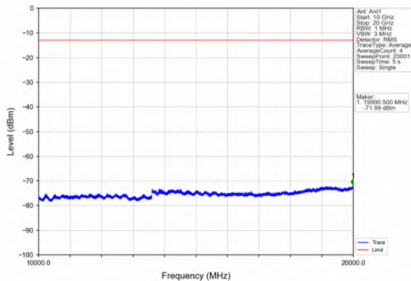
Band4_20MHz_QPSK_LCH_1720MHz_RB_100_0_NTNV
