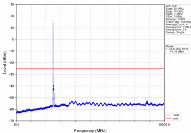
Band7_10MHz_QPSK_LCH_2505MHz_RB_1_0_NTNV
