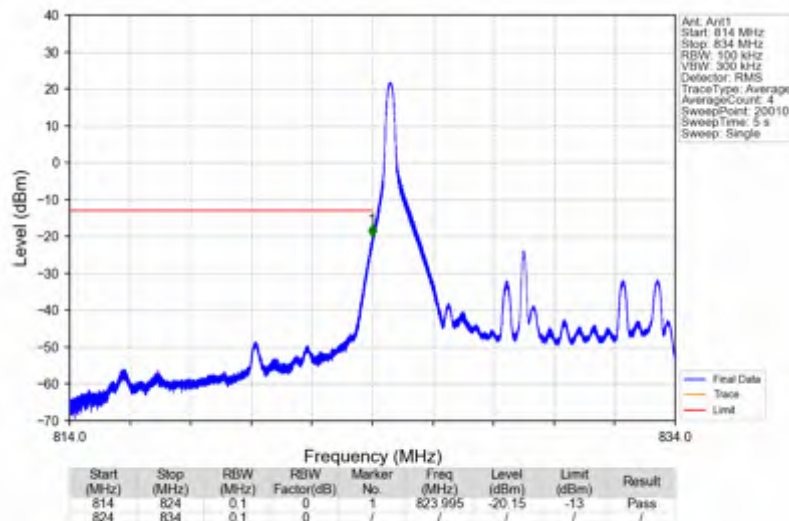
Band5 10MHz_QPSK_LCH_829MHz_RB_1_0_NTNV
