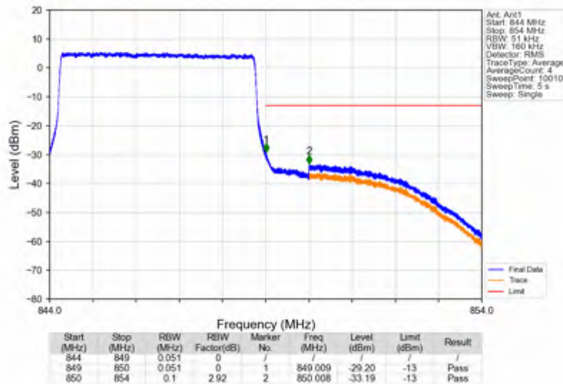
Band5_5MHz_QPSK_HCH_846.5MHz_RB_1_24_NTNV
