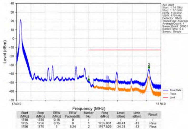
Band4_15MHz_QPSK_HCH_1747.5MHz_RB_1_74_NTNV
