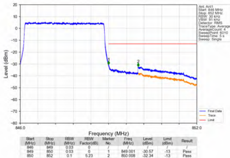
Band5_3MHz_QPSK_HCH_847.5MHz_RB_1_14_NTNV
