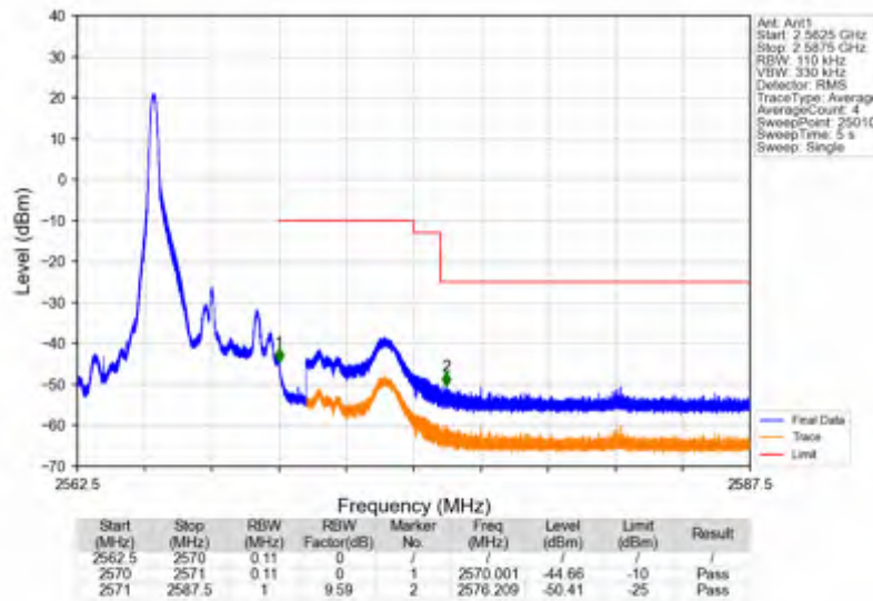
Band7_5MHz_QPSK_HCH_2567.5MHz_RB_25_0_NTNV
