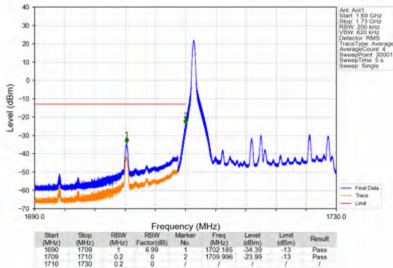
Band4_20MHz_QPSK_LCH_1720MHz_RB_100_0_NTNV
