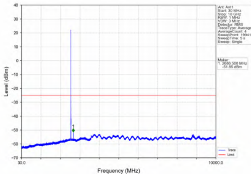
Band7_5MHz_QPSK_HCH_2567.5MHz_RB_1_0_NTNV
