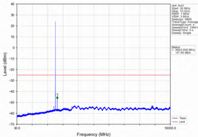
Band7_5MHz_QPSK_MCH_2535MHz_RB_1_0_NTNV
