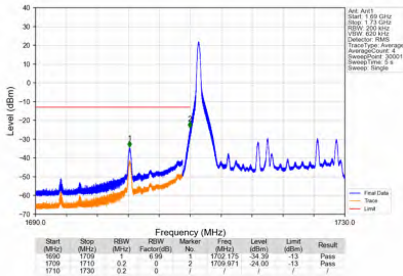
Band4_20MHz_QPSK_LCH_1720MHz_RB_1_0_NTNV
