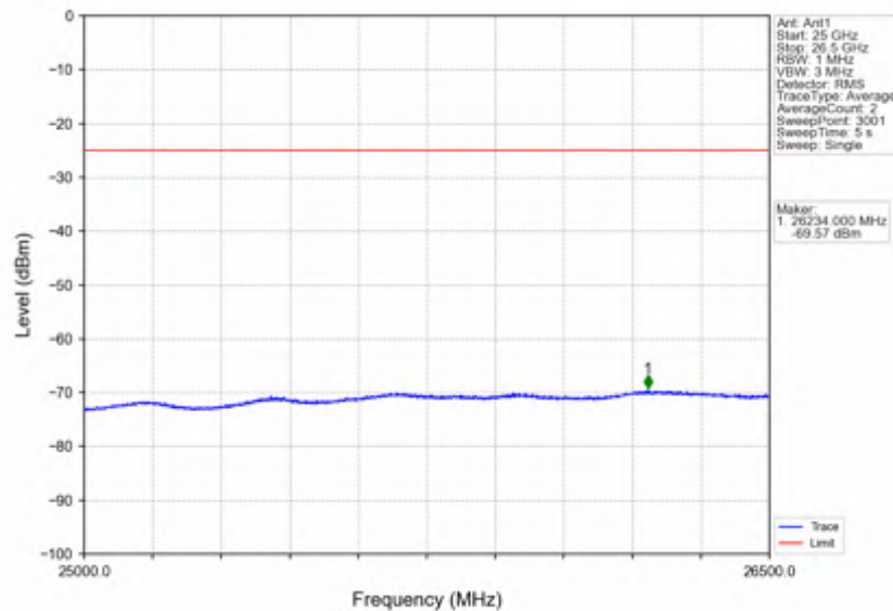
Band7_10MHz_QPSK_LCH_2505MHz_RB_1_0_NTNV
