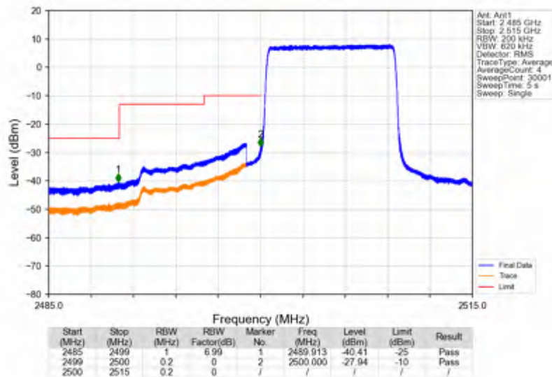
Band7_10MHz_QPSK_LCH_2505MHz_RB_1_0_NTNV
