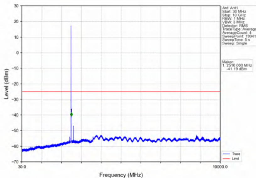
Band7_5MHz_QPSK_LCH_2502.5MHz_RB_1_0_NTNV
