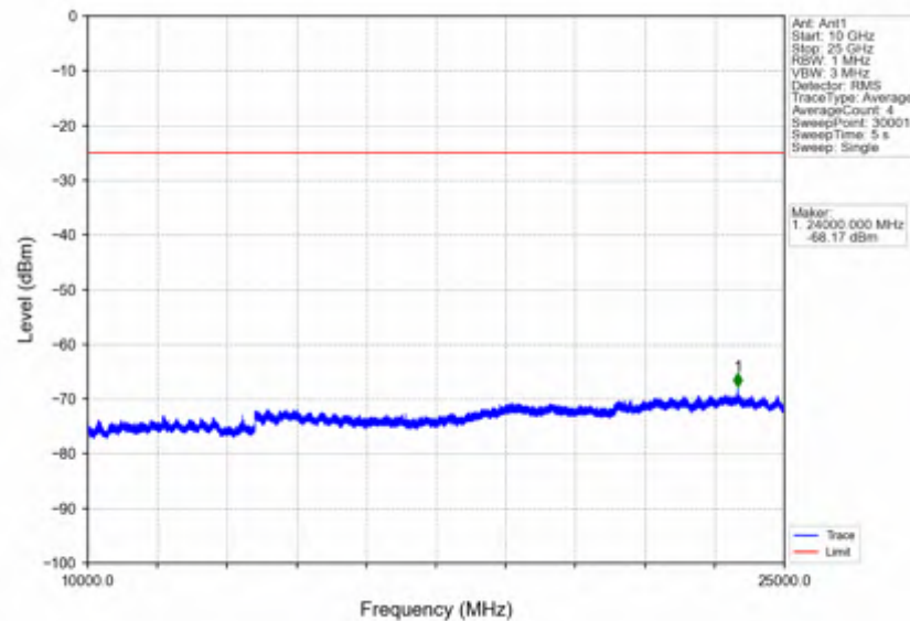
Band7_10MHz_QPSK_MCH_2535MHz_RB_1_0_NTNV
