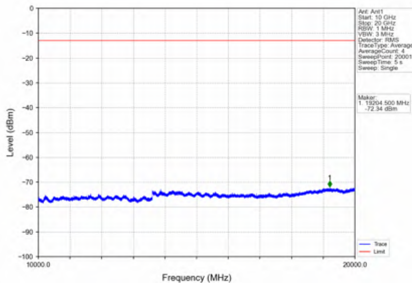
Band4_10MHz_QPSK_HCH_1750MHz_RB_1_0_NTNV
