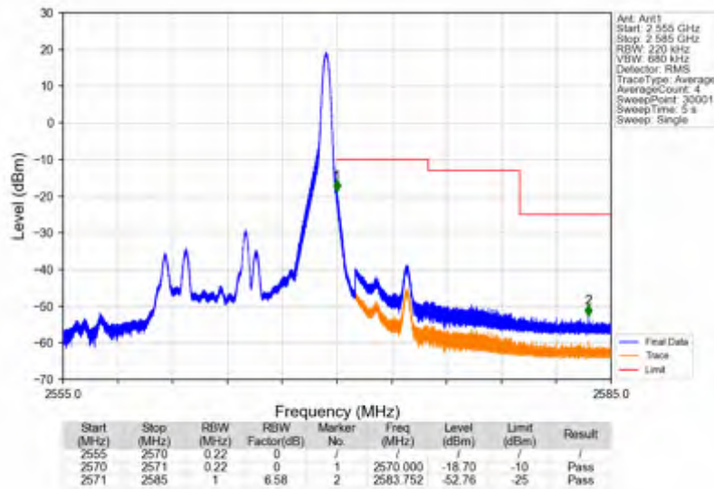
Band7_10MHz_256QAM_HCH_2565MHz_RB_1_49_NTNV
