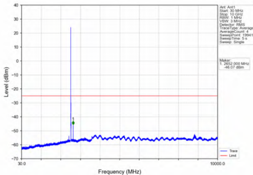
Band7_10MHz_QPSK_MCH_2535MHz_RB_1_0_NTNV
