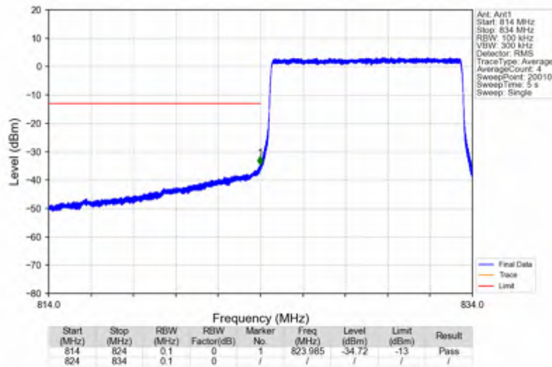
Band5 10MHz 64QAM LCH 829MHz RB 50 0 NTNV
