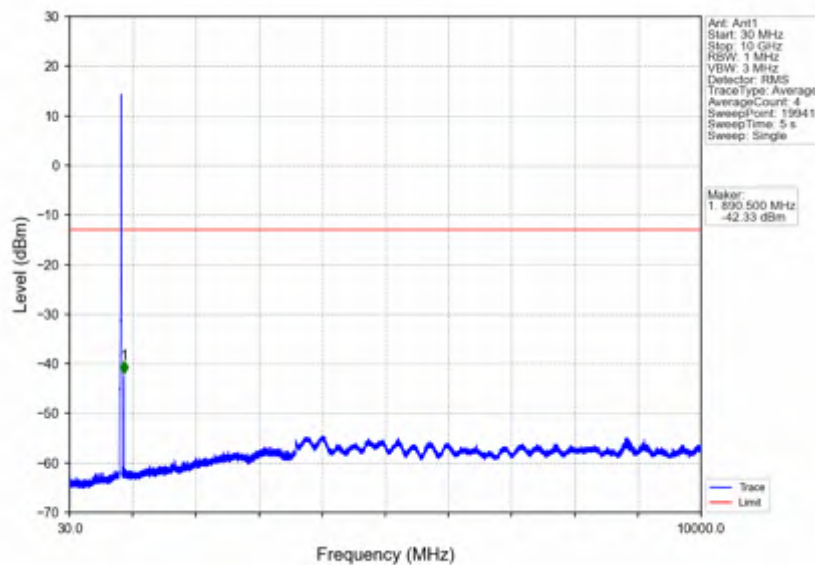
Band5_10MHz_QPSK_HCH_844MHz_RB_1_49_NTNV
