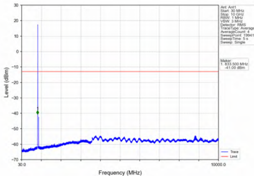
Band5_5MHz_QPSK_HCH_846.5MHz_RB_1_24_NTNV
