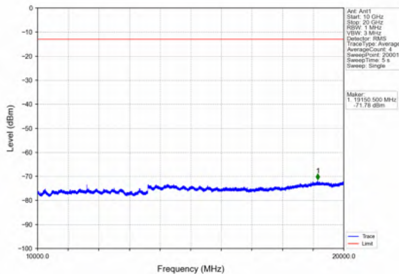
Band4 20MHz 16QAM LCH 1720MHz RB 100 0 NTNV
