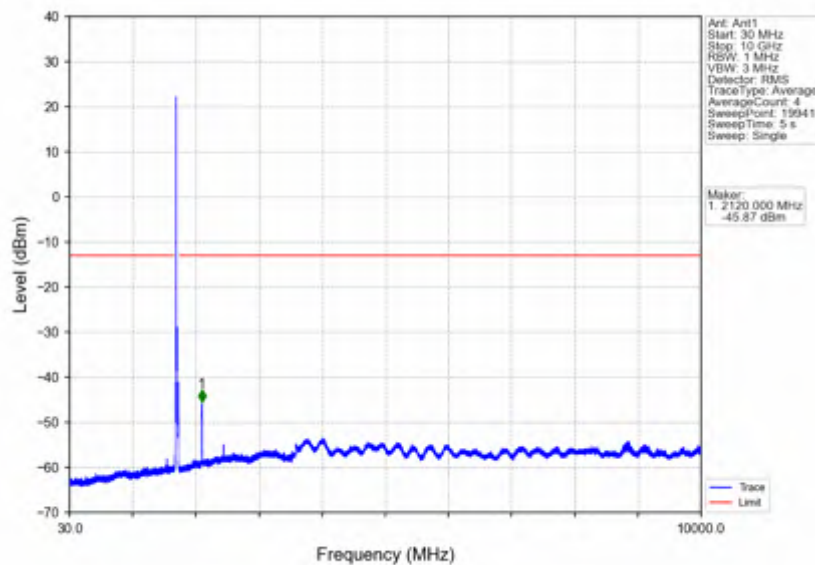
Band4 20MHz 64QAM LCH 1720MHz RB 1 0 NTNV
