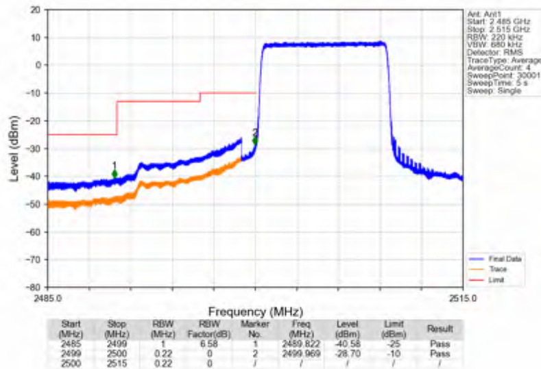
Band7 10MHz 64QAM LCH 2505MHz RB 50 0 NTNV
