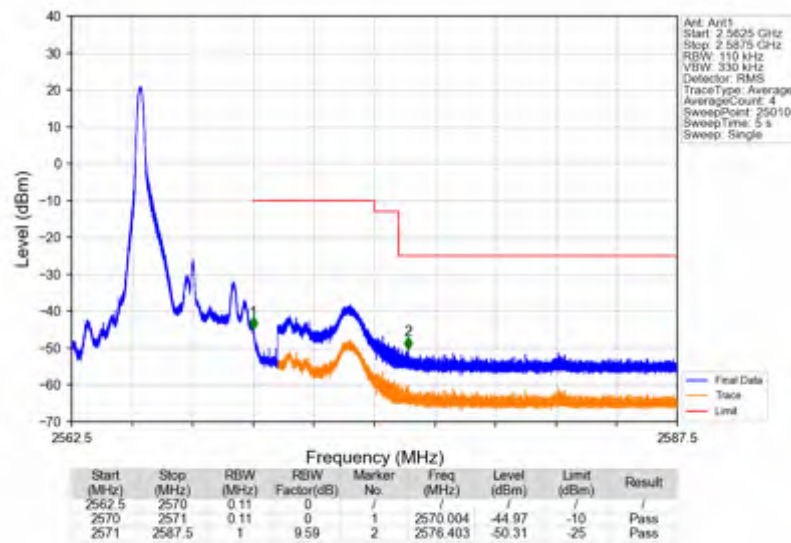
Band7 5MHz QPSK HCH 2567.5MHz RB 1 24 NTNV
