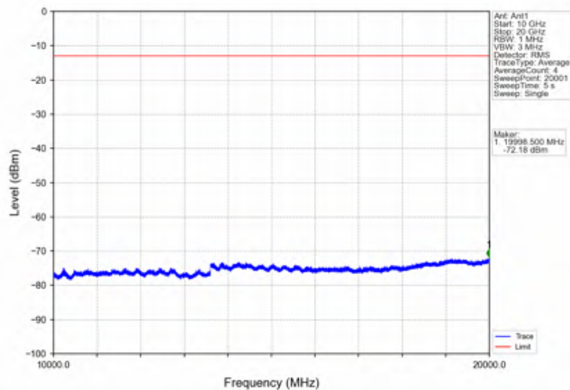
Band4_20MHz_256QAM_LCH_1720MHz_RB_100_0_NTNV
