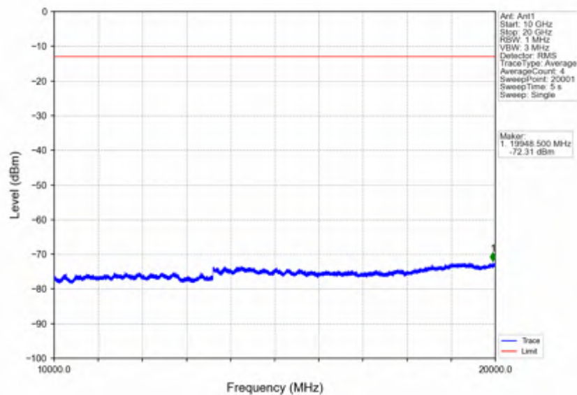
Band2_20MHz_256QAM_LCH_1860MHz_RB_100_0_NTNV
