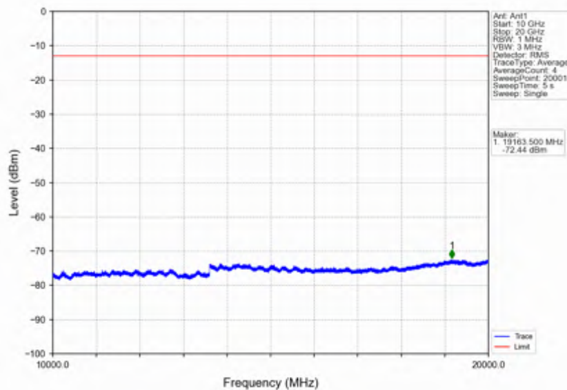
Band2_3MHz_16QAM_MCH_1880MHz_RB_1_0_NTNV
