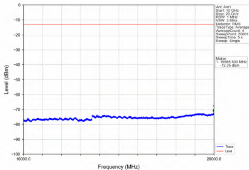
Band2_10MHz_16QAM_LCH_1855MHz_RB_50_0_NTNV
