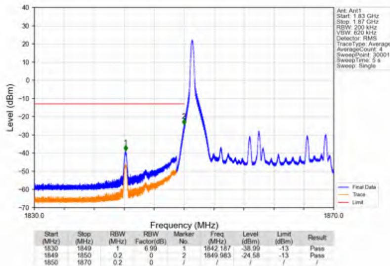
Band2_20MHz_QPSK_LCH_1860MHz_RB_1_0_NTNV
