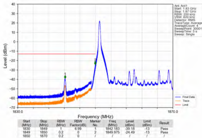
Band2_20MHz_64QAM_LCH_1860MHz_RB_100_0_NTNV
