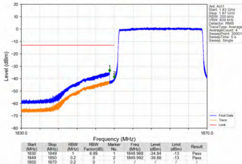
Band2_20MHz_256QAM_LCH_1860MHz_RB_100_0_NTNV
