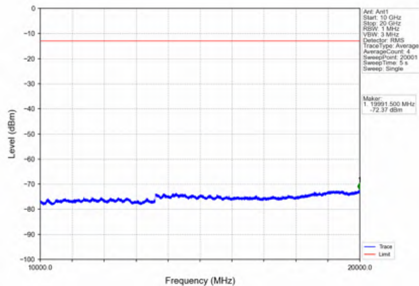
Band2_10MHz_256QAM_LCH_1855MHz_RB_50_0_NTNV
