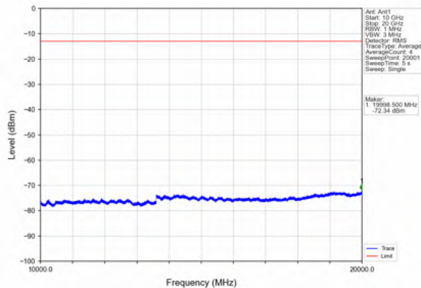
Band2_10MHz_64QAM_LCH_1855MHz_RB_50_0_NTNV
