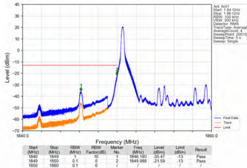
Band2_10MHz_64QAM_LCH_1855MHz_RB_50_0_NTNV
