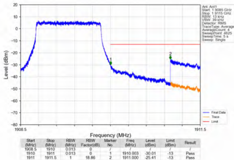
Band2_1.4MHz_QPSK_HCH_1909.3MHz_RB_1_5_NTV
