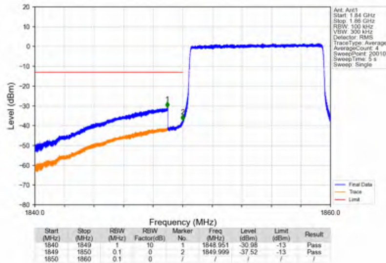
Band2_10MHz_256QAM_LCH_1855MHz_RB_50_0_NTNV
