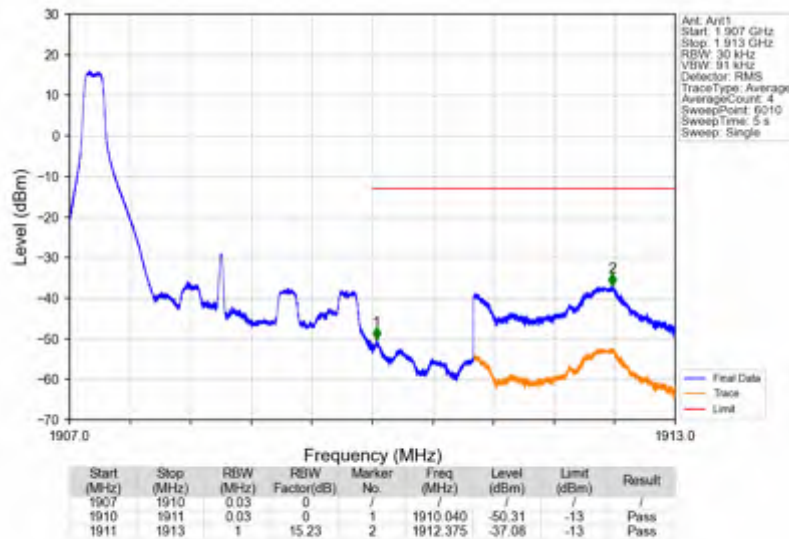
Band2_3MHz_QPSK_HCH_1908.5MHz_RB_1_14_NTNV
