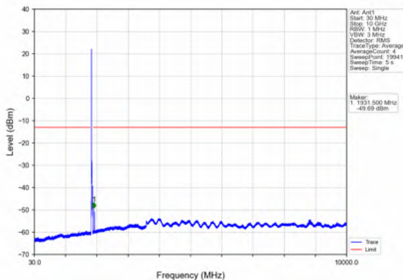
Band2_20MHz_QPSK_LCH_1860MHz_RB_1_0_NTNV
