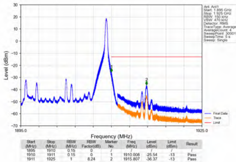
Band2_15MHz_256QAM_HCH_1902.5MHz_RB_1_74_NTNV
