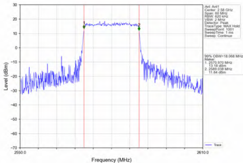
Band38 20MHz 16QAM LCH 2580MHz RB 100 0 NTNv
