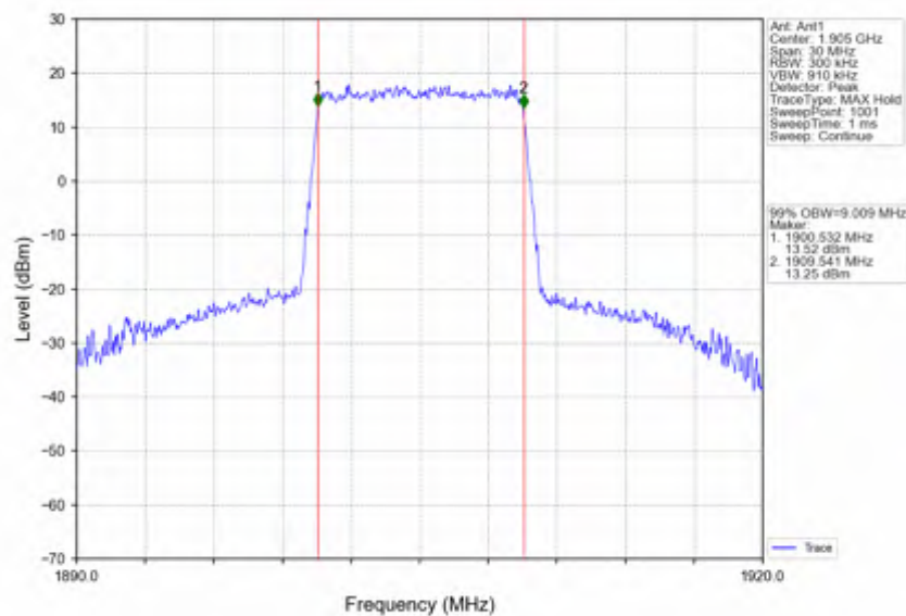
Band2_10MHz_16QAM_HCH_1905MHz_RB_50_0_NTNV
