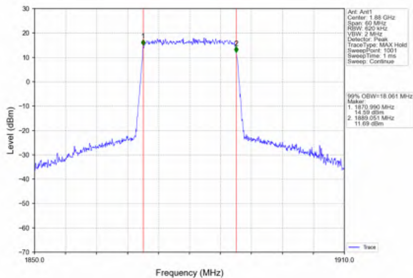
Band2_20MHz_64QAM_MCH_1880MHz_RB_100_0_NTNV
