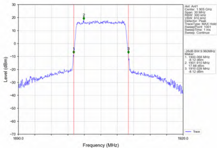
Band2_10MHz_16QAM_HCH_1905MHz_RB_50_0_NTNV
