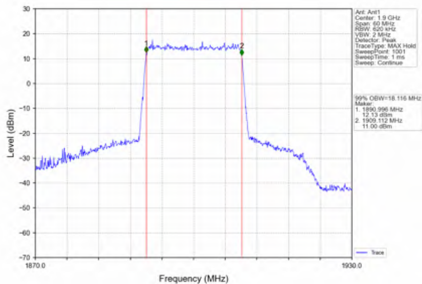
Band2_20MHz_256QAM_HCH_1900MHz_RB_100_0_NTNV
