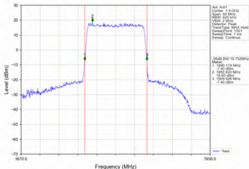
Band2_20MHz_16QAM_HCH_1900MHz_RB_100_0_NTNV
