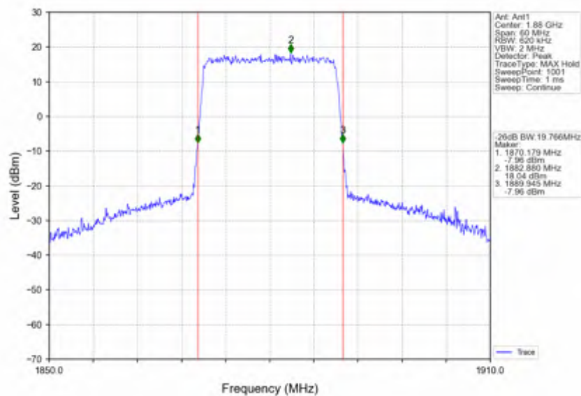
Band2_20MHz_64QAM_MCH_1880MHz_RB_100_0_NTNV
