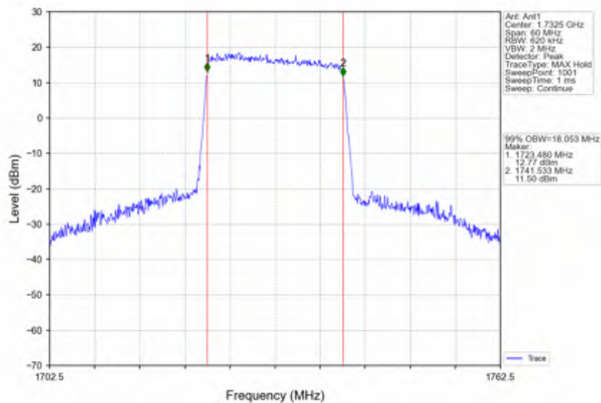
Band4_20MHz_QPSK_MCH_1732.5MHz_RB_100_0_NTNV
