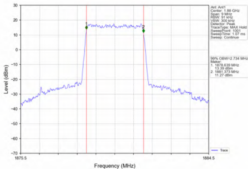
Band2_3MHz_QPSK_MCH_1880MHz_RB_15_0_NTNV
