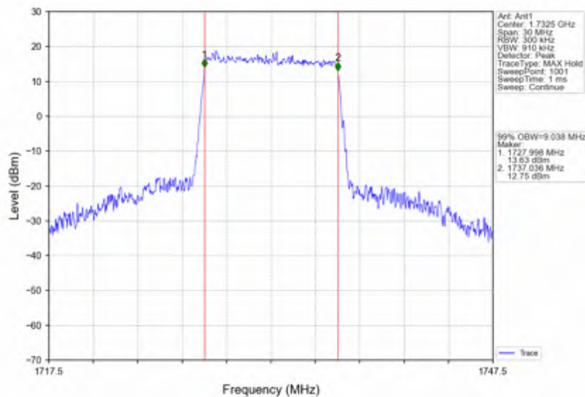
Band4 10MHz QPSK MCH 1732.5MHz RB 50 0 NTNV
