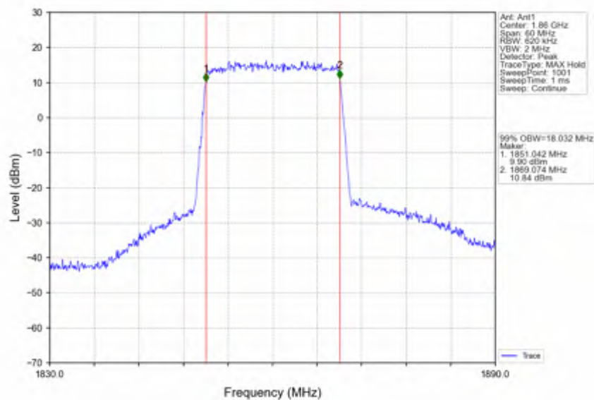
Band2_20MHz_256QAM_LCH_1860MHz_RB_100_0_NTNV
