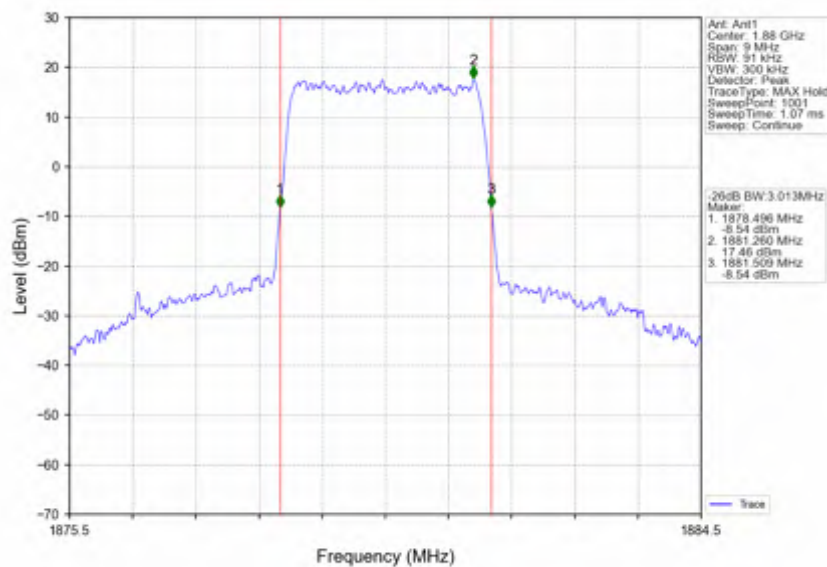
Band2_3MHz_QPSK_MCH_1880MHz_RB_15_0_NTNV
