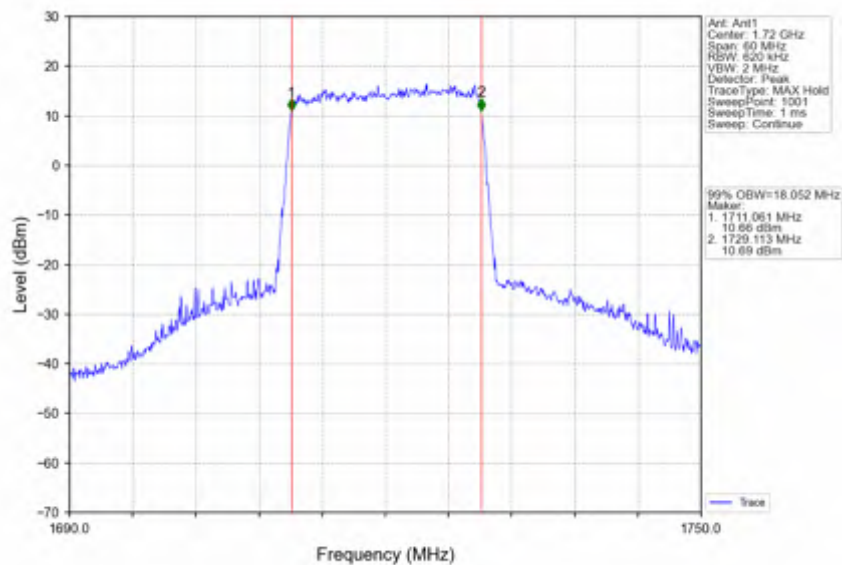
Band4 20MHz 256QAM LCH 1720MHz RB 100 0 NTN
