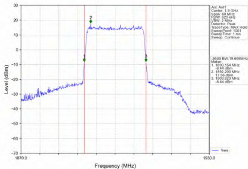
Band2_20MHz_256QAM_HCH_1900MHz_RB_100_0_NTNV
