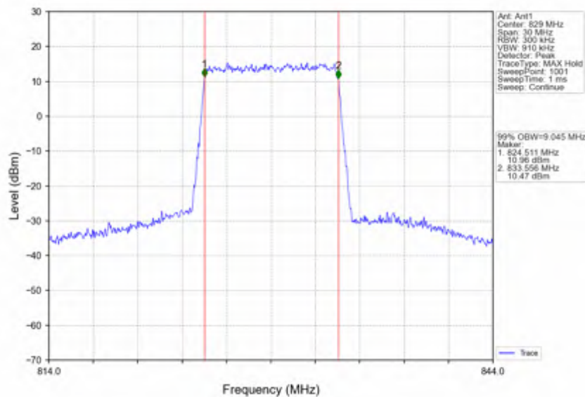
Band5 10MHz 256QAM LCH 829MHz RB 50 0 NTNV
