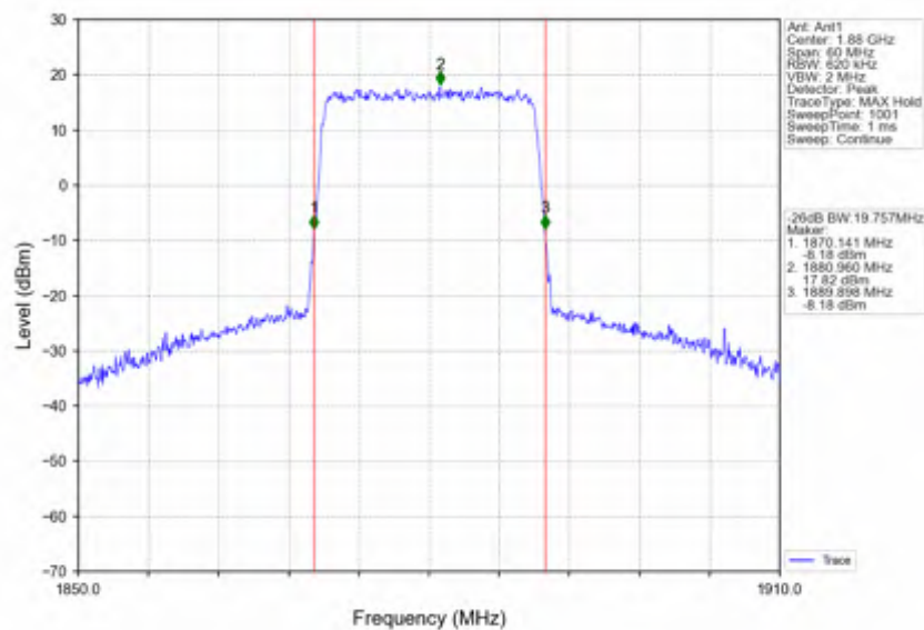
Band2_20MHz_QPSK_MCH_1880MHz_RB_100_0_NTNV
