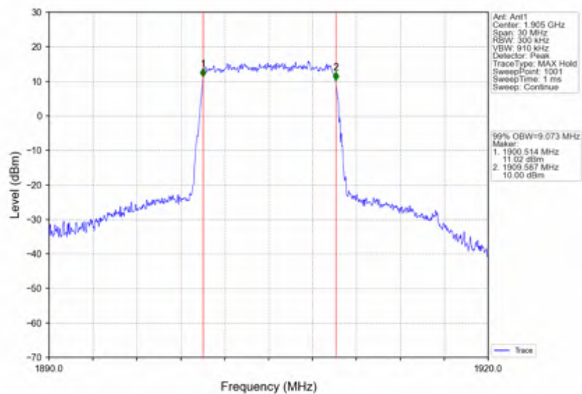
Band2_10MHz_256QAM_HCH_1905MHz_RB_50_0_NTNV
