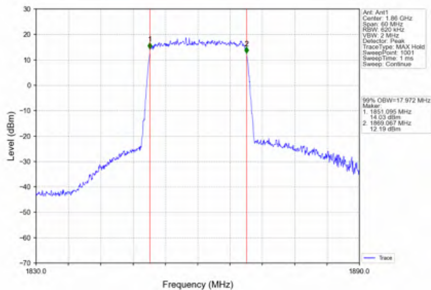
Band2 20MHz 16QAM LCH 1860MHz RB 100 0 NTN
