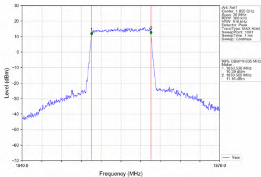
Band2_10MHz_256QAM_LCH_1855MHz_RB_50_0_NTNV
