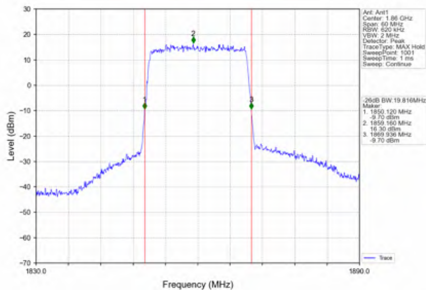
Band2_20MHz_256QAM_LCH_1860MHz_RB_100_0_NTNV
