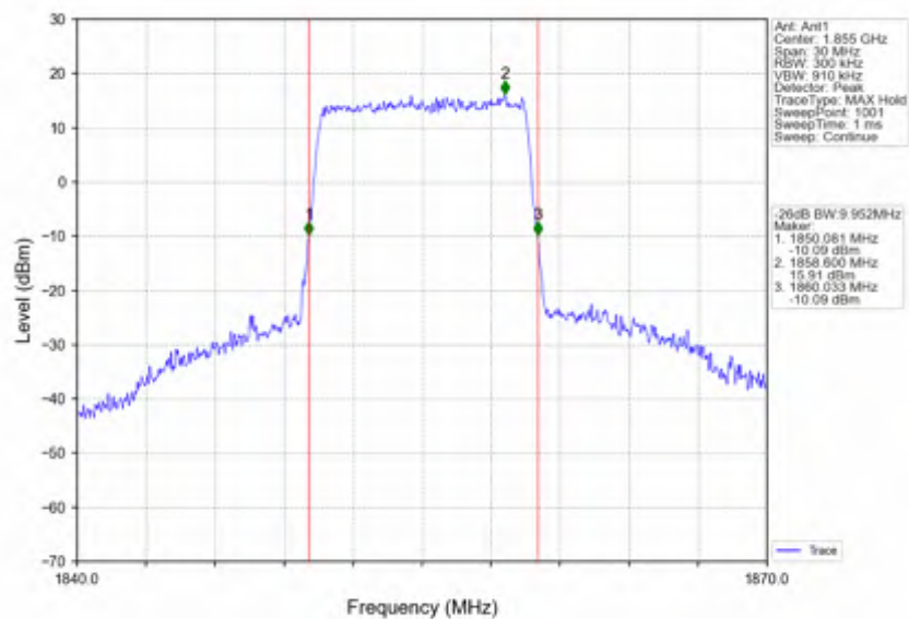
Band2_10MHz_256QAM_LCH_1855MHz_RB_50_0_NTNV
