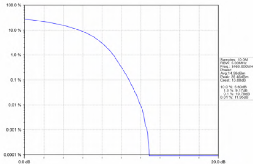
Band42a_20MHz_16QAM_LCH_3460MHz_RB_100_0_NTNV
