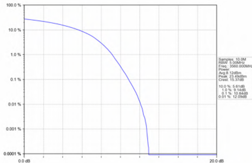
Band42c_20MHz_16QAM_LCH_3560MHz_RB_100_0_NTNV
