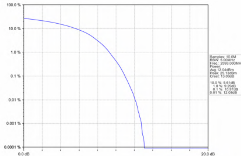
Band41_20MHz_256QAM_MCH_2593MHz_RB_100_0_NTNV
