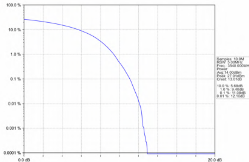
Band42a_20MHz_QPSK_HCH_3540MHz_RB_100_0_NTNV
