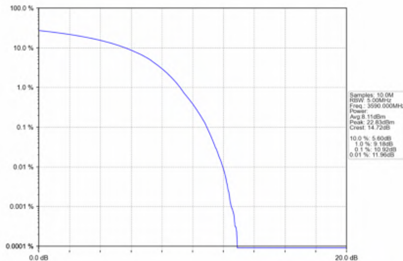
Band42c_20MHz_QPSK_HCH_3590MHz_RB_100_0_NTNV
