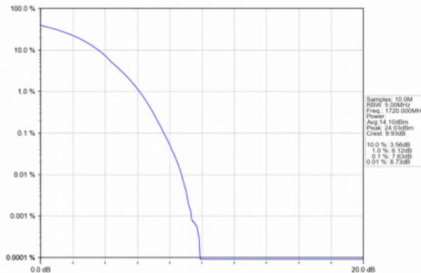
Band4_20MHz_256QAM_LCH_1720MHz_RB_100_0_NTNV
