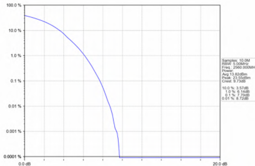
Band7_20MHz_256QAM_HCH_2560MHz_RB_100_0_NTNV
