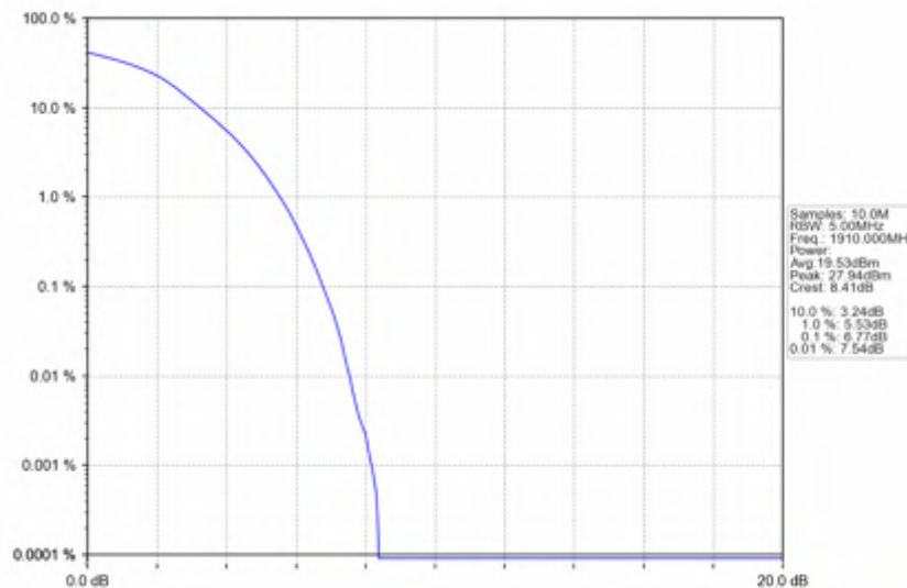
Band25_10MHz_QPSK_HCH_1910MHz_RB_50_0_NTNV
