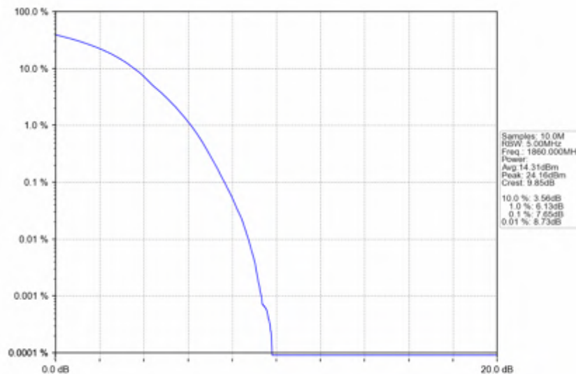
Band2_20MHz_256QAM_LCH_1860MHz_RB_100_0_NTNV
