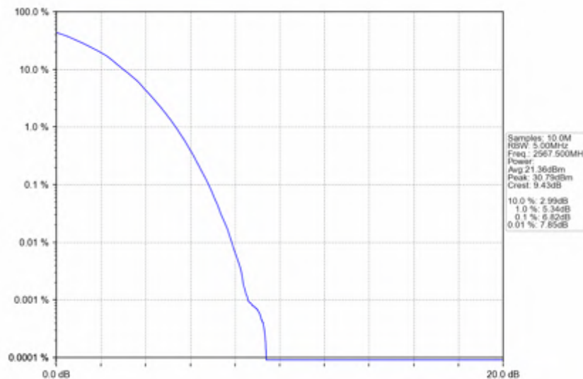
Band7_5MHz_QPSK_HCH_2567.5MHz_RB_25_0_NTNV
