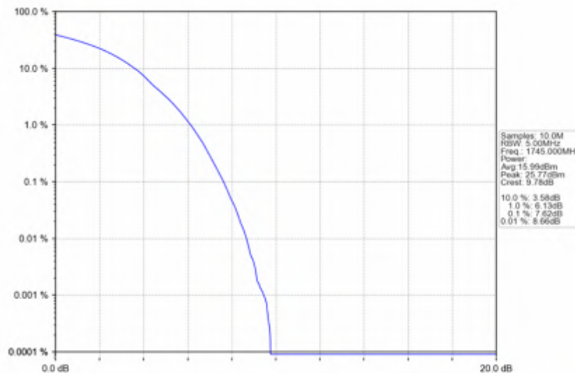
Band4_20MHz_QPSK_HCH_1745MHz_RB_100_0_NTNV
