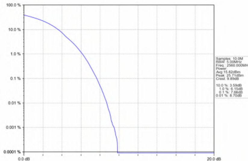
Band7_20MHz_QPSK_HCH_2560MHz_RB_100_0_NTNV
