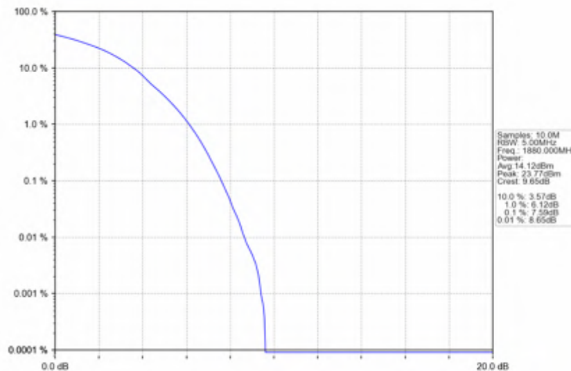
Band2_20MHz_256QAM_MCH_1880MHz_RB_100_0_NTNV
