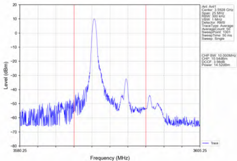
Band42c_10MHz_QPSK_HCH_3595MHz_RB_25_0_NTNV
