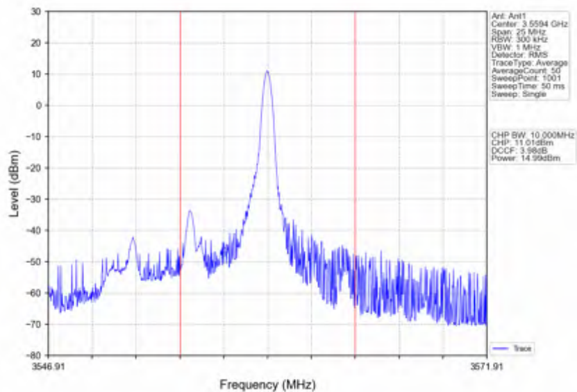
Band42c 10MHz 16QAM LCH 3555MHz RB 1 49 NTNV
