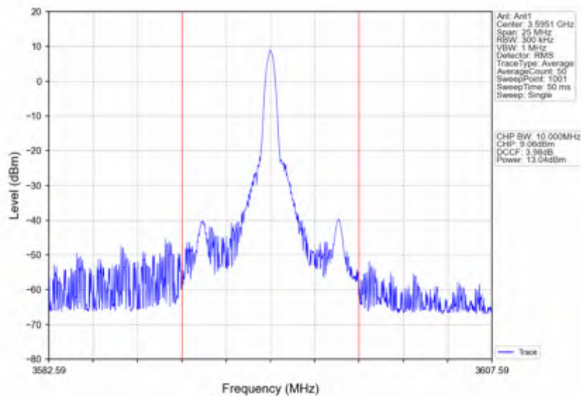
Band42c_10MHz_QPSK_HCH_3595MHz_RB_1_25_NTNV
