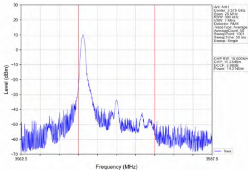
Band42c_10MHz_QPSK_MCH_3575MHz_RB_50_0_NTNV
