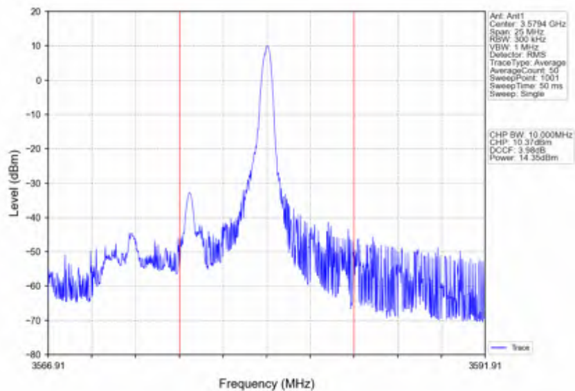
Band42c_10MHz_QPSK_MCH_3575MHz_RB_1_49_NTNV
