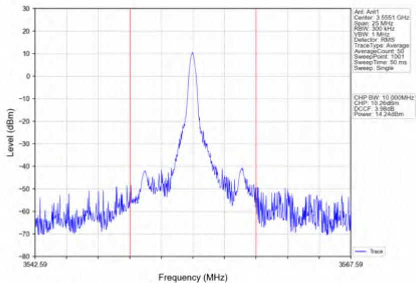
Band42c 10MHz 256QAM LCH 3555MHz RB 1 49 NTNV
