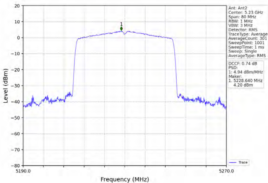
802.11ax(HEW40)_HCH_5230MHz_RU484_Left_Ant2_NTNV
