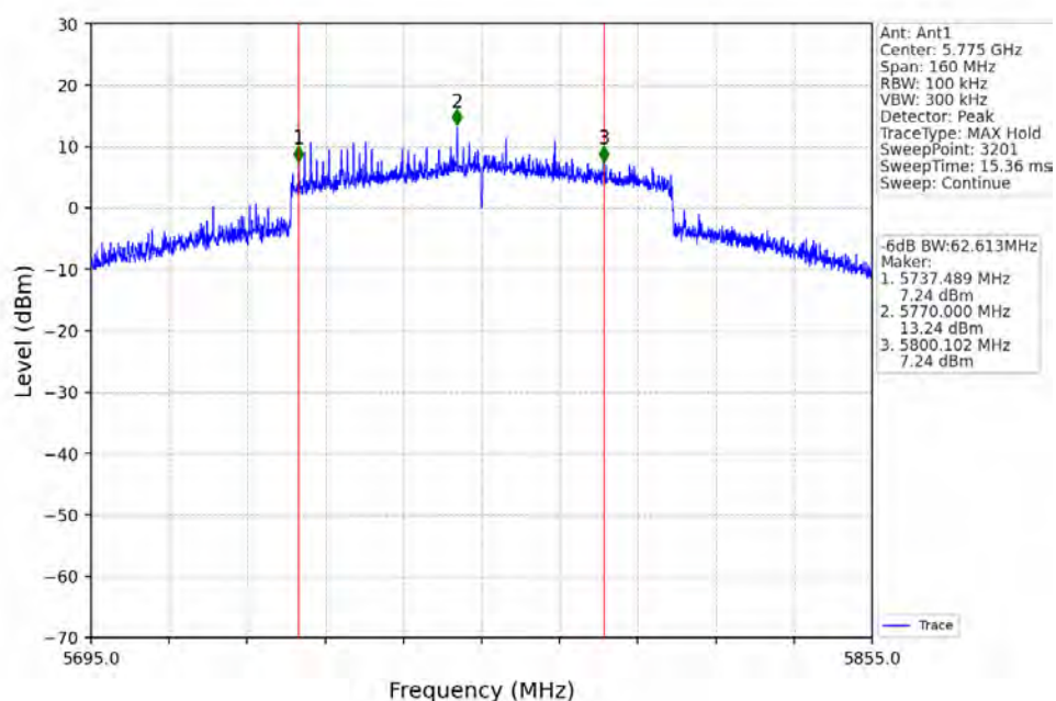
802.11ax(HEW80)_MCH_5775MHz_RU996_Left_Ant1_NTNV
