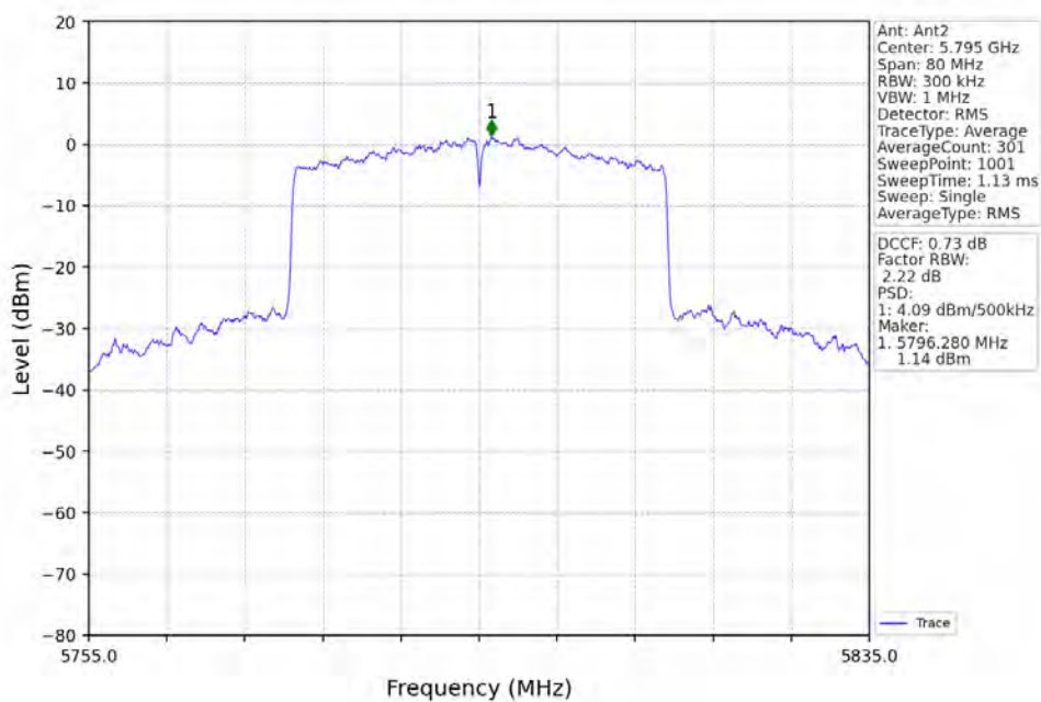
802.11ax(HEW40)_HCH_5795MHz_RU484_Left_Ant2_NTNV
