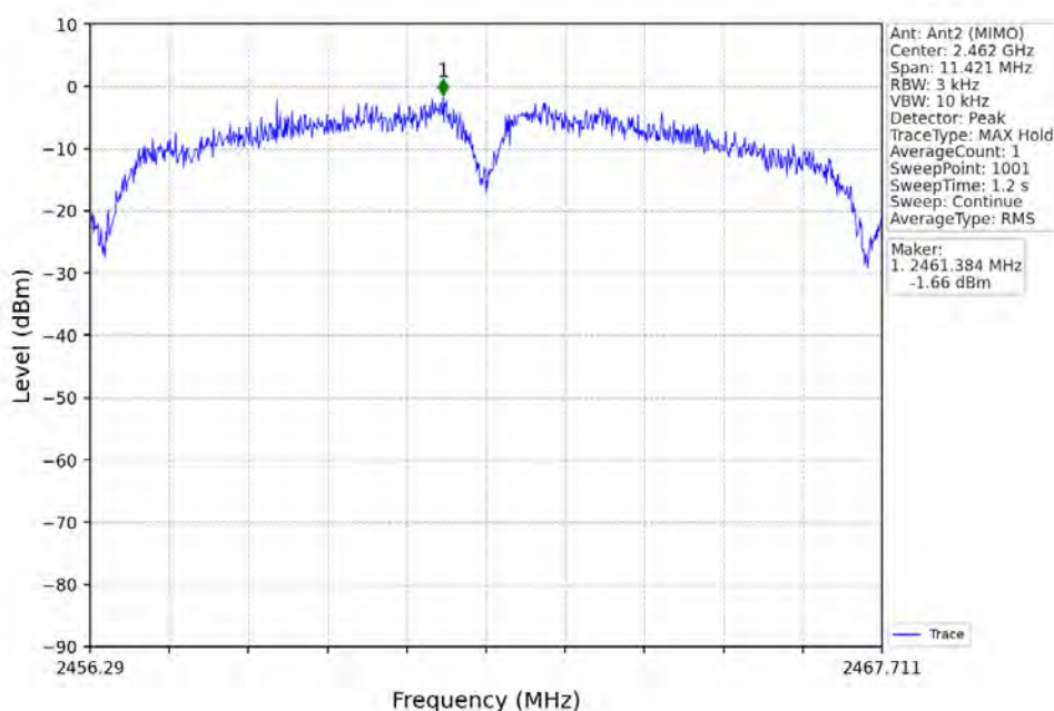
802.11b_HCH_2462MHz_Ant2 (MIMO)_NTNV
