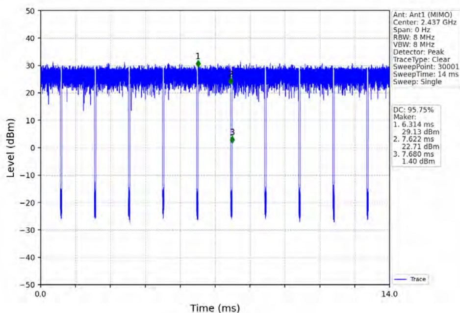
802.11n(HT20)_MCH_2437MHz_Ant1 (MIMO)_NTNV
