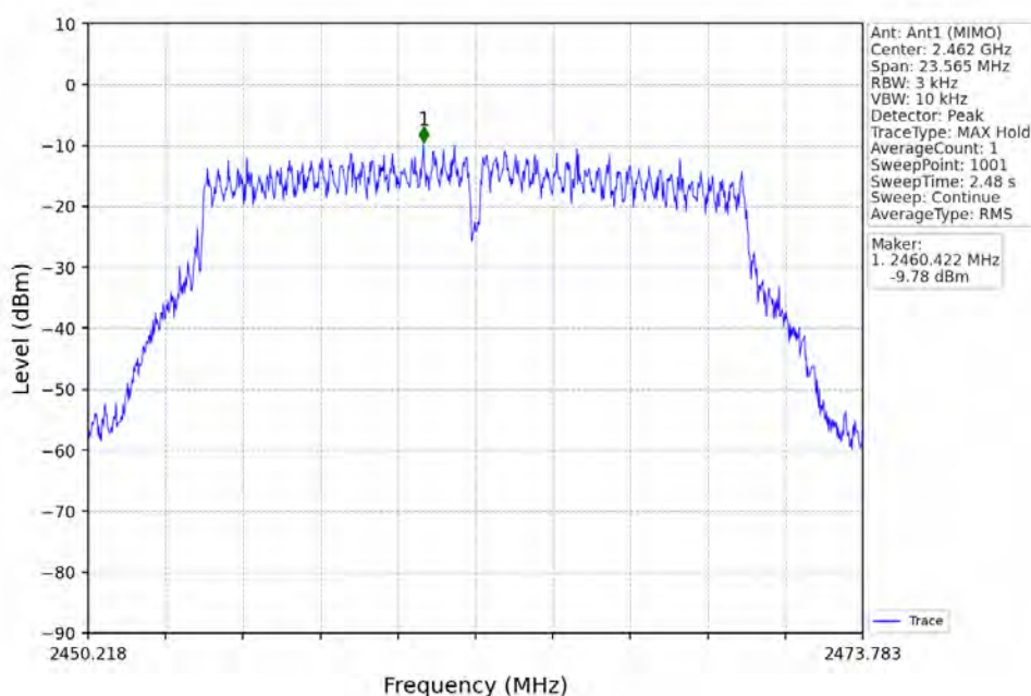
802.11g_HCH_2462MHz_Ant1 (MIMO)_NTNV
