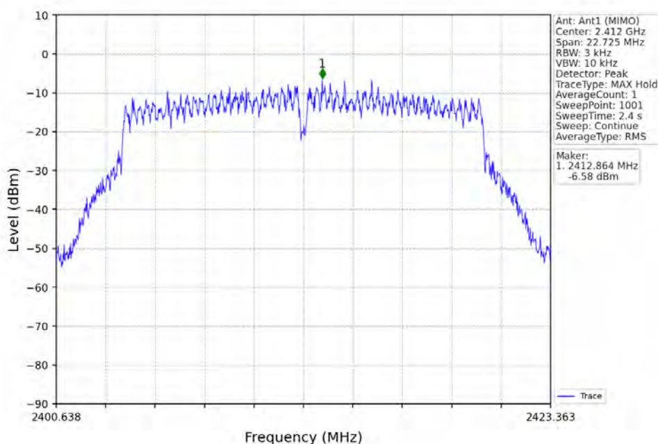
802.11g_LCH_2412MHz_Ant1 (MIMO)_NTNV
