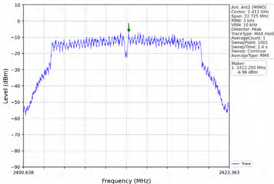
802.11g_LCH_2412MHz_MIMO_NTNV
