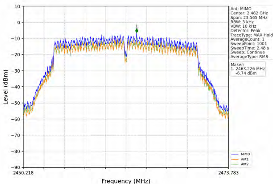
802.11g_HCH_2462MHz_MIMO_NTNV
