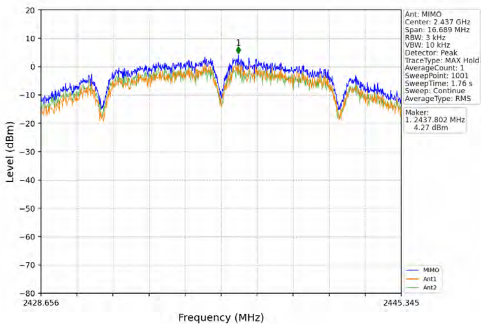
802.11b_MCH_2437MHz_MIMO_NTNV
