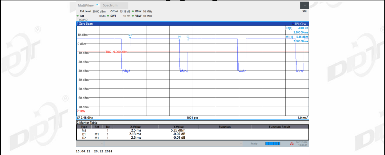
BLE_1M_Right side_2480
