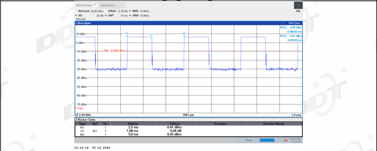
BLE_2M_Right side_2440
