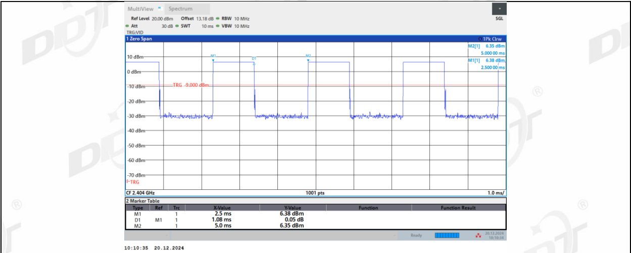
BLE_2M_Right side_2404
