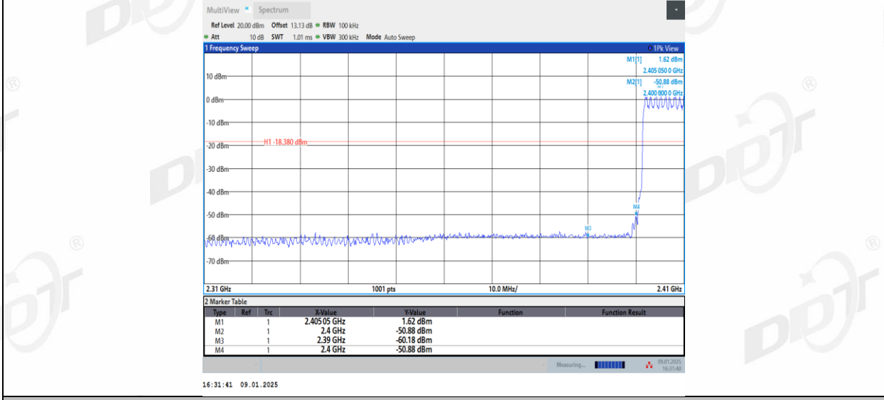
3DH5_Right side_Low_Hop_2402
