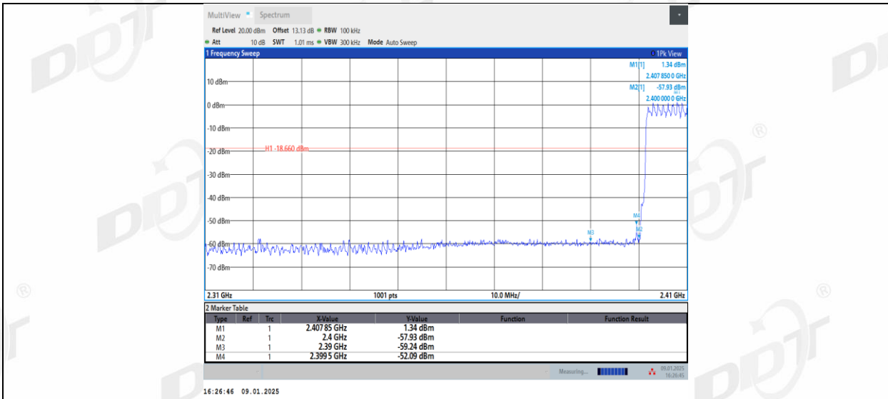
2DH5_Right side_Low_Hop_2402
