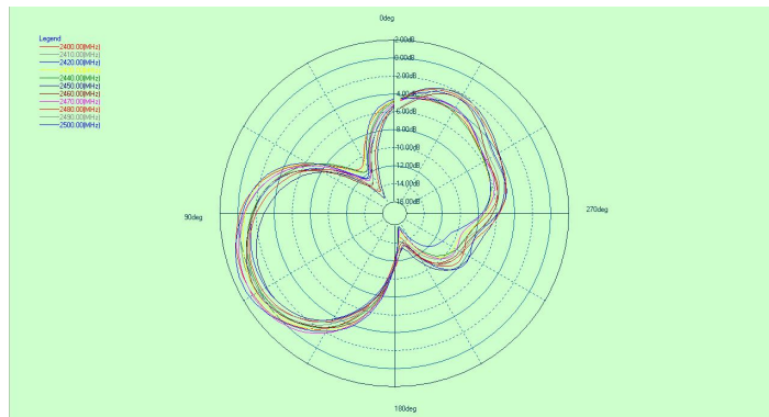
RX0: \Theta=90^\circ
