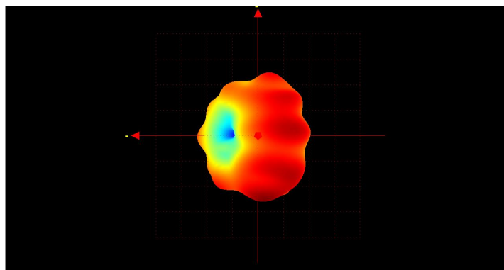
RX0 3D:XOZ
